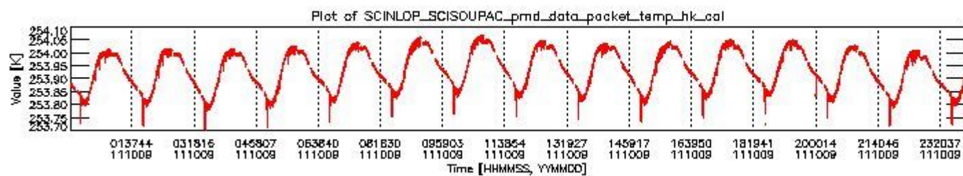
sciamachy_daily_report_level0_KSPT_L0_4504_N_20111009_3.PNG
