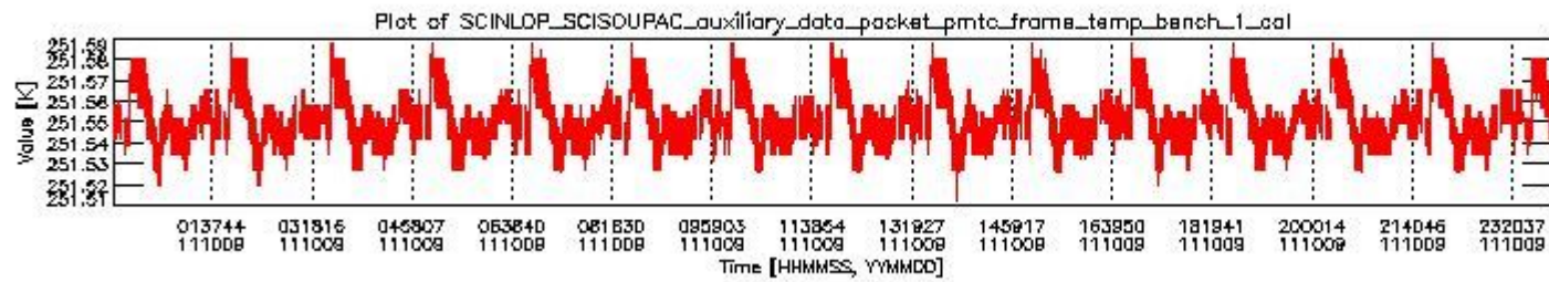
sciamachy_daily_report_level0_KSPT_L0_4504_N_20111009_0.PNG
