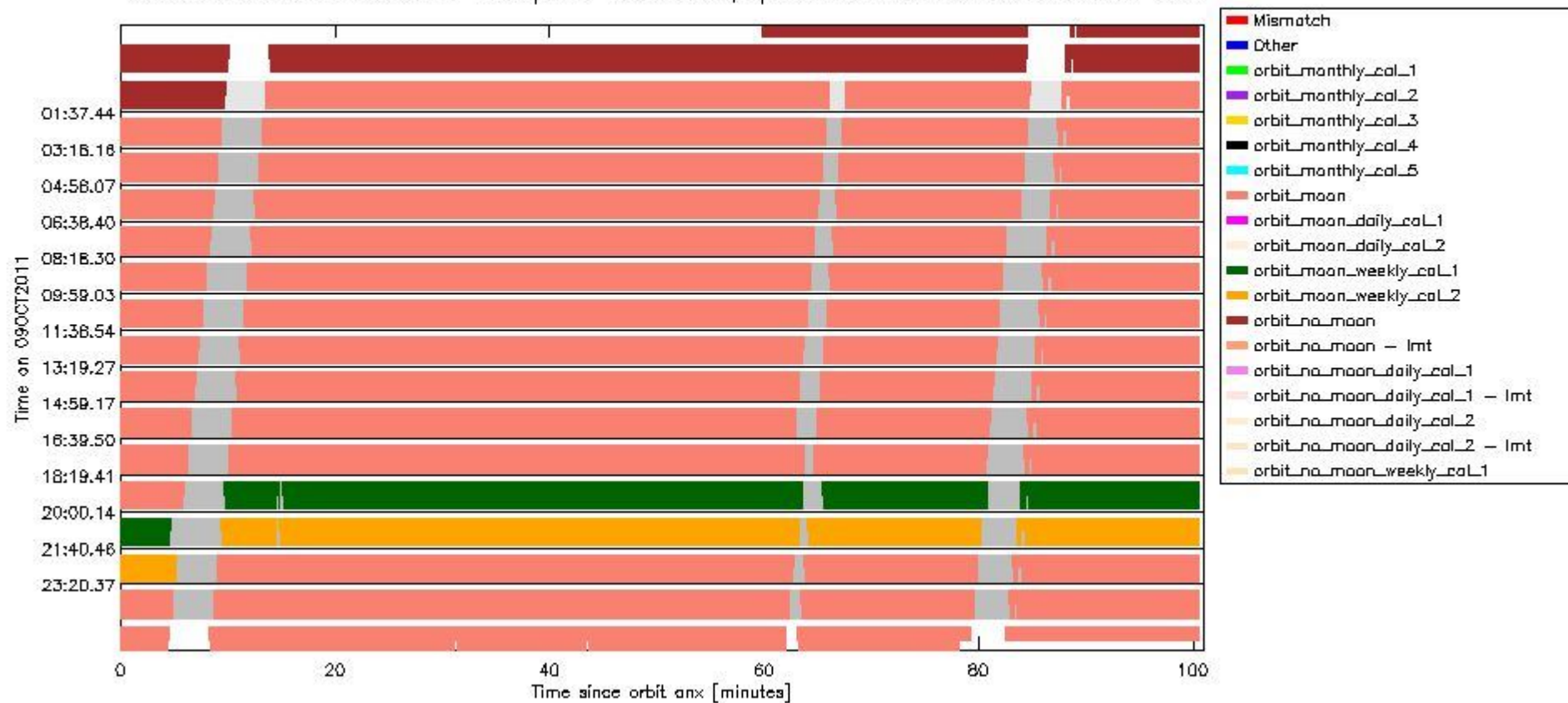
sciamachy_daily_report_level0_KSPT_L0_4504_N_20111009_6.PNG
