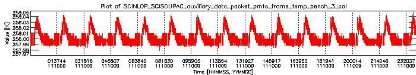
sciamachy_daily_report_level0_KSPT_L0_4504_N_20111009_2.PNG
