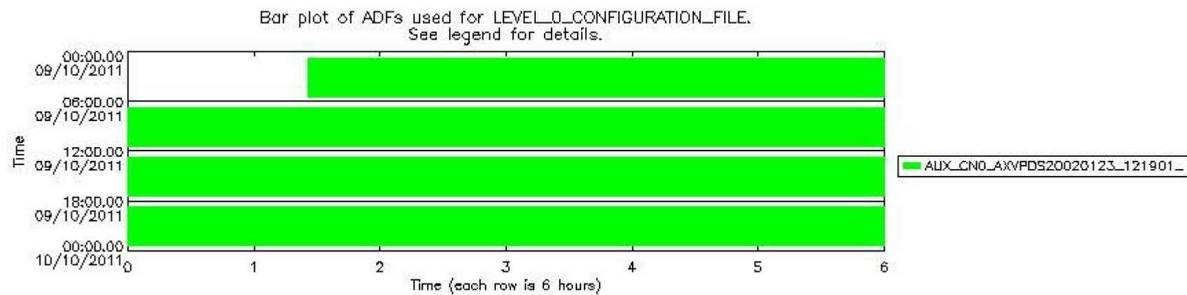
sciamachy_daily_report_level0_KSPT_L0_4504_N_20111009_7.PNG
