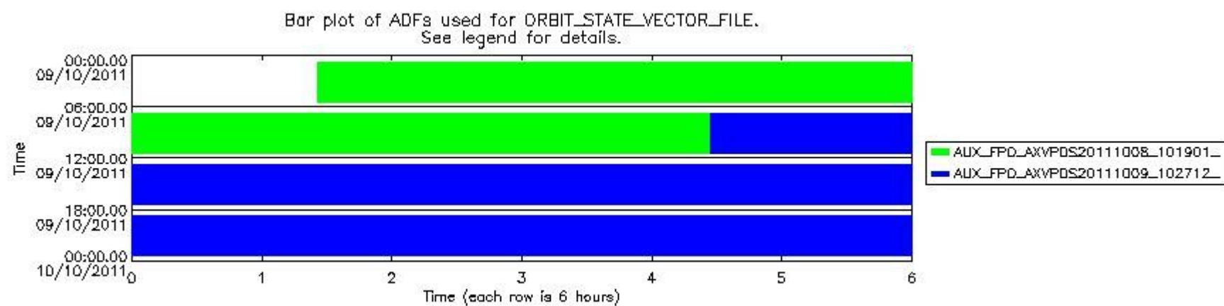
sciamachy_daily_report_level0_KSPT_L0_4504_N_20111009_8.PNG
