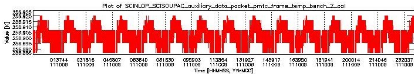
sciamachy_daily_report_level0_KSPT_L0_4504_N_20111009_1.PNG
