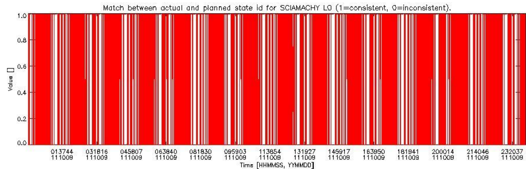
sciamachy_daily_report_level0_KSPT_L0_4504_N_20111009_5.PNG
