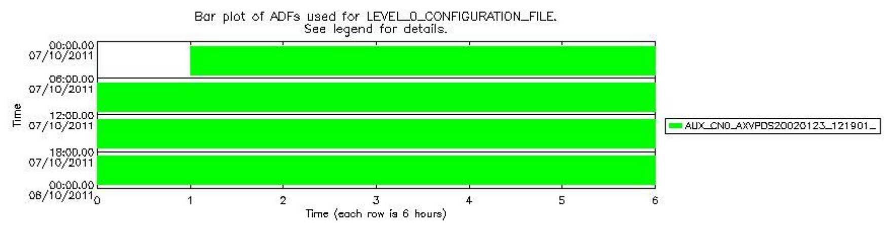
sciamachy_daily_report_level0_KSPT_L0_4504_N_20111007_7.PNG
