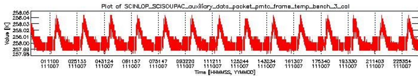
sciamachy_daily_report_level0_KSPT_L0_4504_N_20111007_2.PNG
