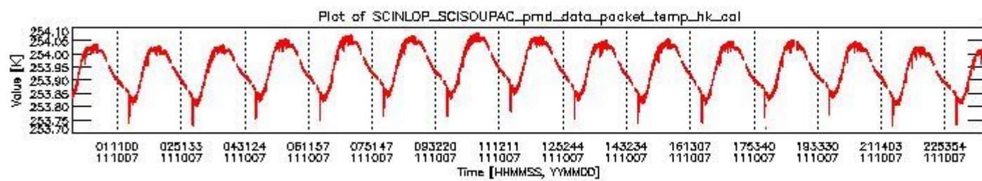
sciamachy_daily_report_level0_KSPT_L0_4504_N_20111007_3.PNG
