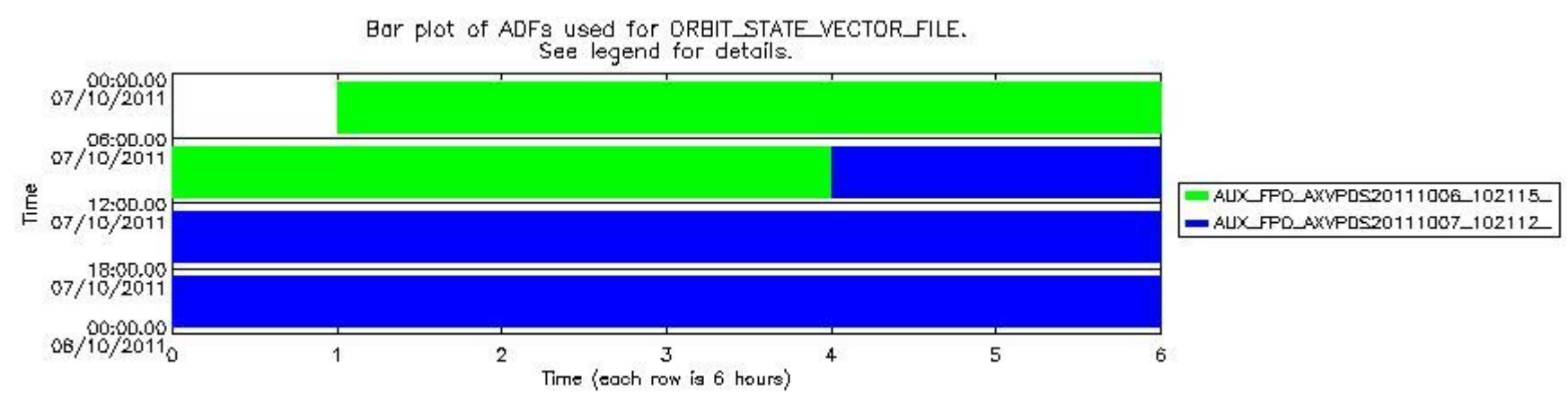
sciamachy_daily_report_level0_KSPT_L0_4504_N_20111007_8.PNG
