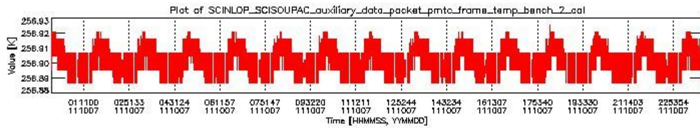
sciamachy_daily_report_level0_KSPT_L0_4504_N_20111007_1.PNG
