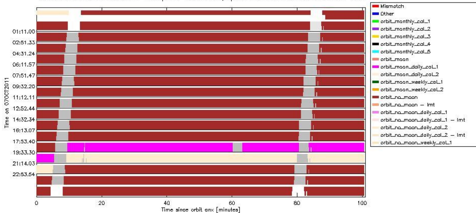
sciamachy_daily_report_level0_KSPT_L0_4504_N_20111007_6.PNG
