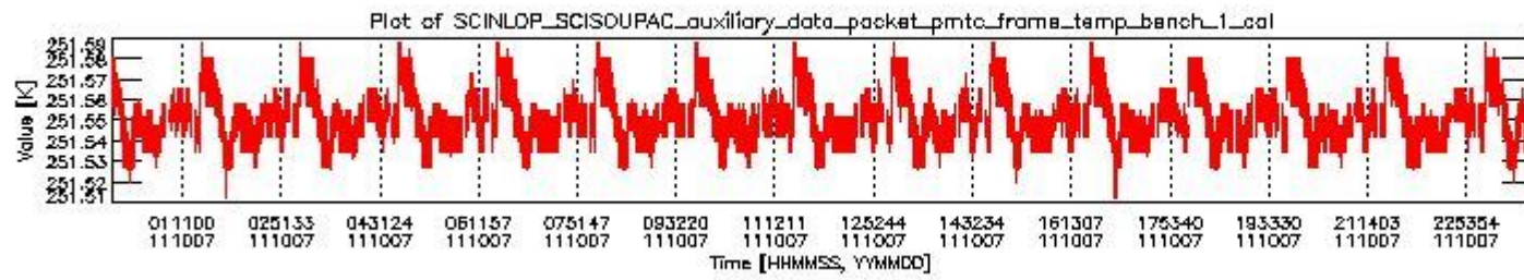
sciamachy_daily_report_level0_KSPT_L0_4504_N_20111007_0.PNG
