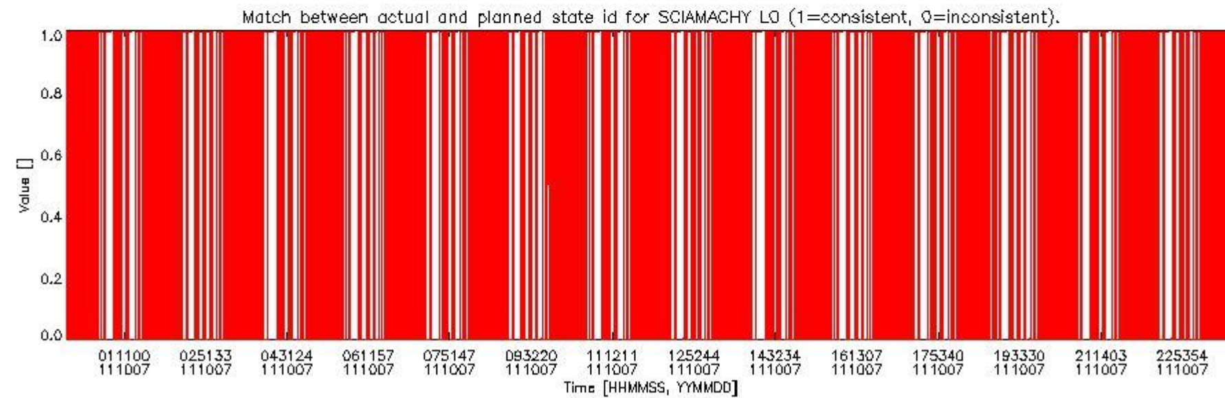
sciamachy_daily_report_level0_KSPT_L0_4504_N_20111007_5.PNG
