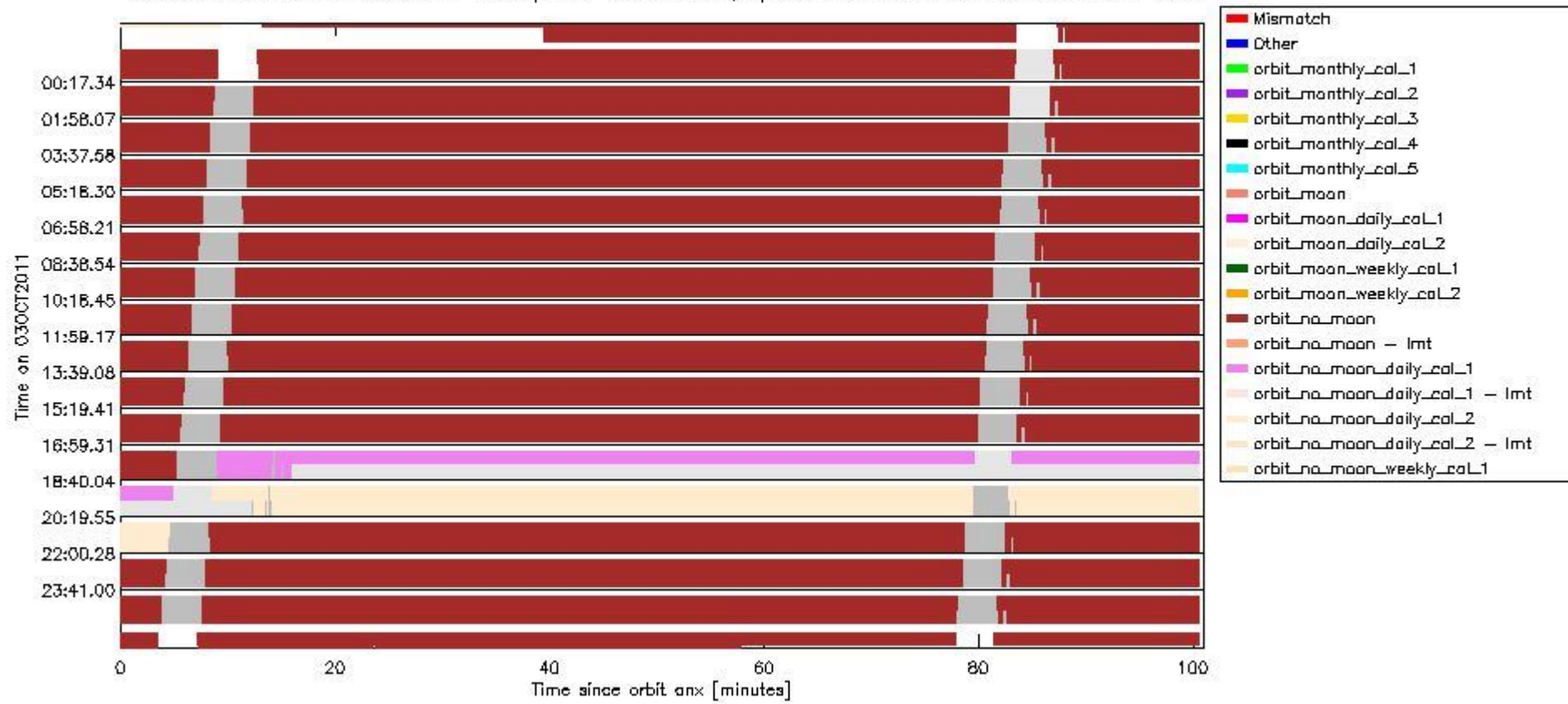
sciamachy_daily_report_level0_KSPT_L0_4504_N_20111003_6.PNG
