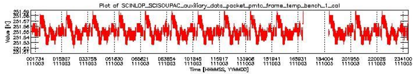
sciamachy_daily_report_level0_KSPT_L0_4504_N_20111003_0.PNG
