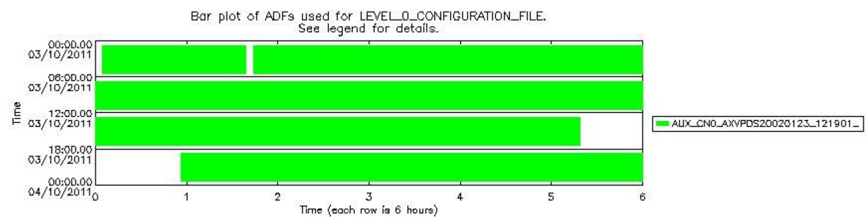
sciamachy_daily_report_level0_KSPT_L0_4504_N_20111003_7.PNG
