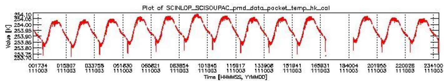
sciamachy_daily_report_level0_KSPT_L0_4504_N_20111003_3.PNG
