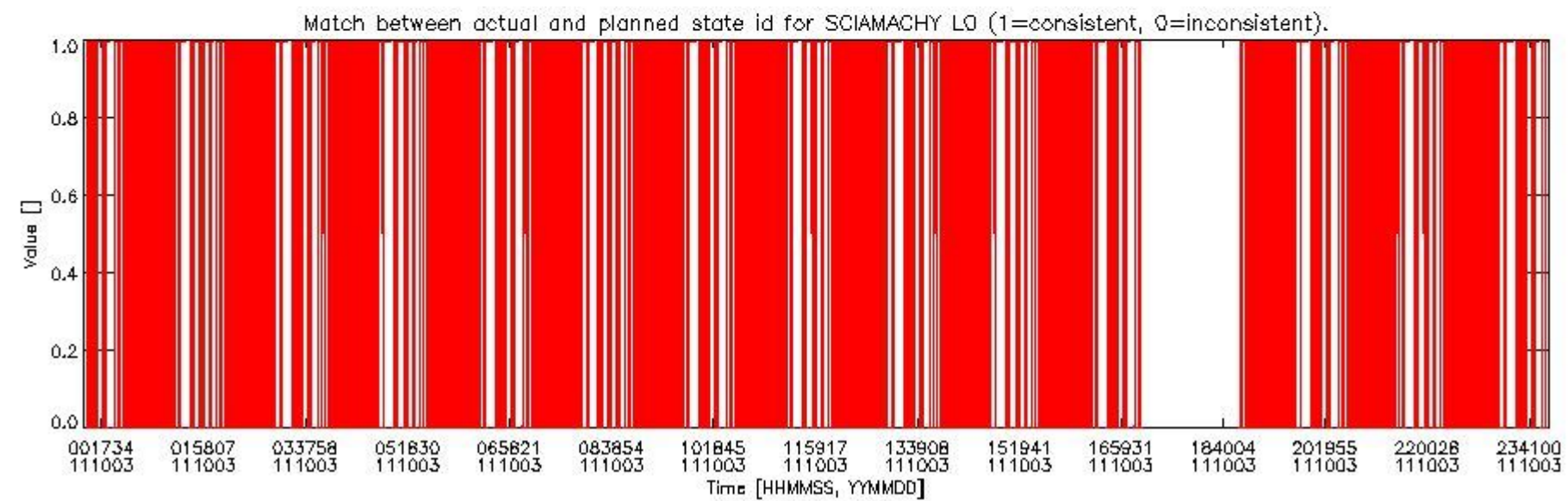
sciamachy_daily_report_level0_KSPT_L0_4504_N_20111003_5.PNG
