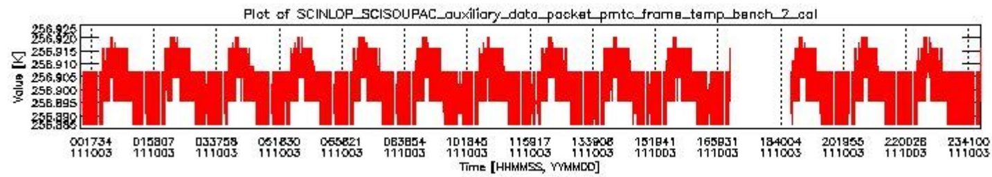
sciamachy_daily_report_level0_KSPT_L0_4504_N_20111003_1.PNG
