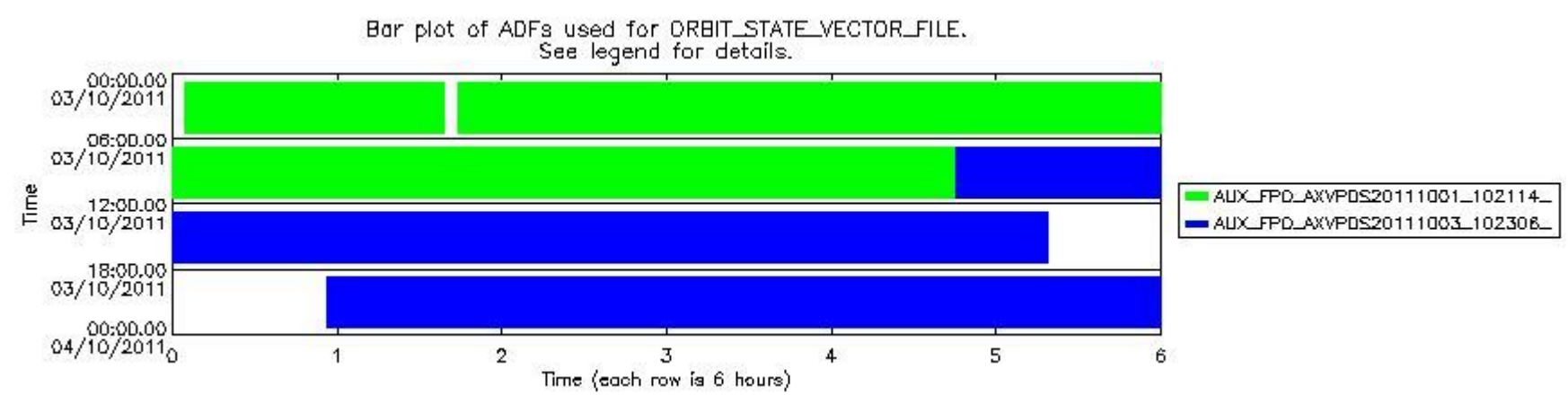
sciamachy_daily_report_level0_KSPT_L0_4504_N_20111003_8.PNG
