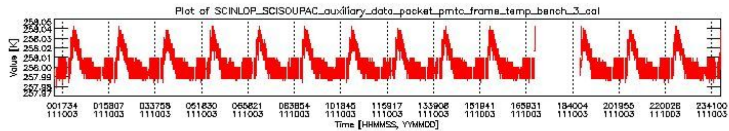
sciamachy_daily_report_level0_KSPT_L0_4504_N_20111003_2.PNG
