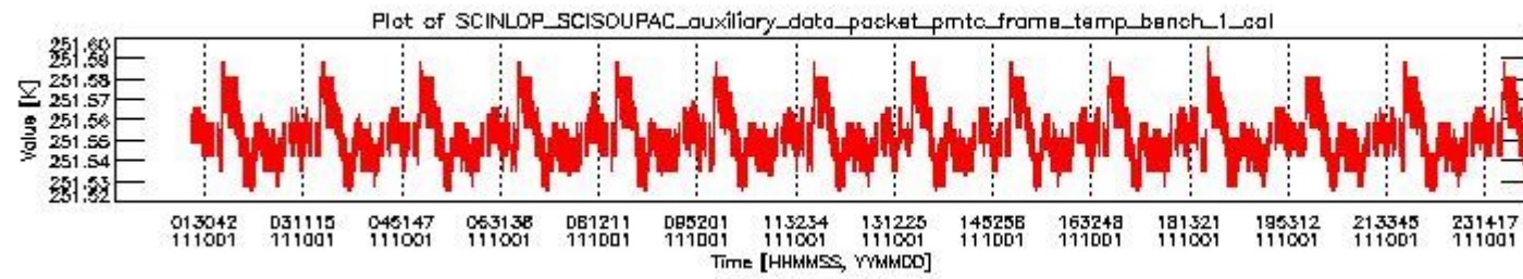
sciamachy_daily_report_level0_KSPT_L0_4504_N_20111001_0.PNG
