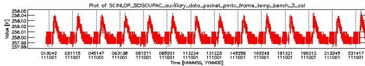
sciamachy_daily_report_level0_KSPT_L0_4504_N_20111001_2.PNG
