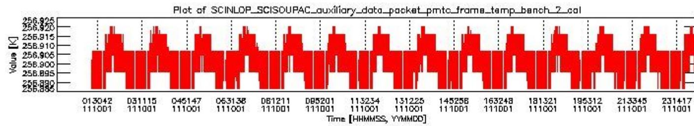
sciamachy_daily_report_level0_KSPT_L0_4504_N_20111001_1.PNG
