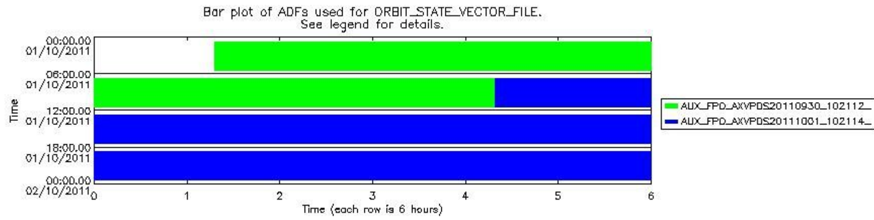
sciamachy_daily_report_level0_KSPT_L0_4504_N_20111001_8.PNG
