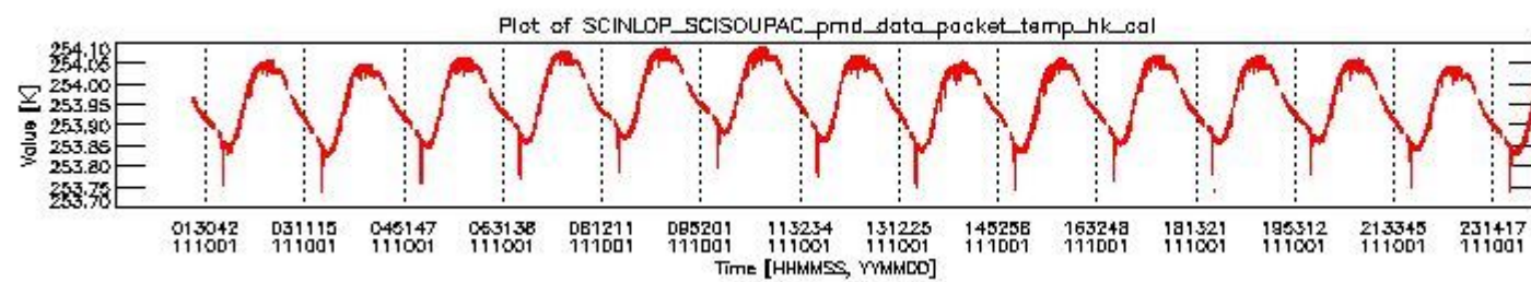
sciamachy_daily_report_level0_KSPT_L0_4504_N_20111001_3.PNG
