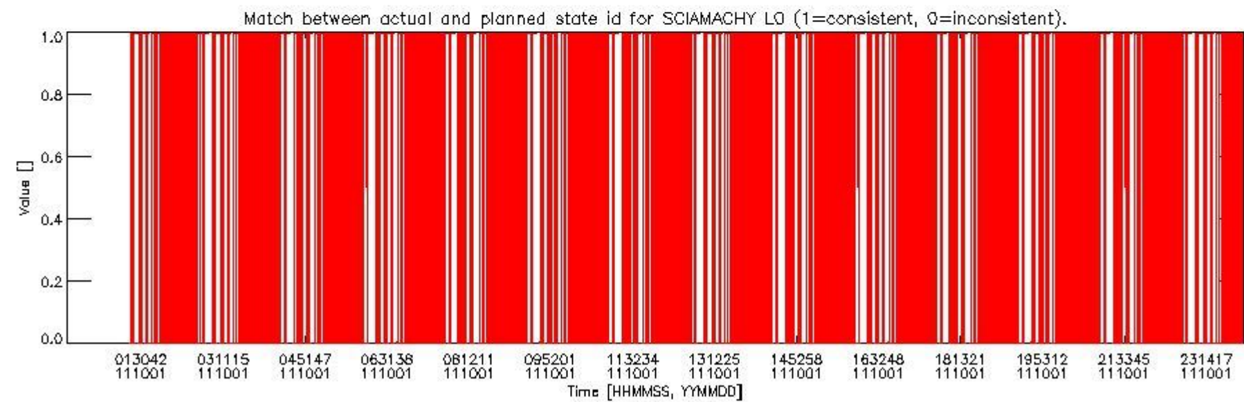
sciamachy_daily_report_level0_KSPT_L0_4504_N_2011001_5.PNG
