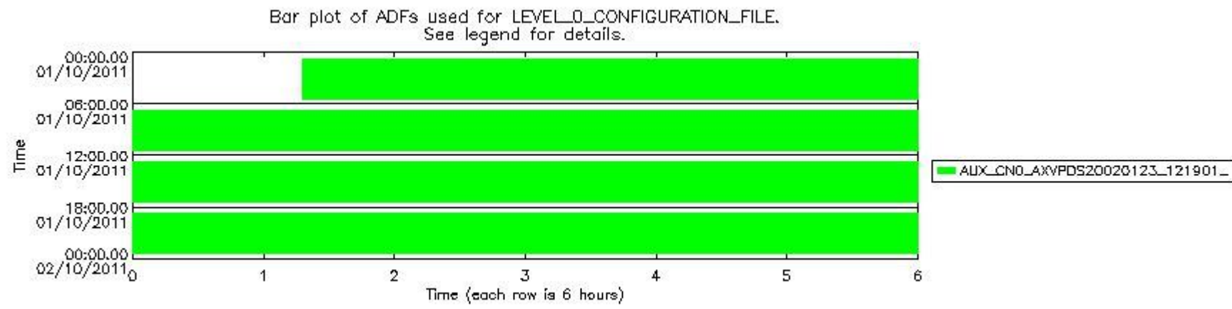
sciamachy_daily_report_level0_KSPT_L0_4504_N_20111001_7.PNG
