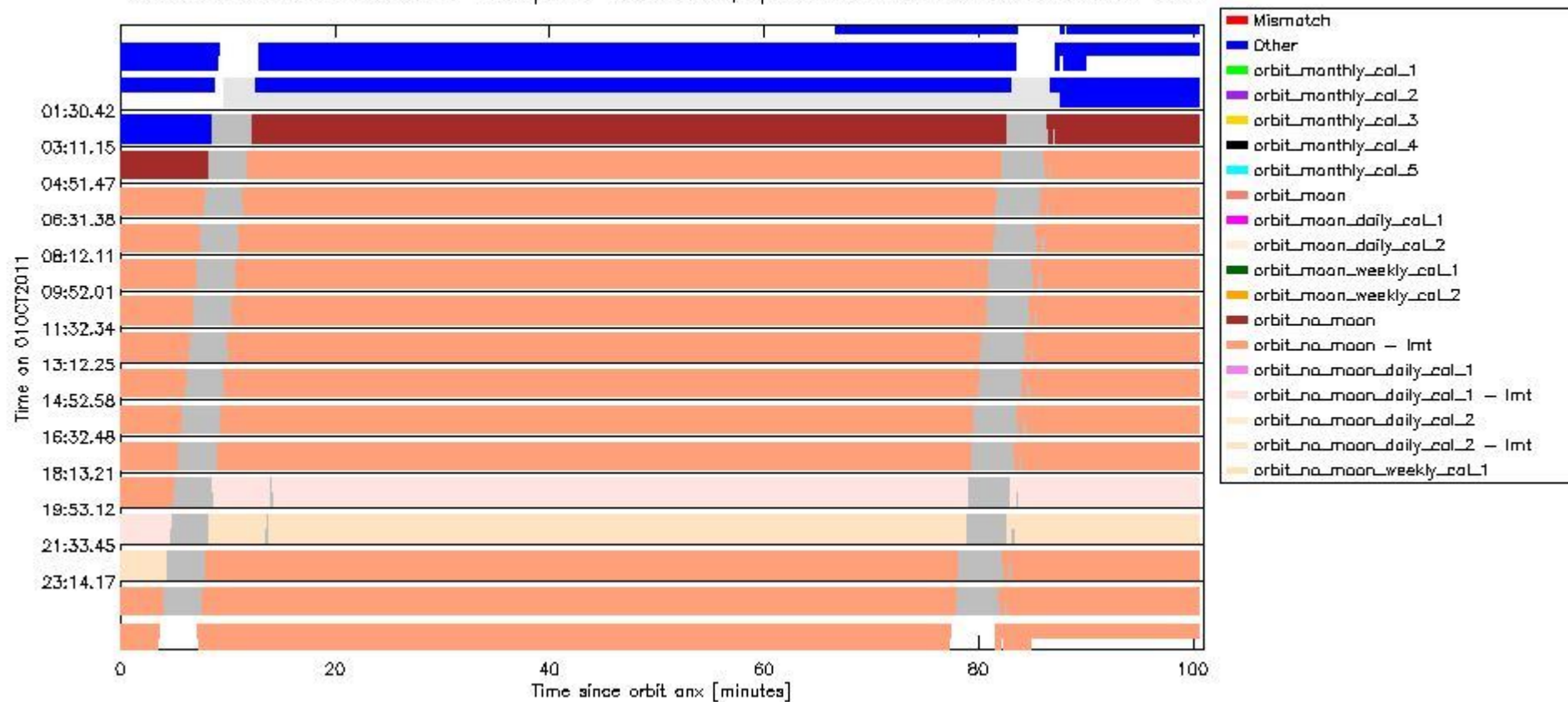
sciamachy_daily_report_level0_KSPT_L0_4504_N_20111001_6.PNG
