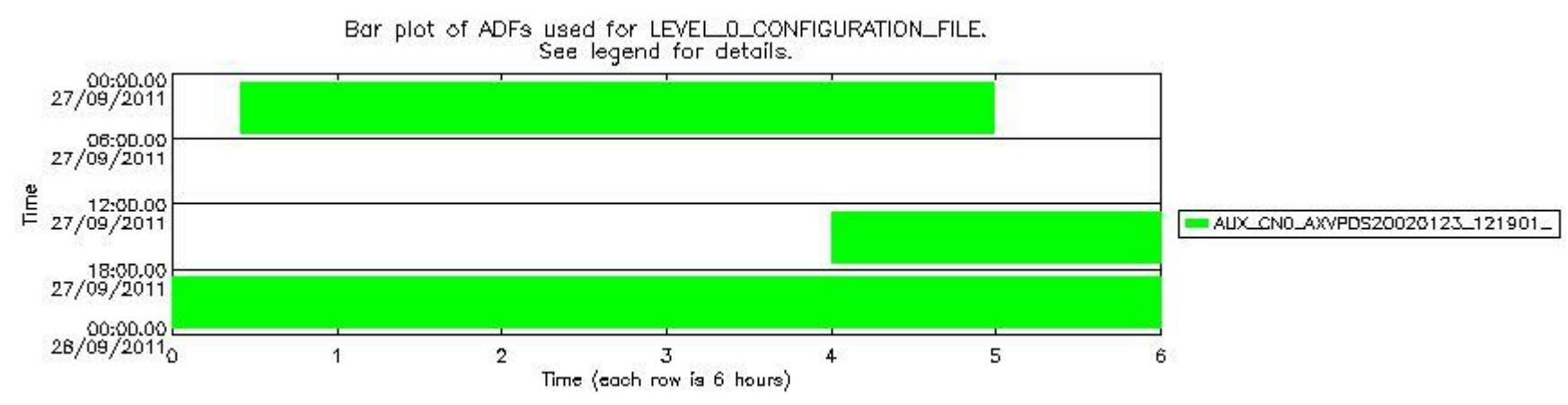
sciamachy_daily_report_level0_KSPT_L0_4504_N_20110927_7.PNG
