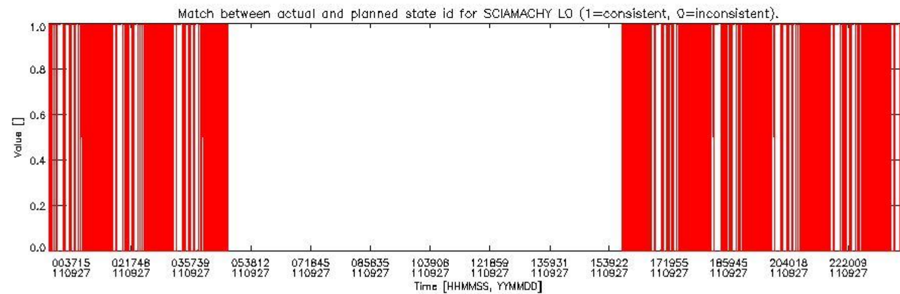
sciamachy_daily_report_level0_KSPT_L0_4504_N_20110927_5.PNG
