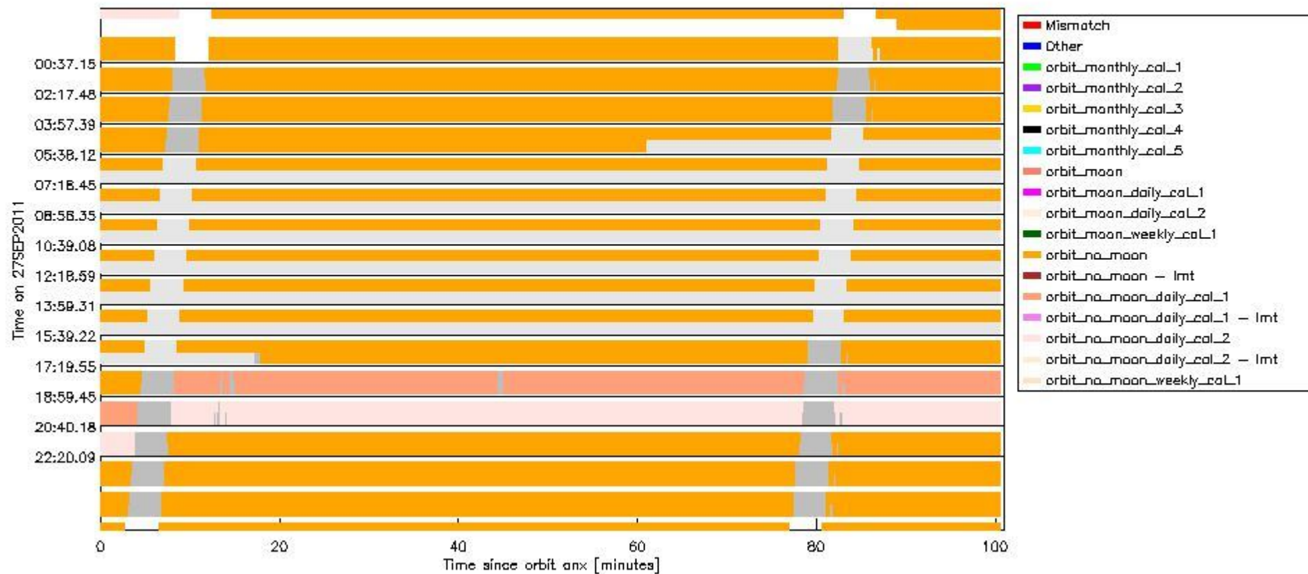
sciamachy_daily_report_level0_KSPT_L0_4504_N_20110927_6.PNG
