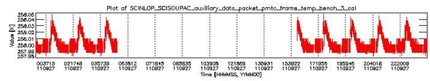
sciamachy_daily_report_level0_KSPT_L0_4504_N_20110927_2.PNG
