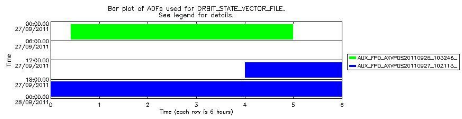
sciamachy_daily_report_level0_KSPT_L0_4504_N_20110927_8.PNG
