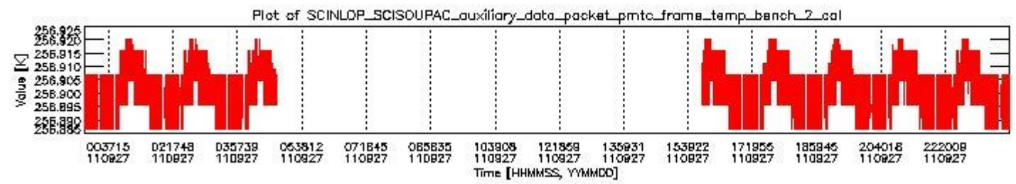
sciamachy_daily_report_level0_KSPT_L0_4504_N_20110927_1.PNG
