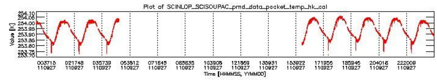
sciamachy_daily_report_level0_KSPT_L0_4504_N_20110927_3.PNG
