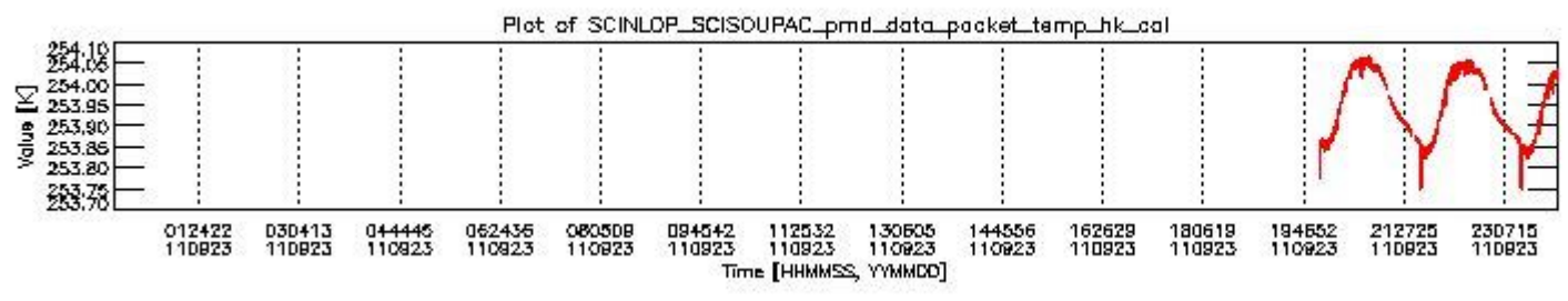
sciamachy_daily_report_level0_KSPT_L0_4504_N_20110923_3.PNG
