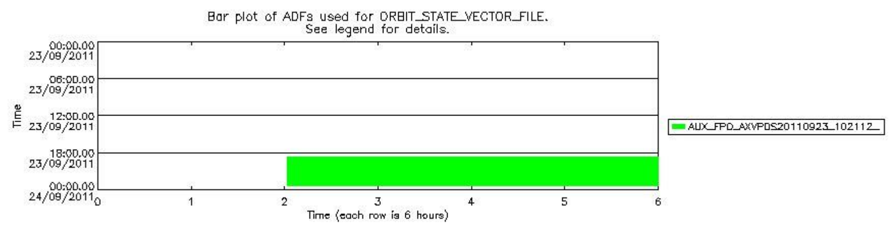
sciamachy_daily_report_level0_KSPT_L0_4504_N_20110923_8.PNG
