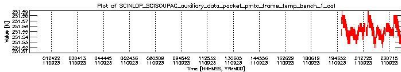
sciamachy_daily_report_level0_KSPT_L0_4504_N_20110923_0.PNG
