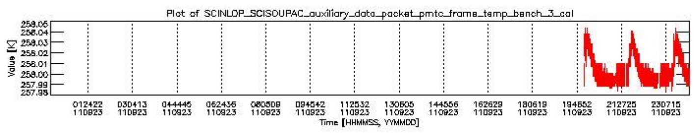
sciamachy_daily_report_level0_KSPT_L0_4504_N_20110923_2.PNG
