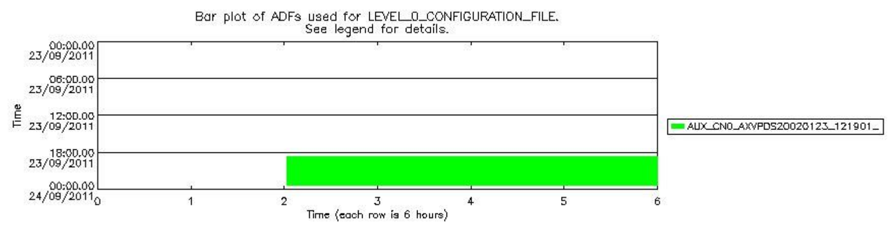
sciamachy_daily_report_level0_KSPT_L0_4504_N_20110923_7.PNG
