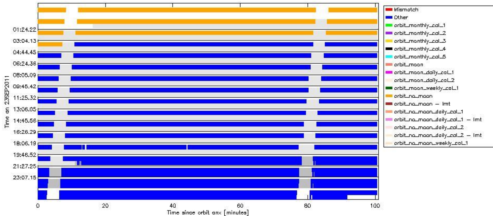
sciamachy_daily_report_level0_KSPT_L0_4504_N_20110923_6.PNG
