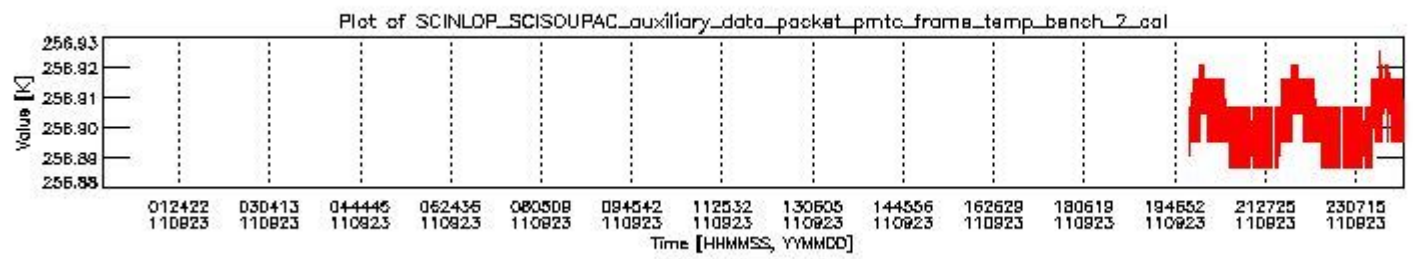
sciamachy_daily_report_level0_KSPT_L0_4504_N_20110923_1.PNG
