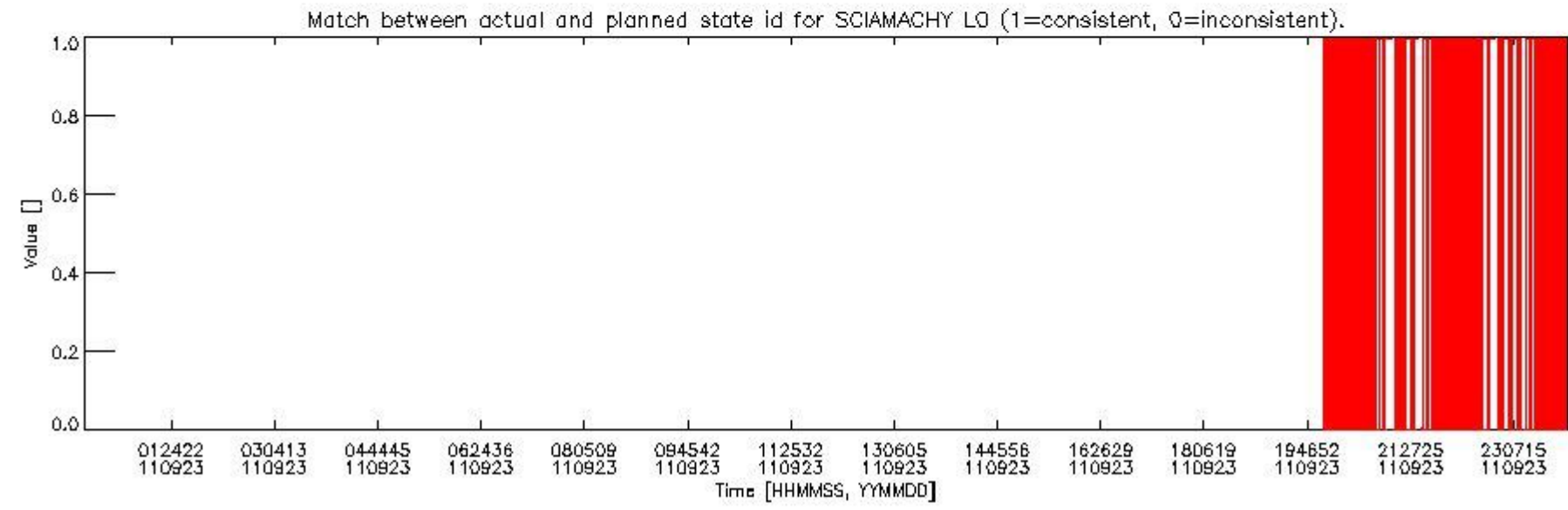
sciamachy_daily_report_level0_KSPT_L0_4504_N_20110923_5.PNG
