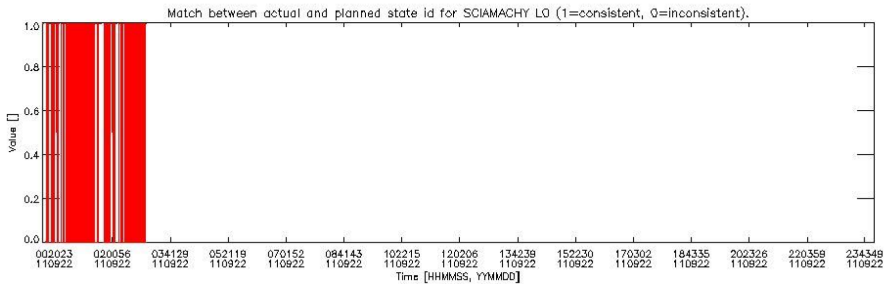
sciamachy_daily_report_level0_KSPT_L0_4504_N_20110922_5.PNG
