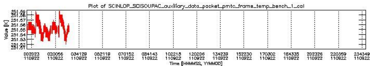
sciamachy_daily_report_level0_KSPT_L0_4504_N_20110922_0.PNG
