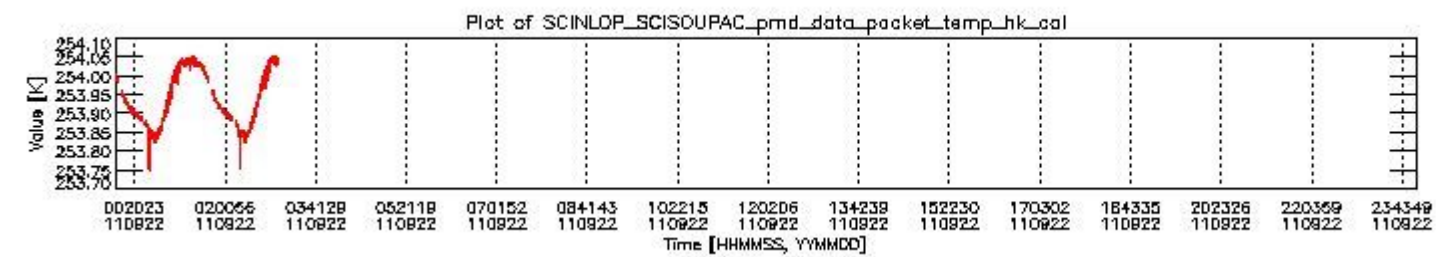
sciamachy_daily_report_level0_KSPT_L0_4504_N_20110922_3.PNG
