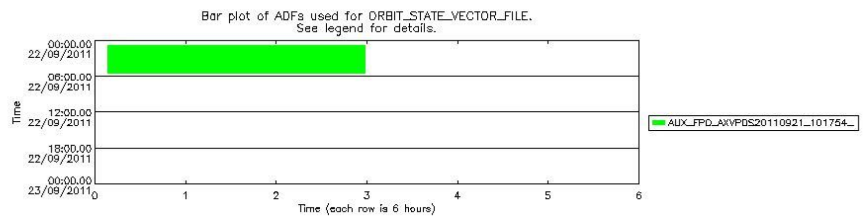
sciamachy_daily_report_level0_KSPT_L0_4504_N_20110922_8.PNG
