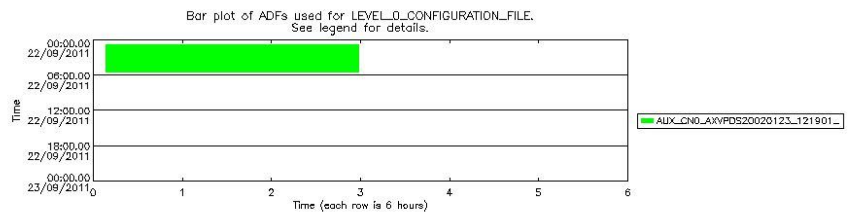
sciamachy_daily_report_level0_KSPT_L0_4504_N_20110922_7.PNG
