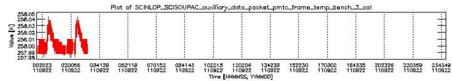
sciamachy_daily_report_level0_KSPT_L0_4504_N_20110922_2.PNG
