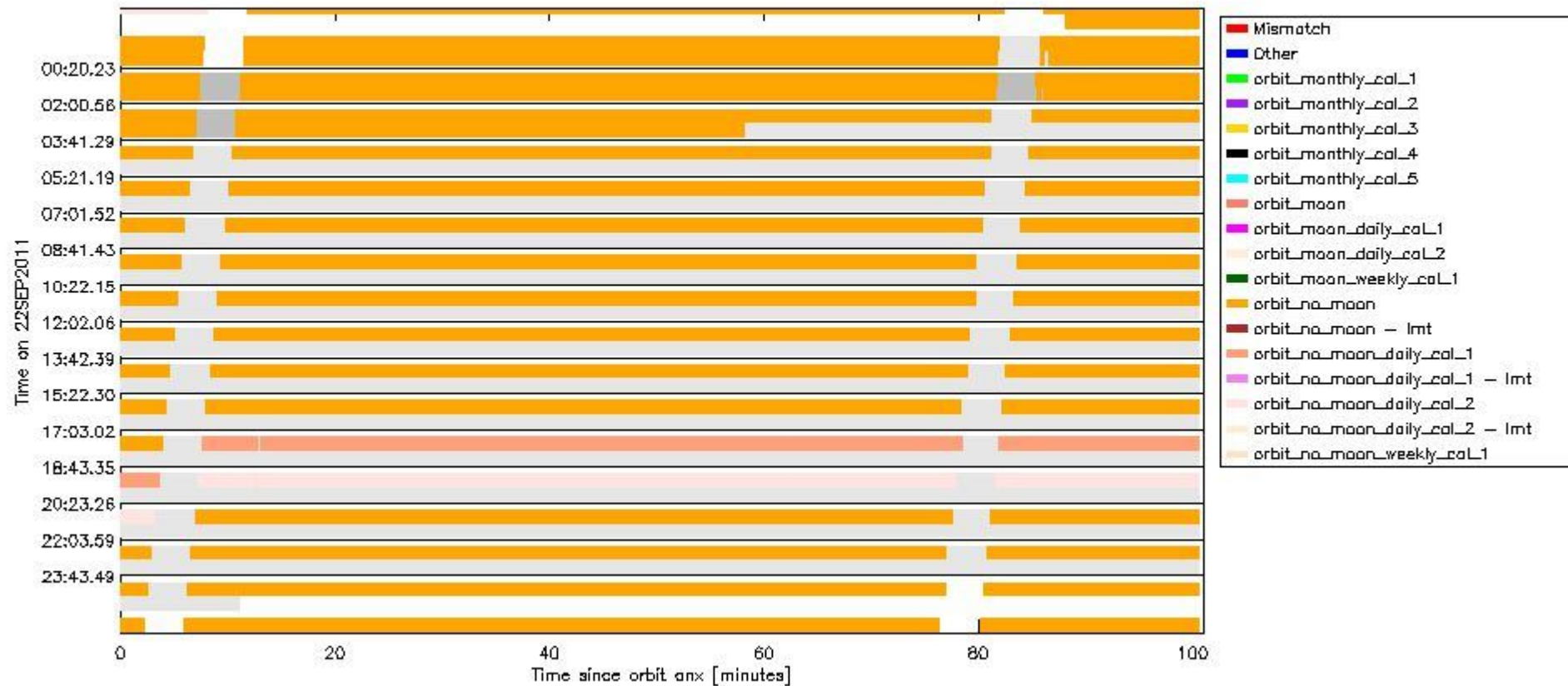
sciamachy_daily_report_level0_KSPT_L0_4504_N_20110922_6.PNG
