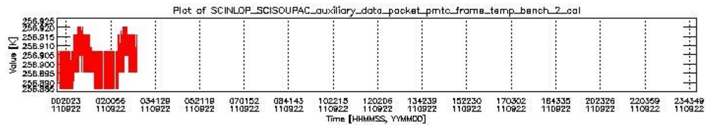
sciamachy_daily_report_level0_KSPT_L0_4504_N_20110922_1.PNG
