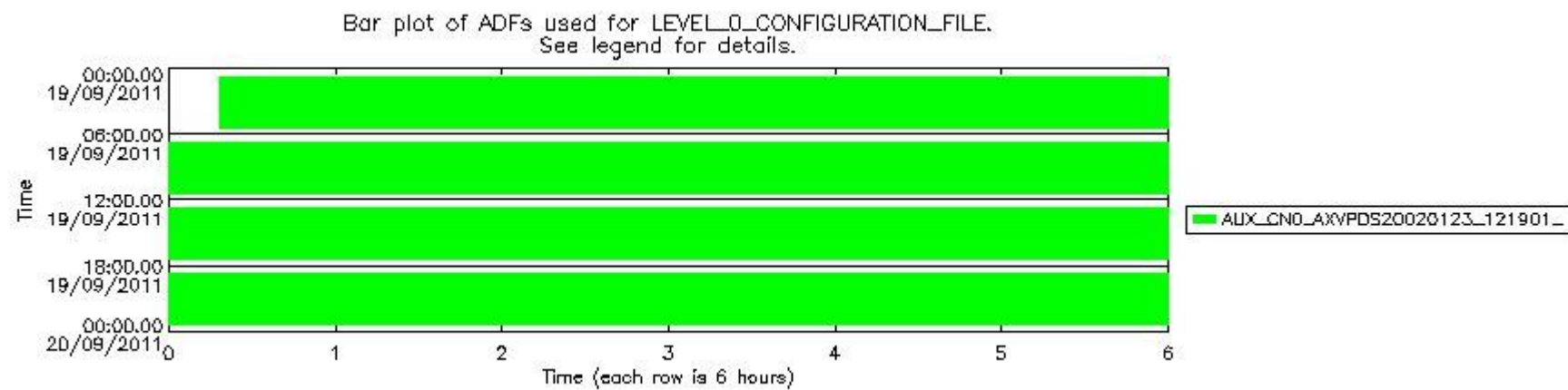
sciamachy_daily_report_level0_KSPT_L0_4504_N_20110919_7.PNG
