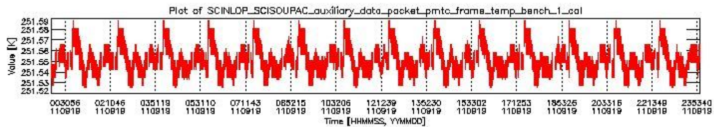
sciamachy_daily_report_level0_KSPT_L0_4504_N_20110919_0.PNG
