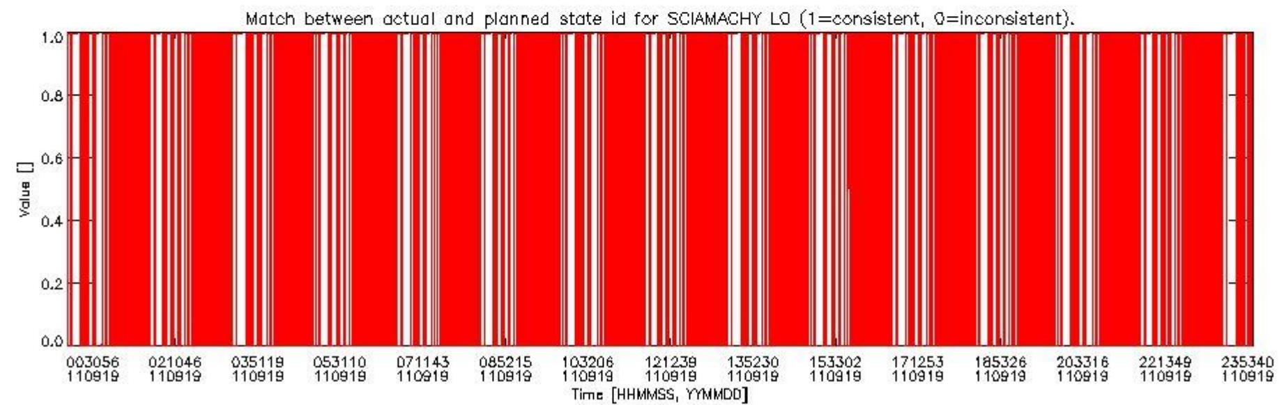
sciamachy_daily_report_level0_KSPT_L0_4504_N_20110919_5.PNG
