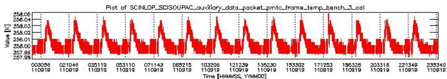
sciamachy_daily_report_level0_KSPT_L0_4504_N_20110919_2.PNG
