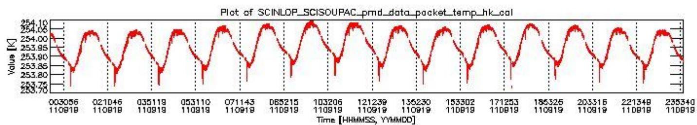
sciamachy_daily_report_level0_KSPT_L0_4504_N_20110919_3.PNG
