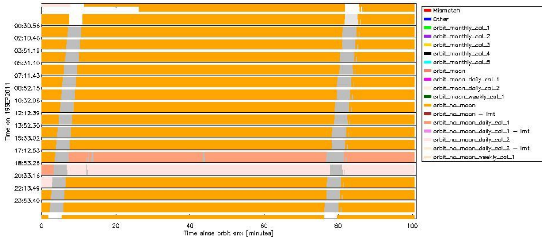
sciamachy_daily_report_level0_KSPT_L0_4504_N_20110919_6.PNG
