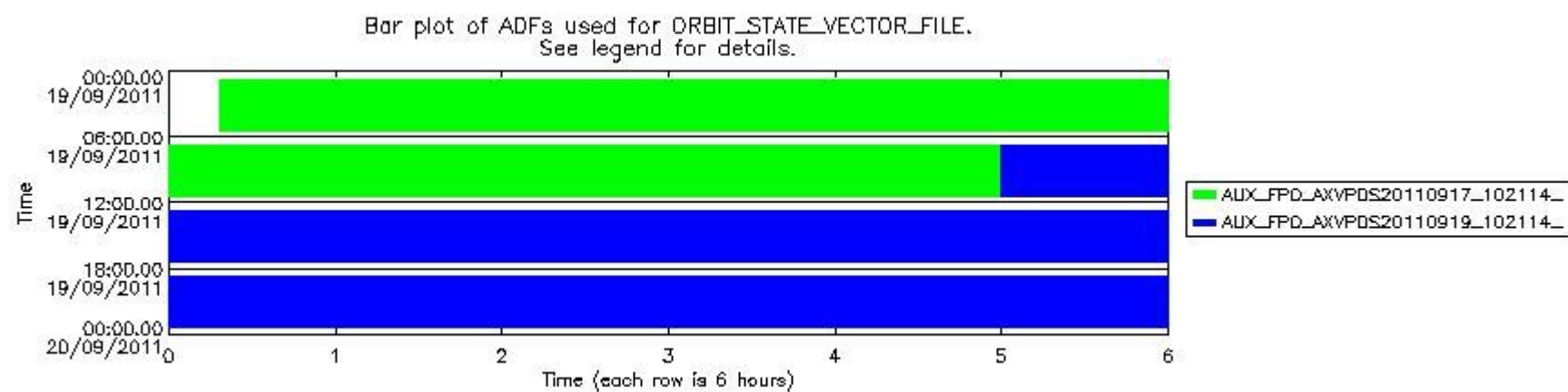
sciamachy_daily_report_level0_KSPT_L0_4504_N_20110919_8.PNG
