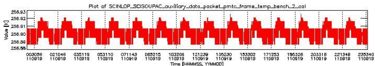
sciamachy_daily_report_level0_KSPT_L0_4504_N_20110919_1.PNG
