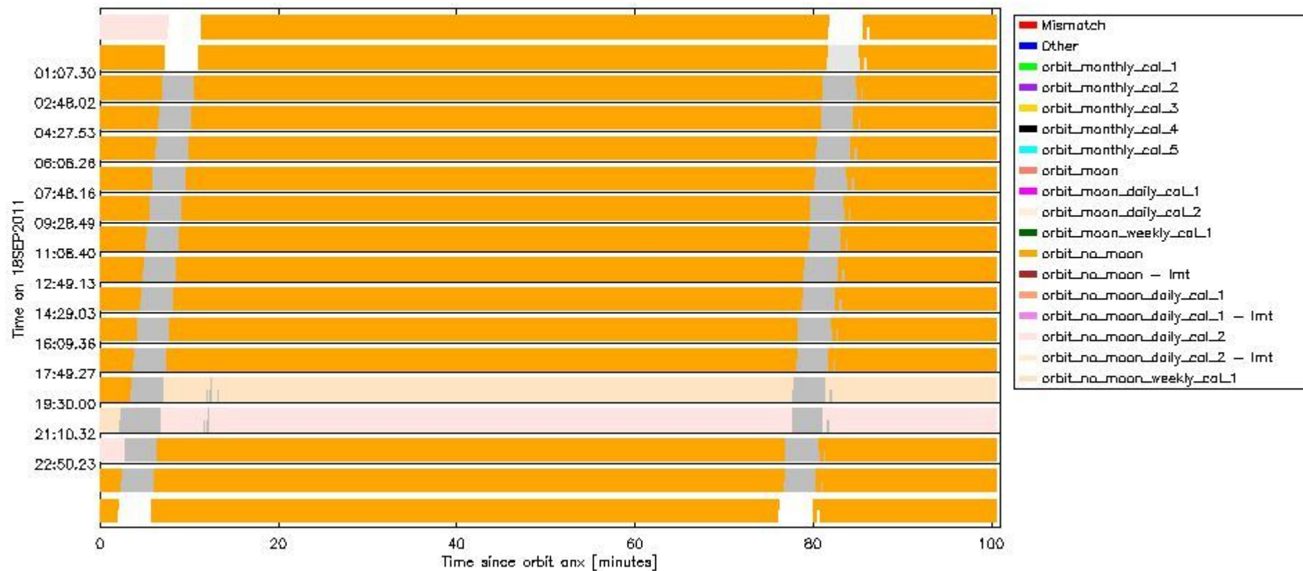
sciamachy_daily_report_level0_KSPT_L0_4504_N_20110918_6.PNG
