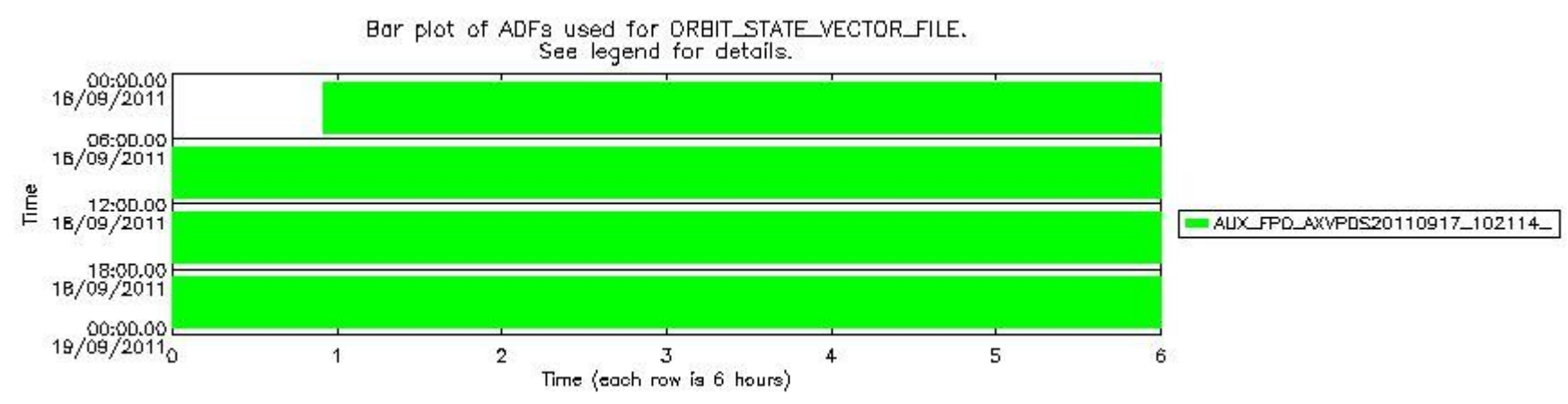
sciamachy_daily_report_level0_KSPT_L0_4504_N_20110918_8.PNG
