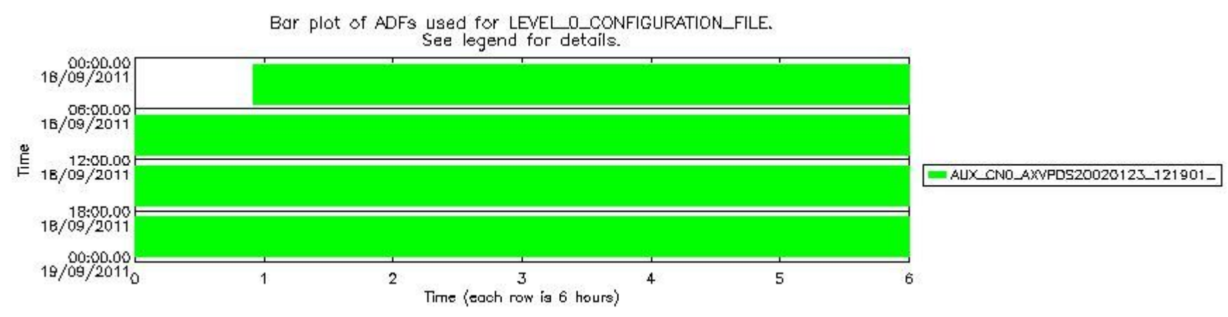
sciamachy_daily_report_level0_KSPT_L0_4504_N_20110918_7.PNG
