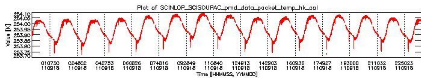
sciamachy_daily_report_level0_KSPT_L0_4504_N_20110918_3.PNG
