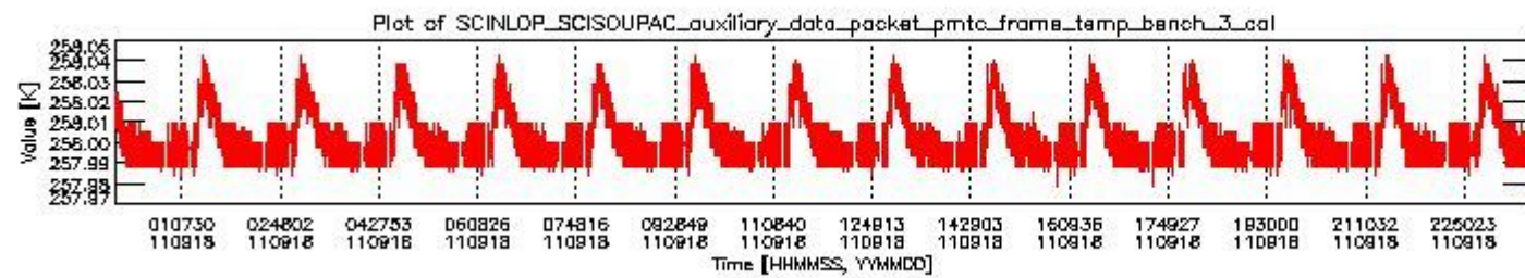
sciamachy_daily_report_level0_KSPT_L0_4504_N_20110918_2.PNG
