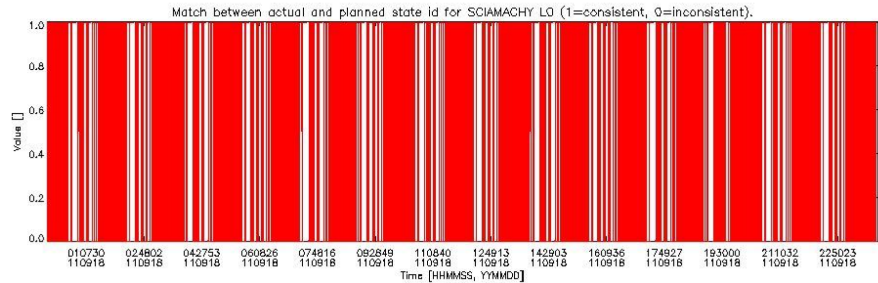
sciamachy_daily_report_level0_KSPT_L0_4504_N_20110918_5.PNG
