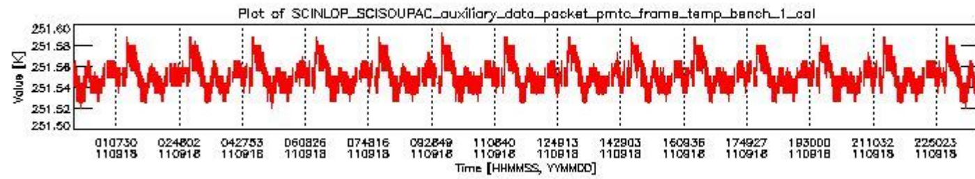
sciamachy_daily_report_level0_KSPT_L0_4504_N_20110918_0.PNG
