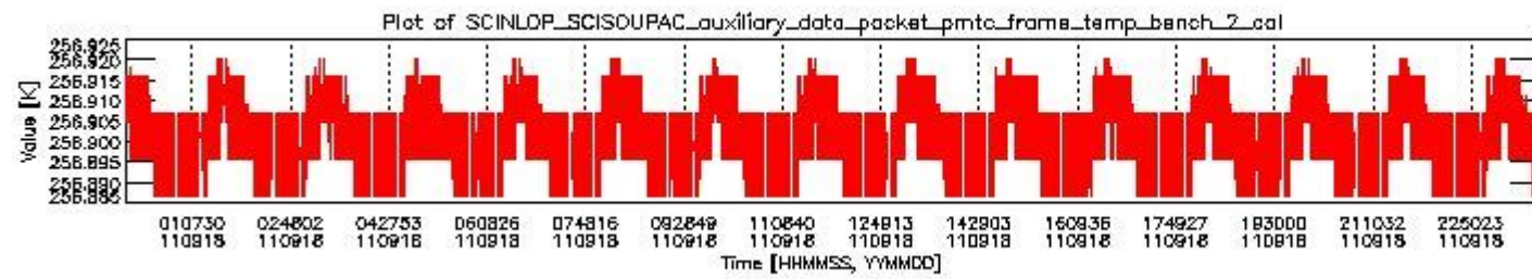
sciamachy_daily_report_level0_KSPT_L0_4504_N_20110918_1.PNG
