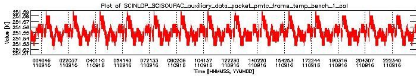
sciamachy_daily_report_level0_KSPT_L0_4504_N_20110916_0.PNG
