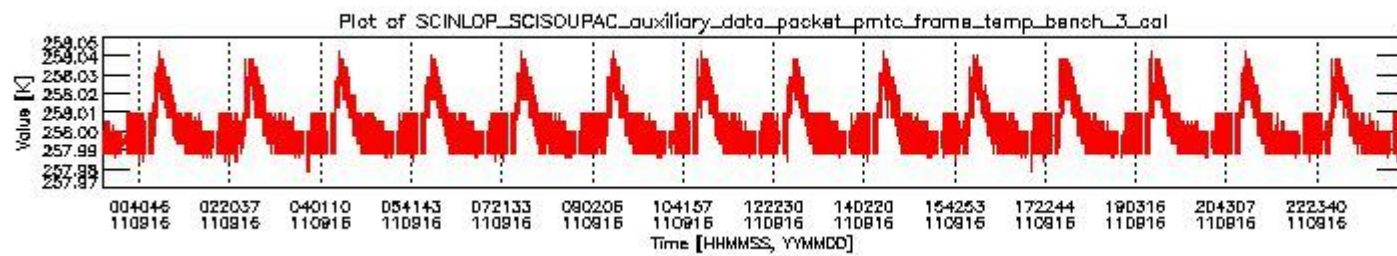
sciamachy_daily_report_level0_KSPT_L0_4504_N_20110916_2.PNG
