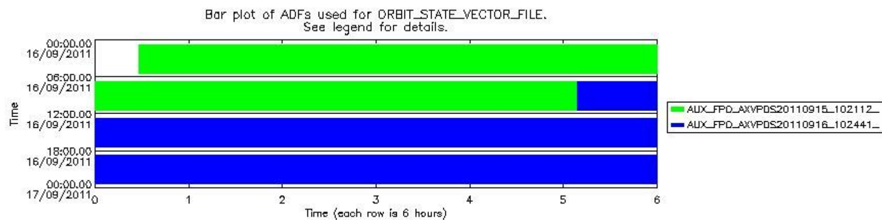
sciamachy_daily_report_level0_KSPT_L0_4504_N_20110916_8.PNG
