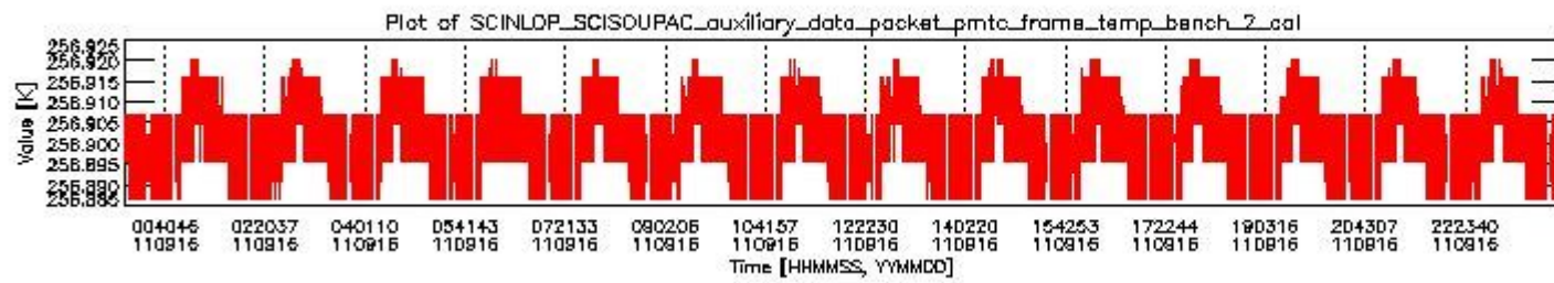
sciamachy_daily_report_level0_KSPT_L0_4504_N_20110916_1.PNG
