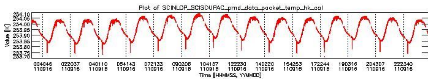
sciamachy_daily_report_level0_KSPT_L0_4504_N_20110916_3.PNG
