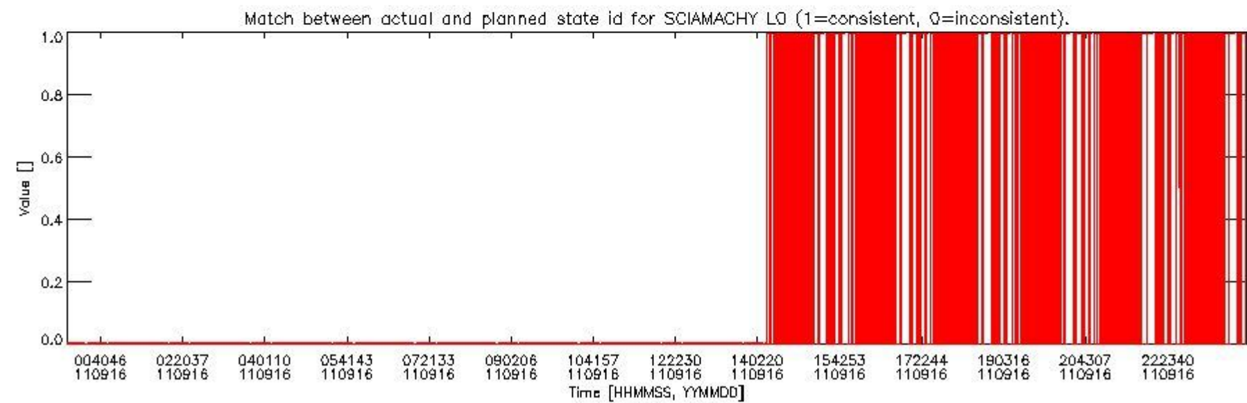
sciamachy_daily_report_level0_KSPT_L0_4504_N_20110916_5.PNG
