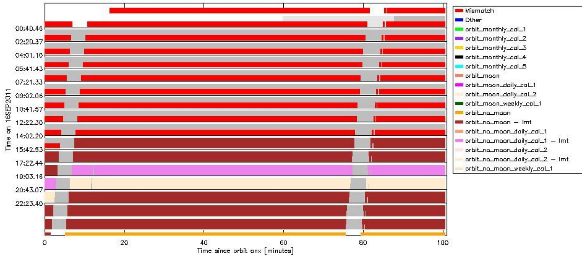
sciamachy_daily_report_level0_KSPT_L0_4504_N_20110916_6.PNG
