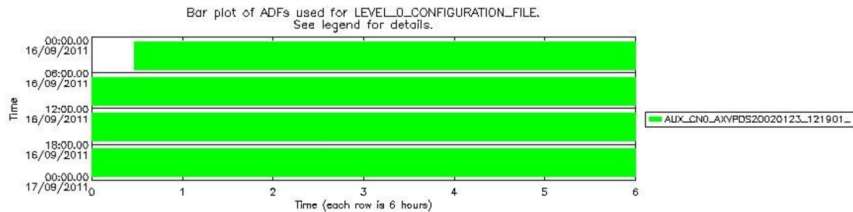
sciamachy_daily_report_level0_KSPT_L0_4504_N_20110916_7.PNG
