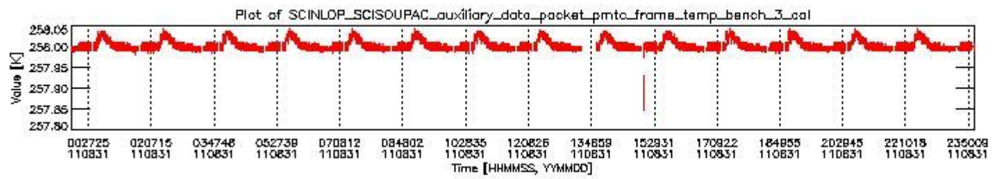
sciamachy_daily_report_level0_KSPT_L0_4504_N_20110831_2.PNG
