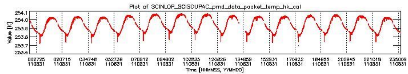
sciamachy_daily_report_level0_KSPT_L0_4504_N_20110831_3.PNG
