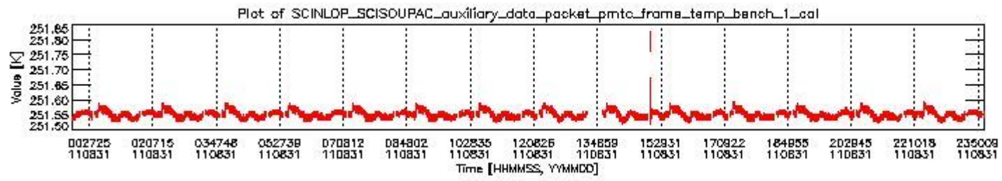
sciamachy_daily_report_level0_KSPT_L0_4504_N_20110831_0.PNG
