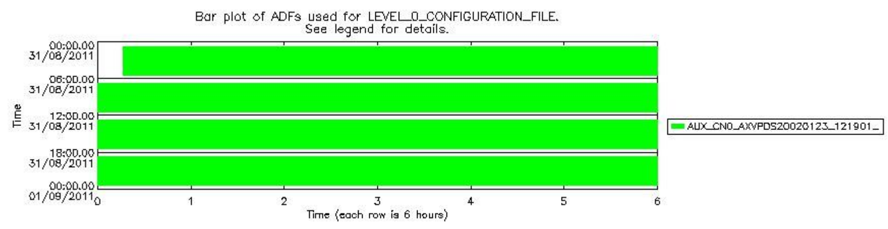
sciamachy_daily_report_level0_KSPT_L0_4504_N_20110831_7.PNG
