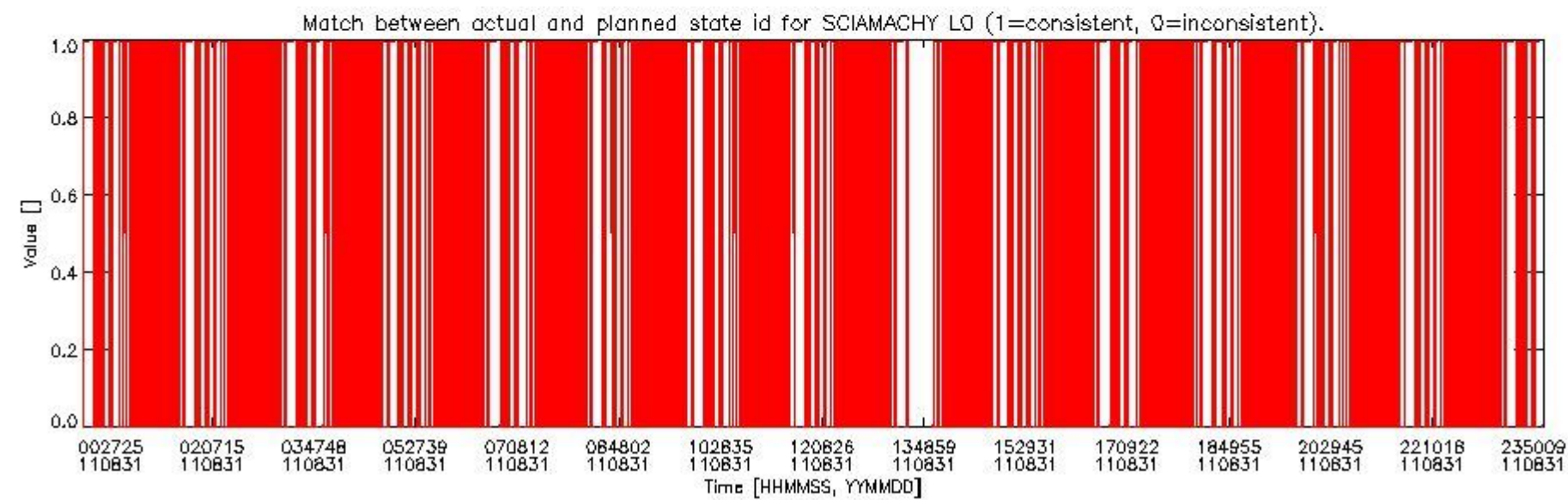
sciamachy_daily_report_level0_KSPT_L0_4504_N_20110831_5.PNG
