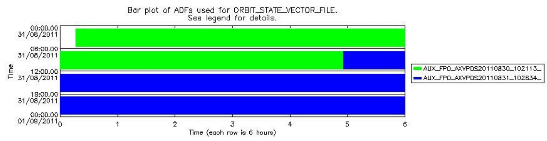
sciamachy_daily_report_level0_KSPT_L0_4504_N_20110831_8.PNG
