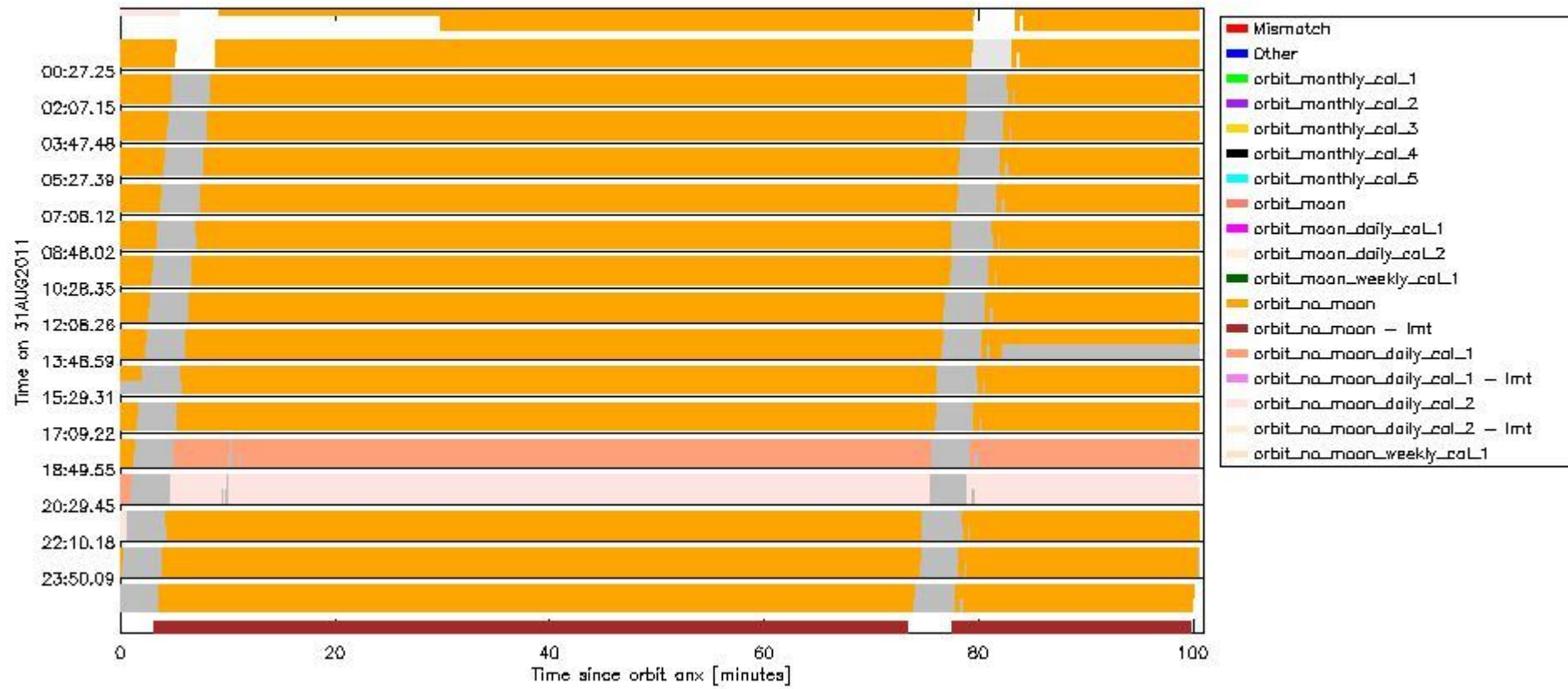
sciamachy_daily_report_level0_KSPT_L0_4504_N_20110831_6.PNG
