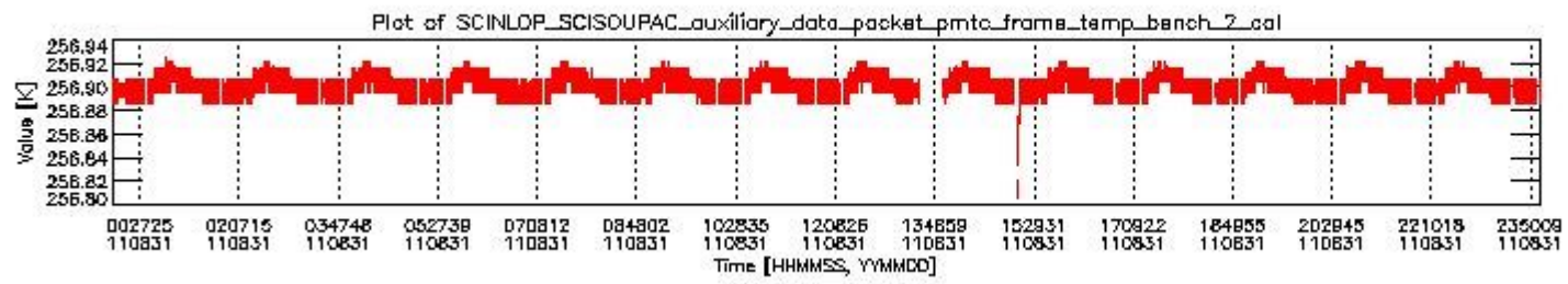
sciamachy_daily_report_level0_KSPT_L0_4504_N_20110831_1.PNG
