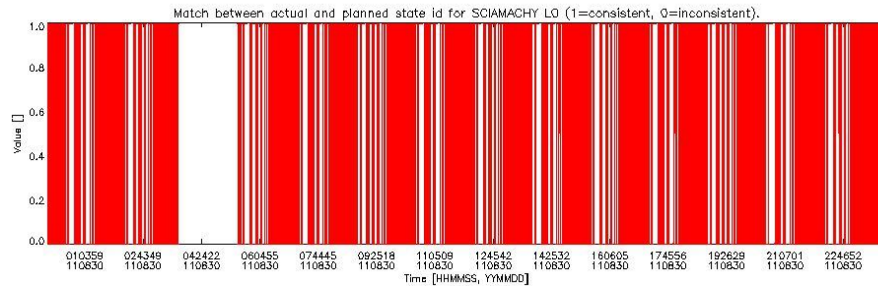
sciamachy_daily_report_level0_KSPT_L0_4504_N_20110830_5.PNG
