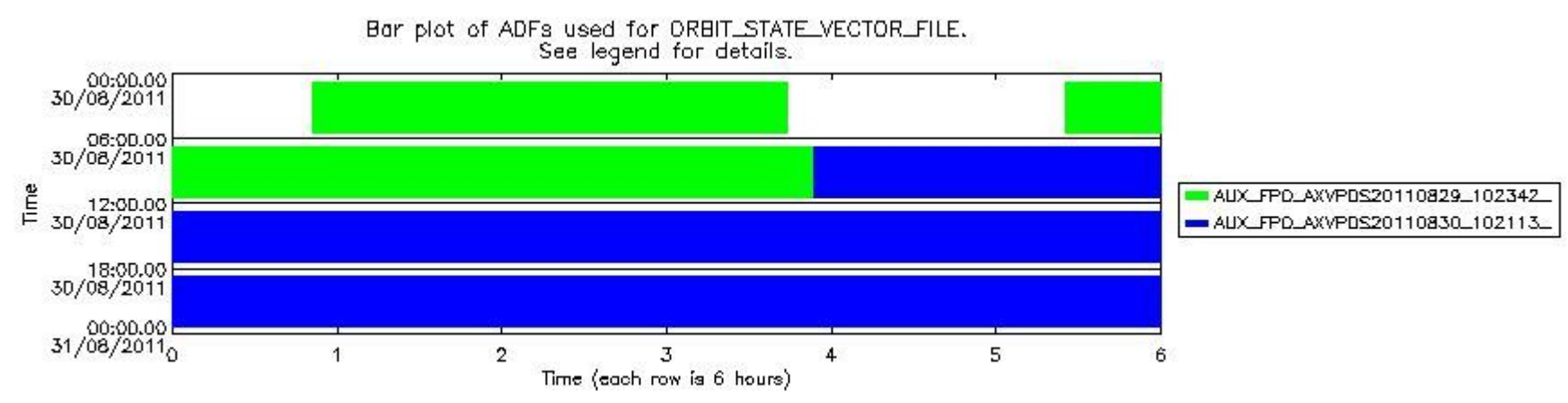
sciamachy_daily_report_level0_KSPT_L0_4504_N_20110830_8.PNG
