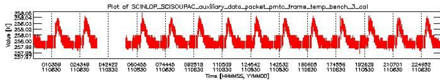
sciamachy_daily_report_level0_KSPT_L0_4504_N_20110830_2.PNG
