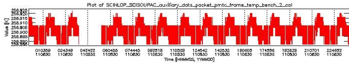
sciamachy_daily_report_level0_KSPT_L0_4504_N_20110830_1.PNG
