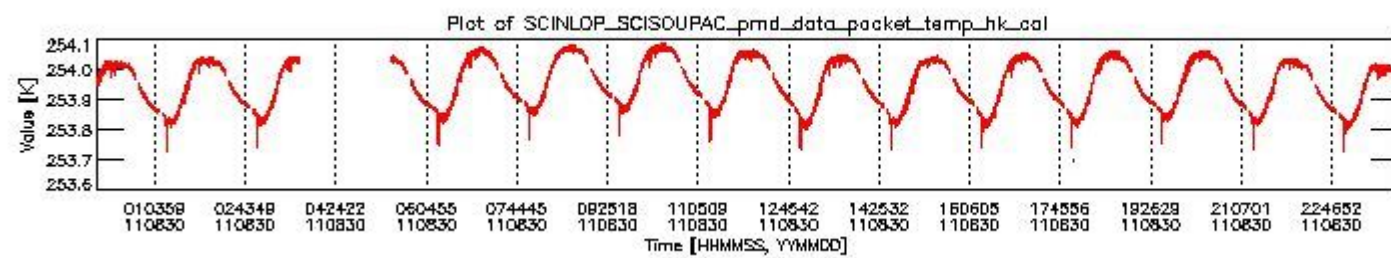
sciamachy_daily_report_level0_KSPT_L0_4504_N_20110830_3.PNG
