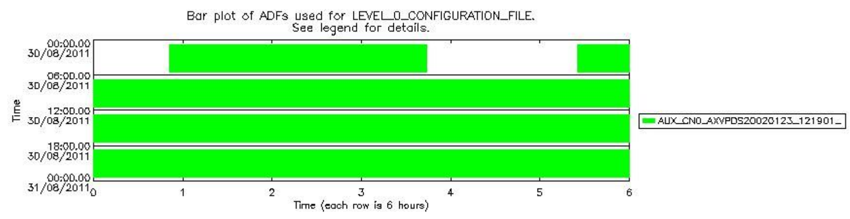
sciamachy_daily_report_level0_KSPT_L0_4504_N_20110830_7.PNG
