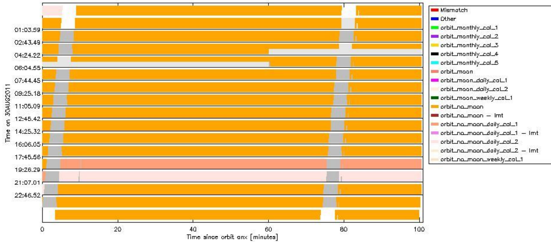
sciamachy_daily_report_level0_KSPT_L0_4504_N_20110830_6.PNG
