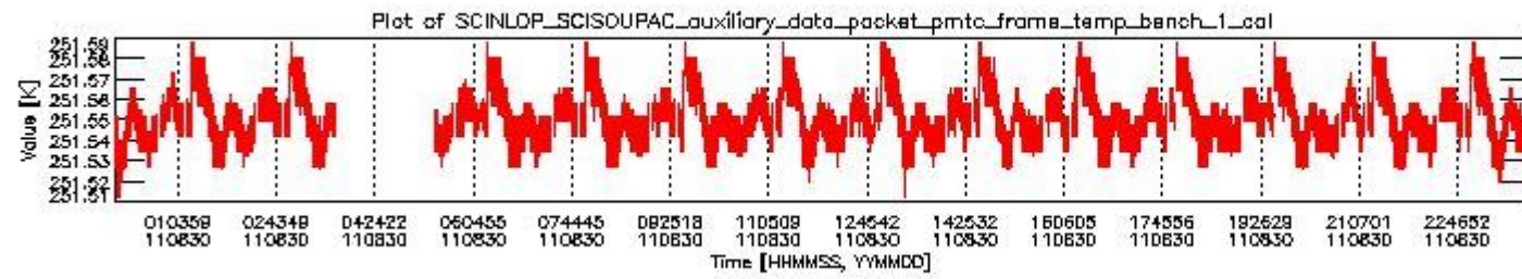
sciamachy_daily_report_level0_KSPT_L0_4504_N_20110830_0.PNG
