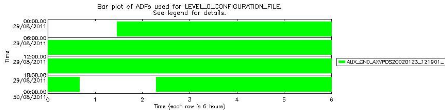
sciamachy_daily_report_level0_KSPT_L0_4504_N_20110829_7.PNG
