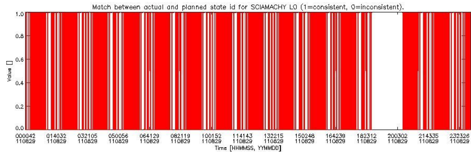
sciamachy_daily_report_level0_KSPT_L0_4504_N_20110829_5.PNG
