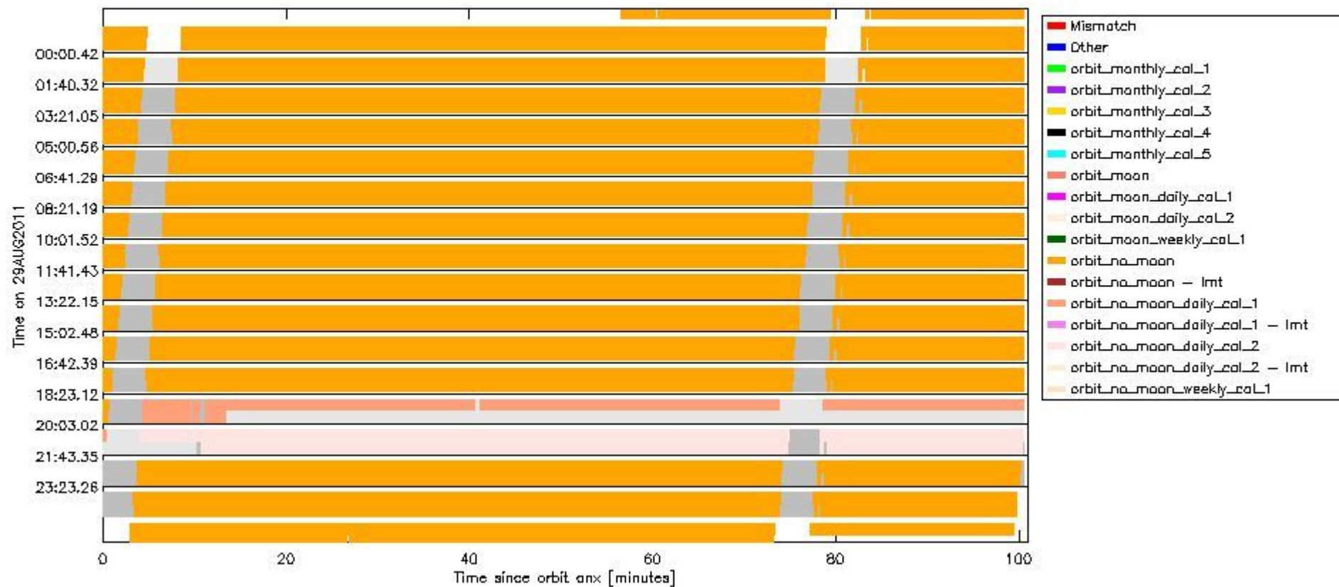
sciamachy_daily_report_level0_KSPT_L0_4504_N_20110829_6.PNG
