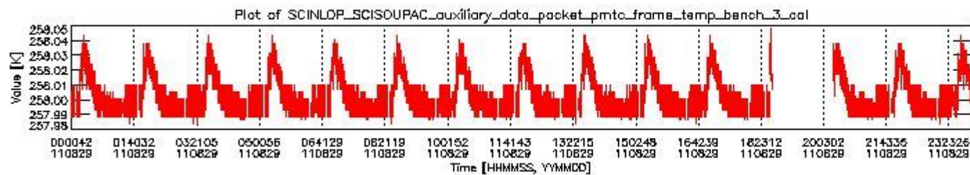
sciamachy_daily_report_level0_KSPT_L0_4504_N_20110829_2.PNG
