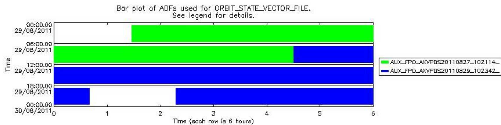
sciamachy_daily_report_level0_KSPT_L0_4504_N_20110829_8.PNG
