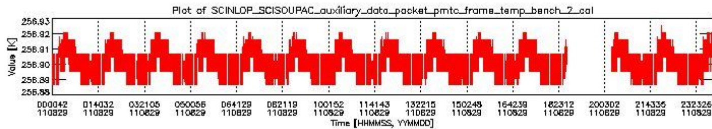
sciamachy_daily_report_level0_KSPT_L0_4504_N_20110829_1.PNG
