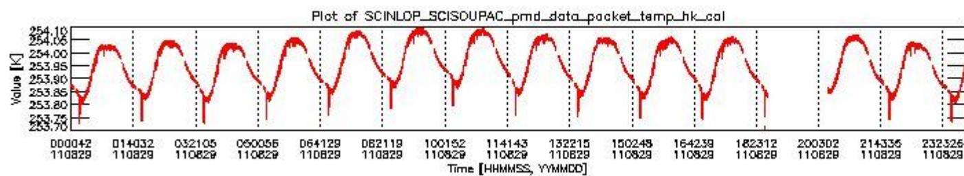
sciamachy_daily_report_level0_KSPT_L0_4504_N_20110829_3.PNG
