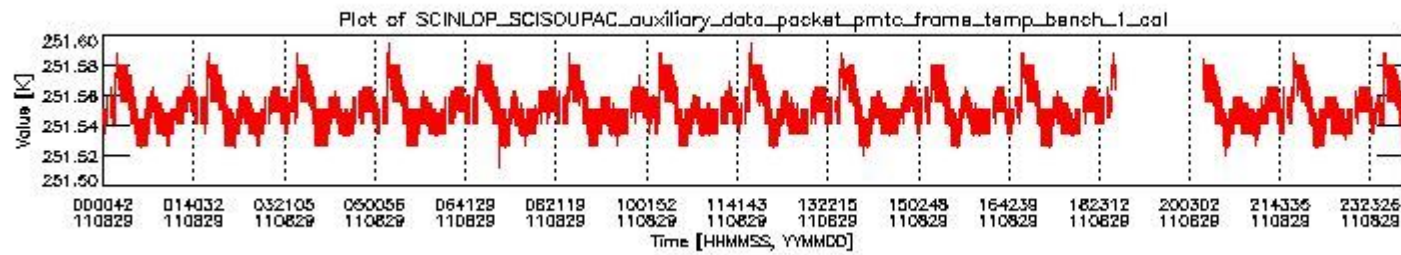
sciamachy_daily_report_level0_KSPT_L0_4504_N_20110829_0.PNG
