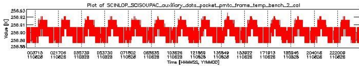
sciamachy_daily_report_level0_KSPT_L0_4504_N_20110828_1.PNG
