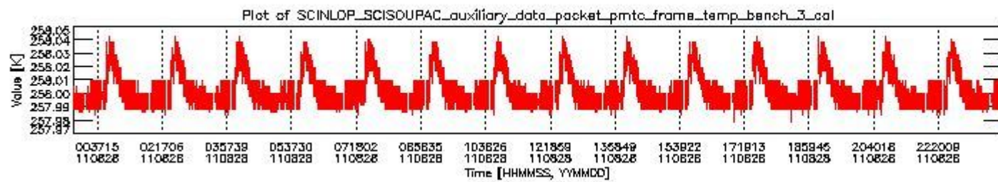
sciamachy_daily_report_level0_KSPT_L0_4504_N_20110828_2.PNG
