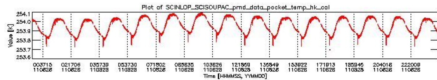
sciamachy_daily_report_level0_KSPT_L0_4504_N_20110828_3.PNG
