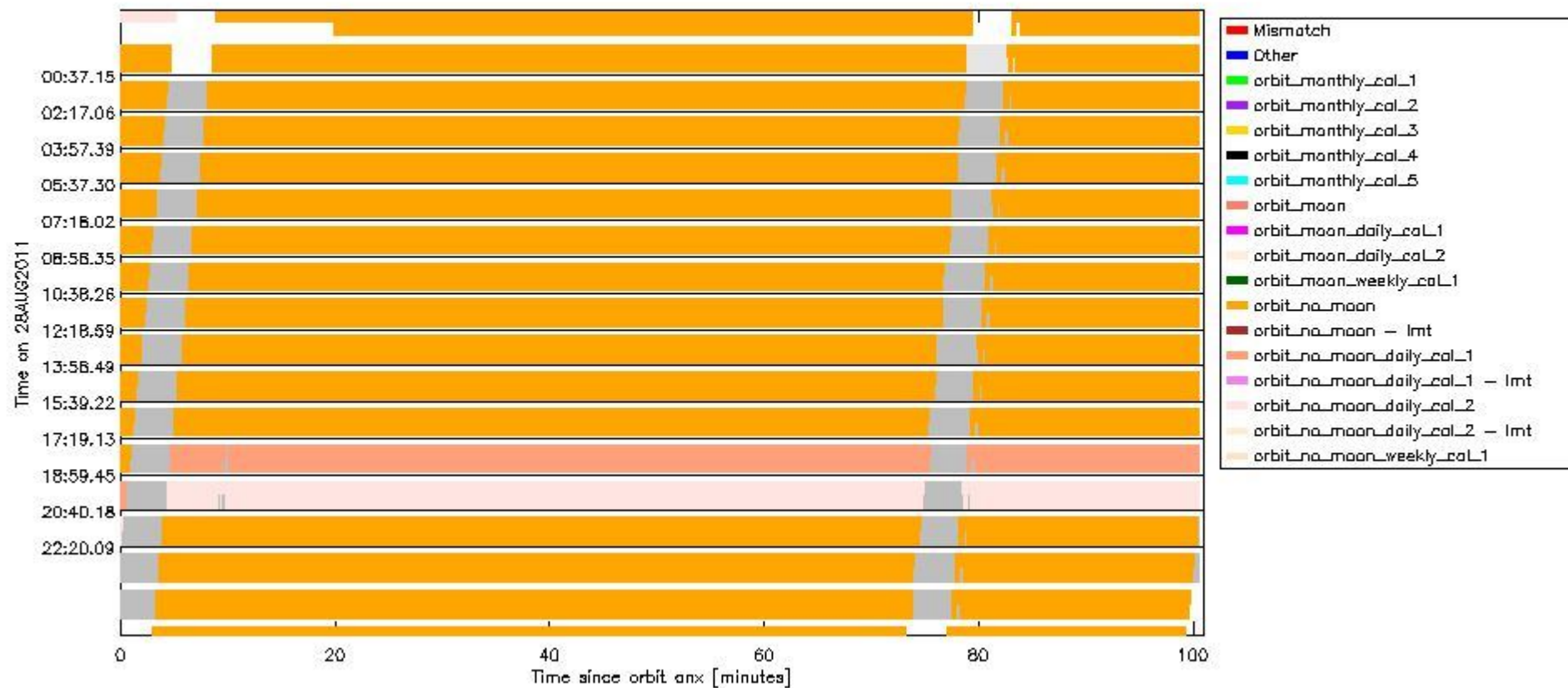
sciamachy_daily_report_level0_KSPT_L0_4504_N_20110828_6.PNG
