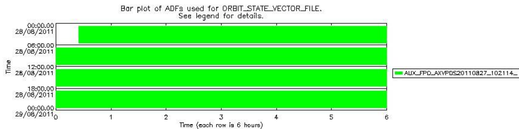
sciamachy_daily_report_level0_KSPT_L0_4504_N_20110828_8.PNG
