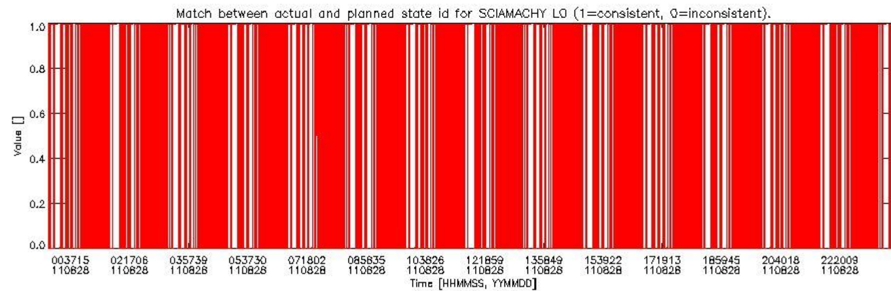
sciamachy_daily_report_level0_KSPT_L0_4504_N_20110828_5.PNG
