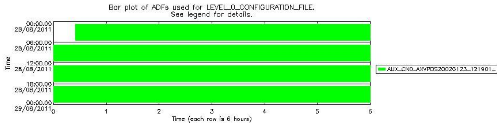
sciamachy_daily_report_level0_KSPT_L0_4504_N_20110828_7.PNG
