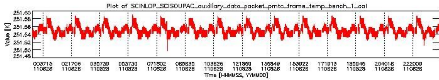
sciamachy_daily_report_level0_KSPT_L0_4504_N_20110828_0.PNG
