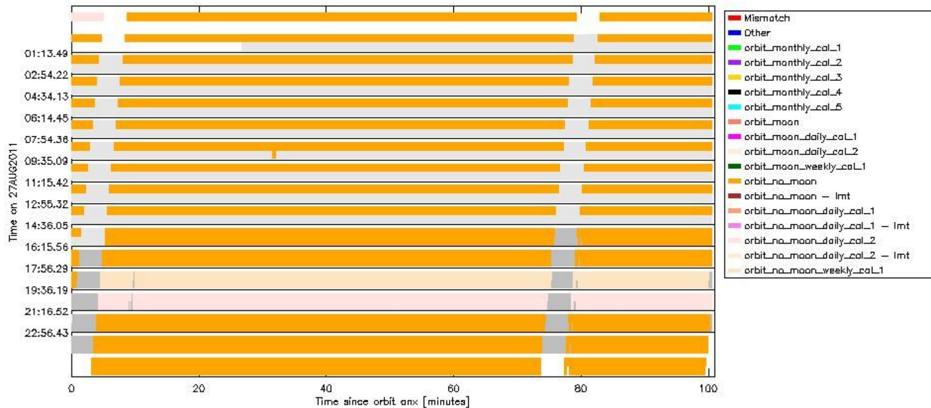
sciamachy_daily_report_level0_KSPT_L0_4504_N_20110827_6.PNG
