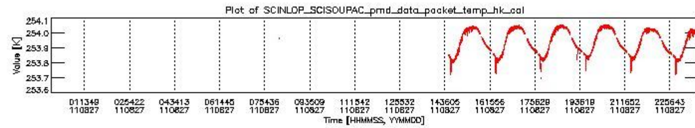
sciamachy_daily_report_level0_KSPT_L0_4504_N_20110827_3.PNG
