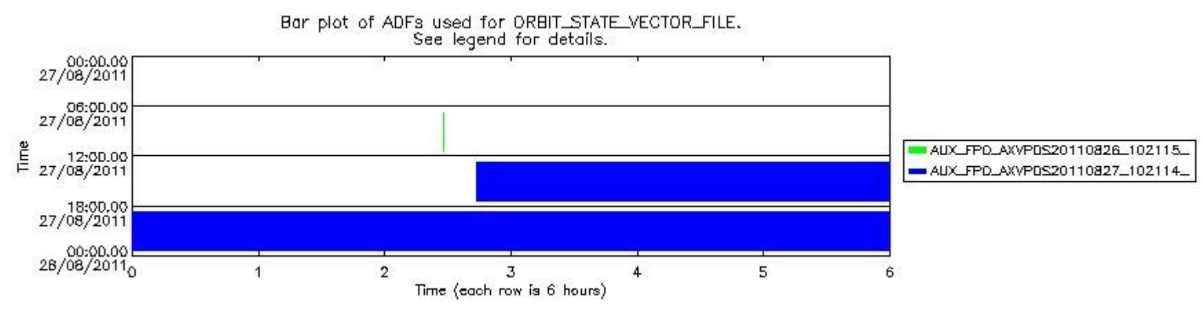
sciamachy_daily_report_level0_KSPT_L0_4504_N_20110827_8.PNG
