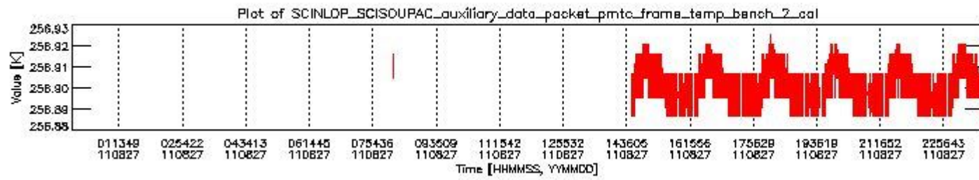
sciamachy_daily_report_level0_KSPT_L0_4504_N_20110827_1.PNG
