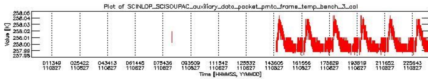
sciamachy_daily_report_level0_KSPT_L0_4504_N_20110827_2.PNG
