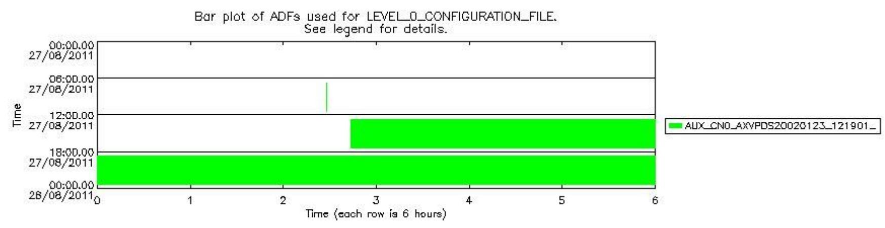
sciamachy_daily_report_level0_KSPT_L0_4504_N_20110827_7.PNG
