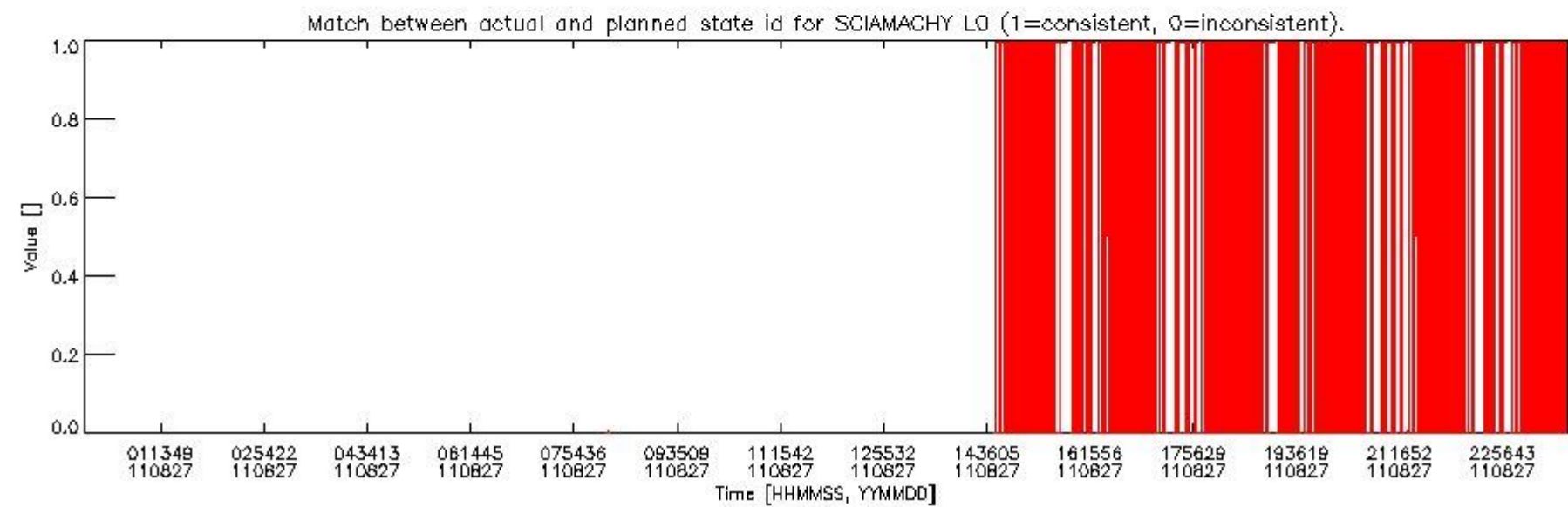
sciamachy_daily_report_level0_KSPT_L0_4504_N_20110827_5.PNG
