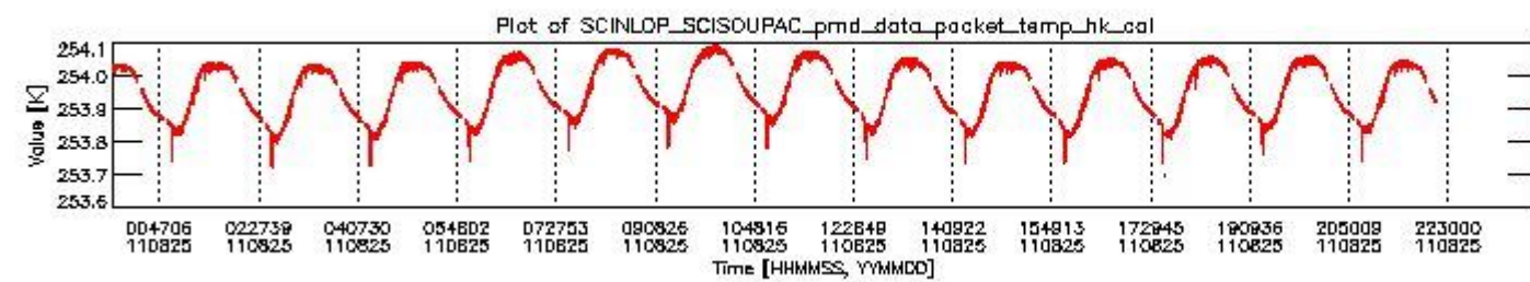
sciamachy_daily_report_level0_KSPT_L0_4504_N_20110825_3.PNG
