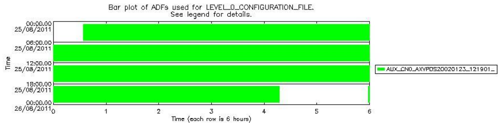
sciamachy_daily_report_level0_KSPT_L0_4504_N_20110825_7.PNG
