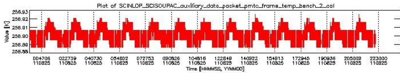
sciamachy_daily_report_level0_KSPT_L0_4504_N_20110825_1.PNG
