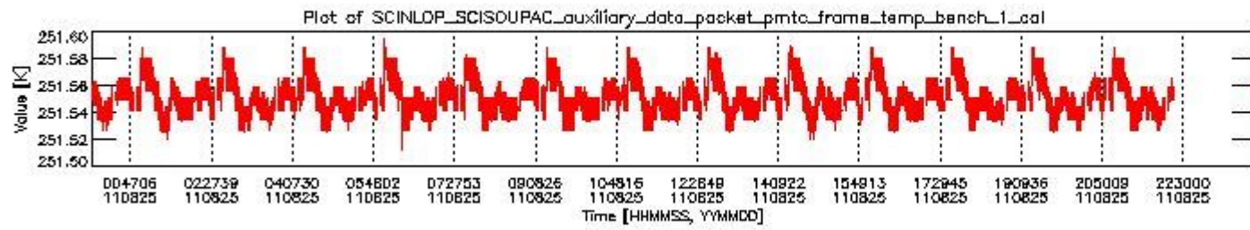
sciamachy_daily_report_level0_KSPT_L0_4504_N_20110825_0.PNG
