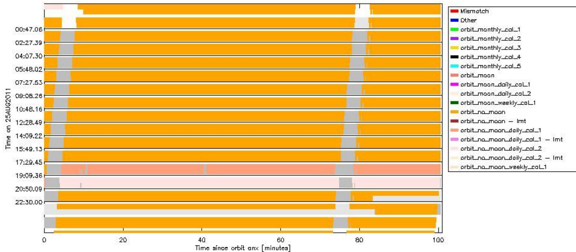
sciamachy_daily_report_level0_KSPT_L0_4504_N_20110825_6.PNG
