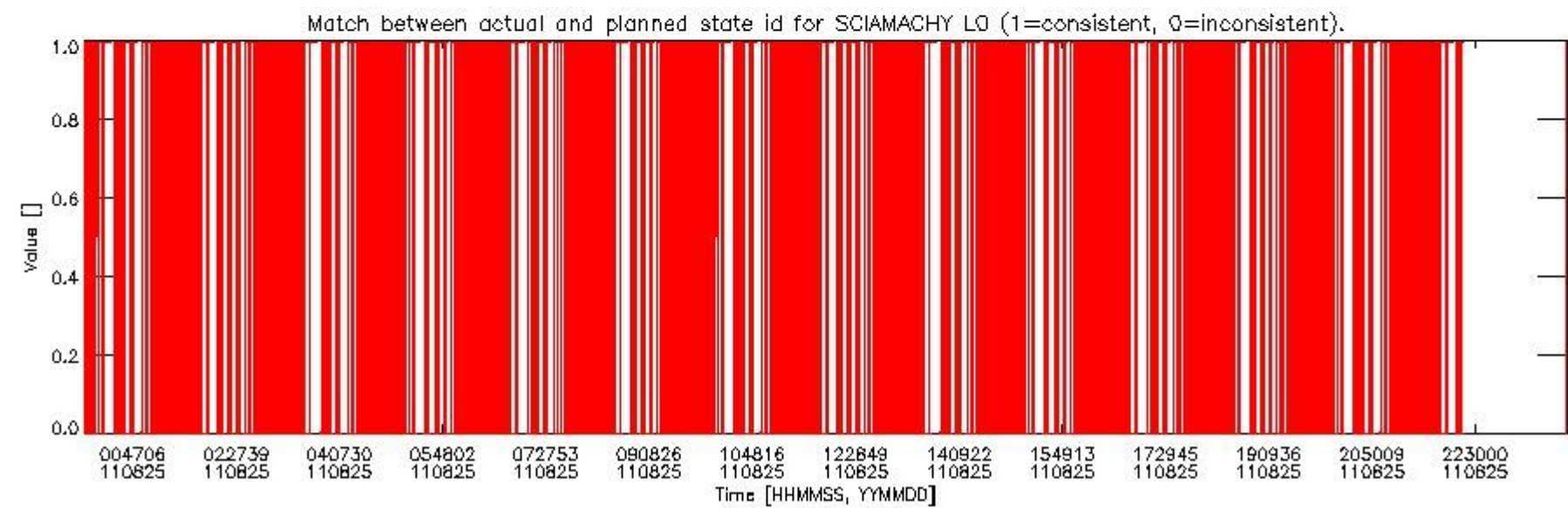
sciamachy_daily_report_level0_KSPT_L0_4504_N_20110825_5.PNG
