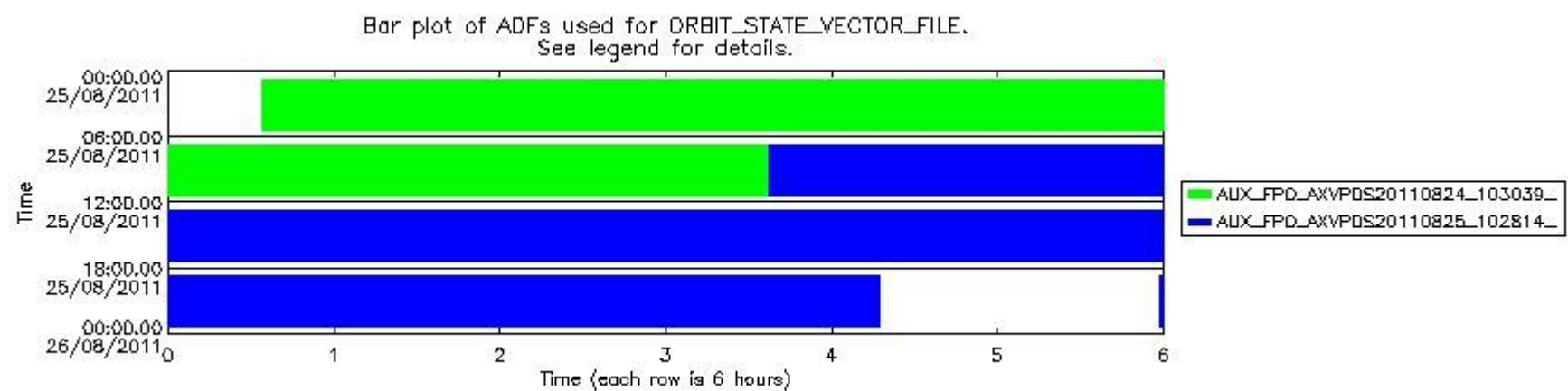
sciamachy_daily_report_level0_KSPT_L0_4504_N_20110825_8.PNG
