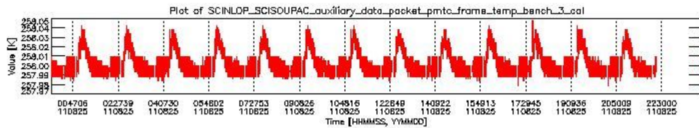
sciamachy_daily_report_level0_KSPT_L0_4504_N_20110825_2.PNG
