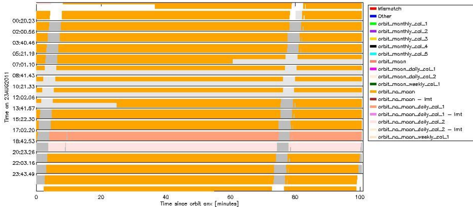
sciamachy_daily_report_level0_KSPT_L0_4504_N_20110823_6.PNG
