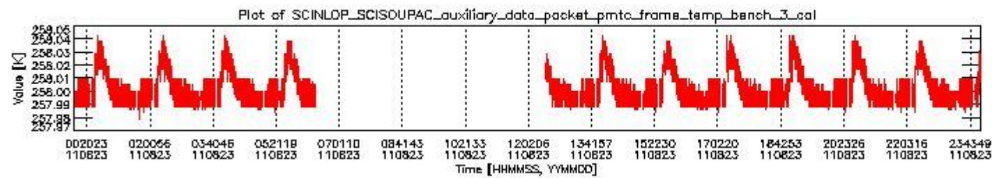
sciamachy_daily_report_level0_KSPT_L0_4504_N_20110823_2.PNG
