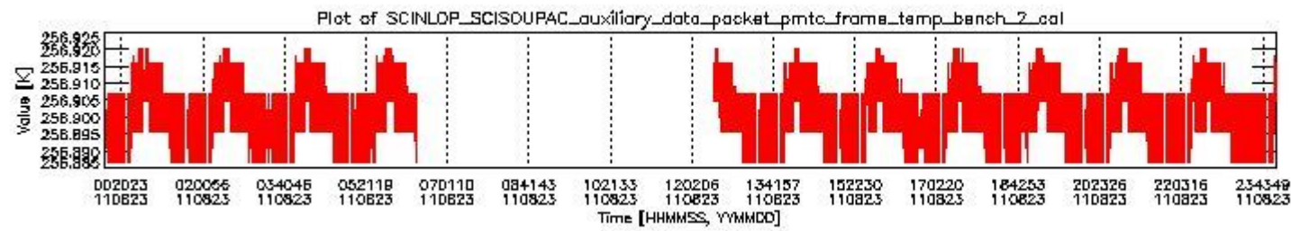
sciamachy_daily_report_level0_KSPT_L0_4504_N_20110823_1.PNG
