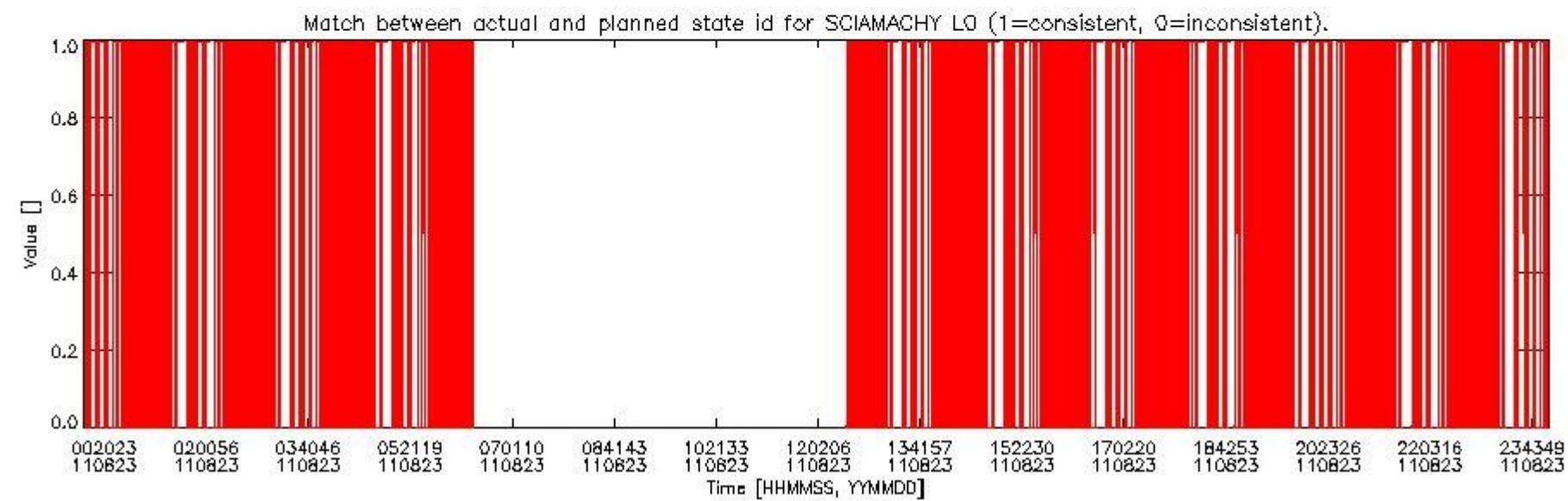
sciamachy_daily_report_level0_KSPT_L0_4504_N_20110823_5.PNG
