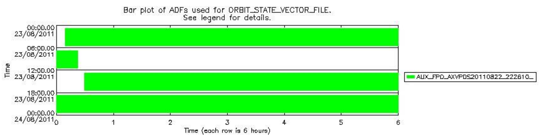
sciamachy_daily_report_level0_KSPT_L0_4504_N_20110823_8.PNG
