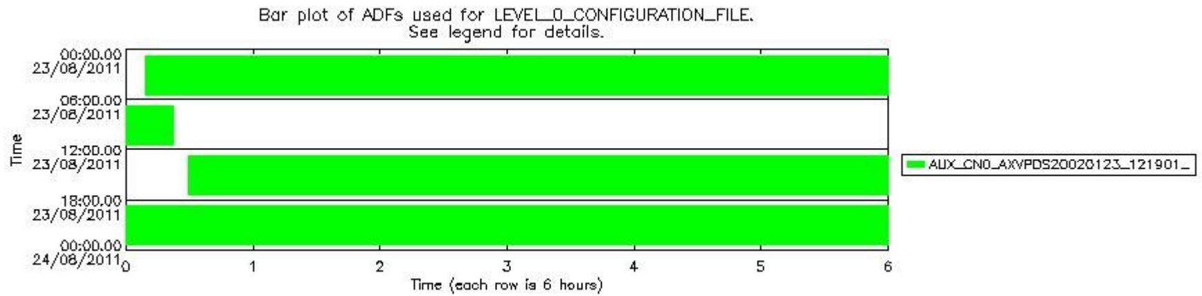
sciamachy_daily_report_level0_KSPT_L0_4504_N_20110823_7.PNG
