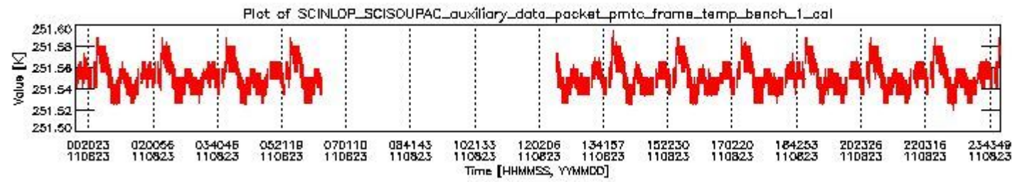
sciamachy_daily_report_level0_KSPT_L0_4504_N_20110823_0.PNG
