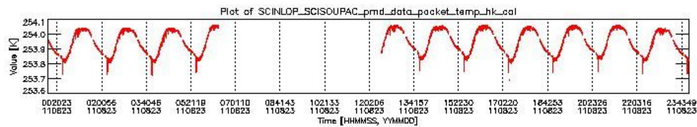
sciamachy_daily_report_level0_KSPT_L0_4504_N_20110823_3.PNG
