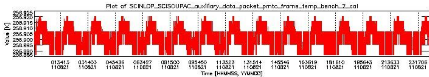
sciamachy_daily_report_level0_KSPT_L0_4504_N_20110821_1.PNG
