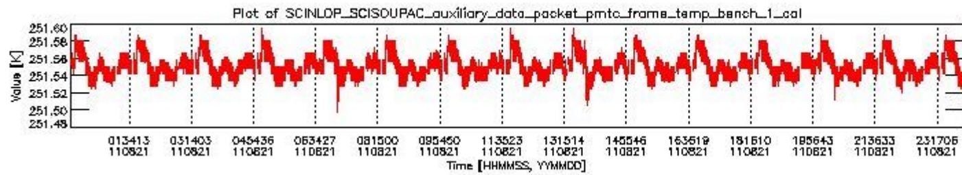
sciamachy_daily_report_level0_KSPT_L0_4504_N_20110821_0.PNG
