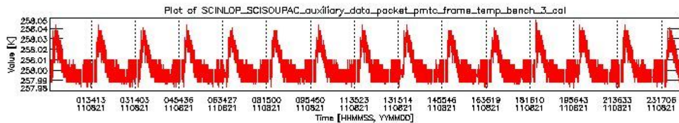
sciamachy_daily_report_level0_KSPT_L0_4504_N_20110821_2.PNG
