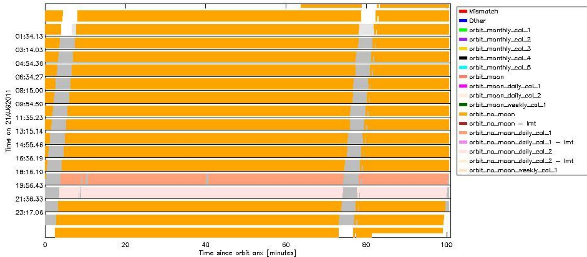
sciamachy_daily_report_level0_KSPT_L0_4504_N_20110821_6.PNG
