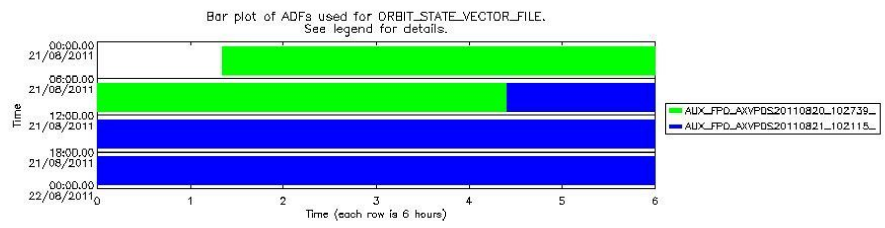
sciamachy_daily_report_level0_KSPT_L0_4504_N_20110821_8.PNG
