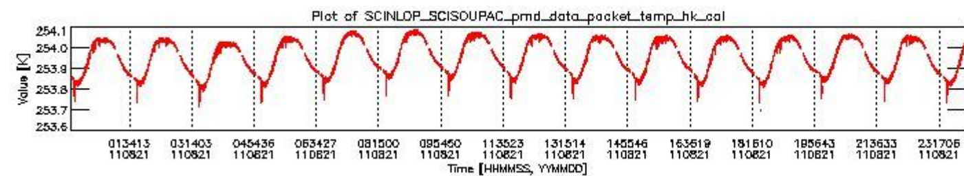
sciamachy_daily_report_level0_KSPT_L0_4504_N_20110821_3.PNG
