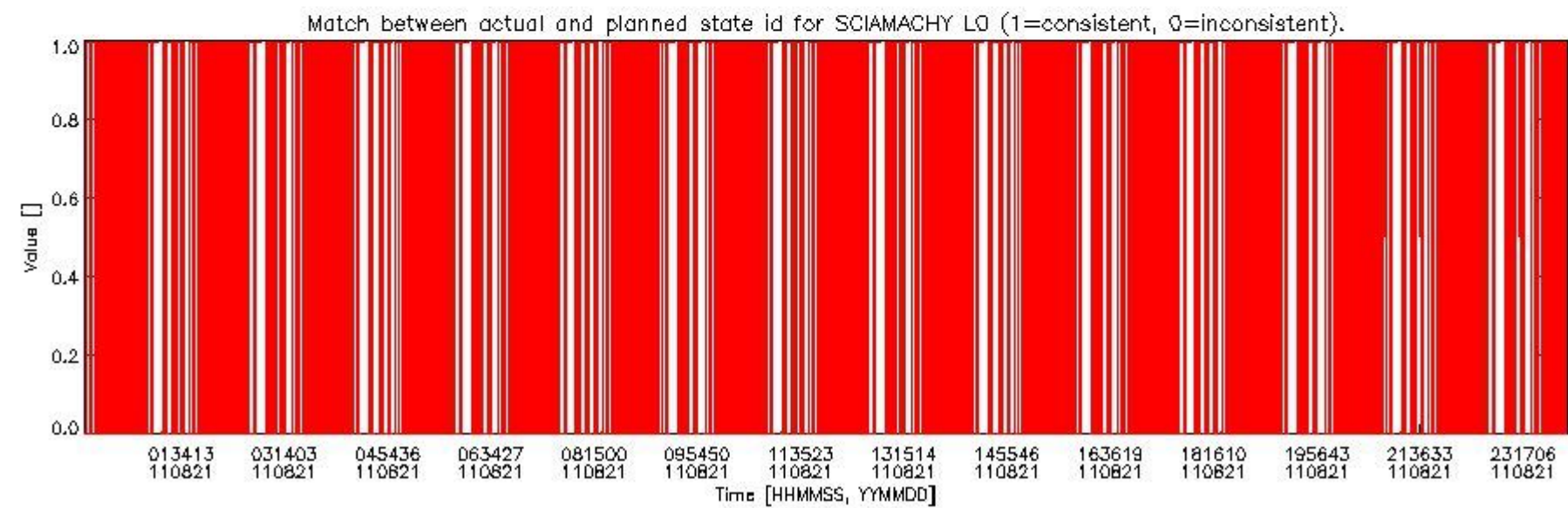
sciamachy_daily_report_level0_KSPT_L0_4504_N_20110821_5.PNG
