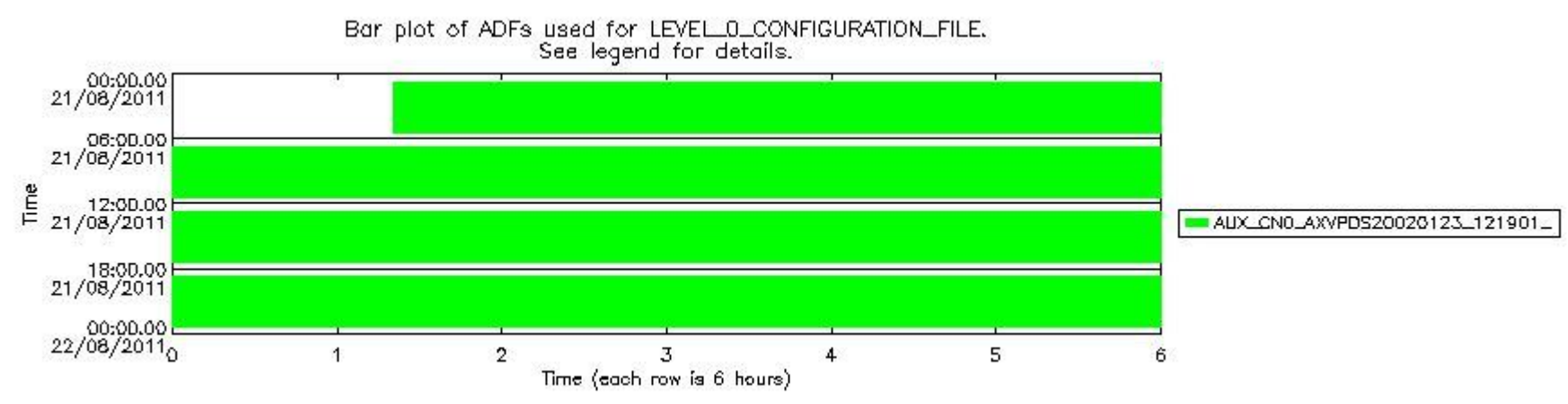
sciamachy_daily_report_level0_KSPT_L0_4504_N_20110821_7.PNG
