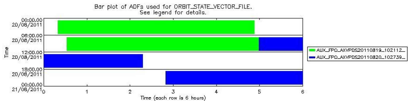
sciamachy_daily_report_level0_KSPT_L0_4504_N_20110820_8.PNG
