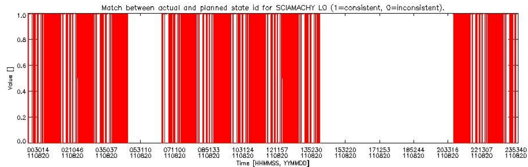
sciamachy_daily_report_level0_KSPT_L0_4504_N_20110820_5.PNG
