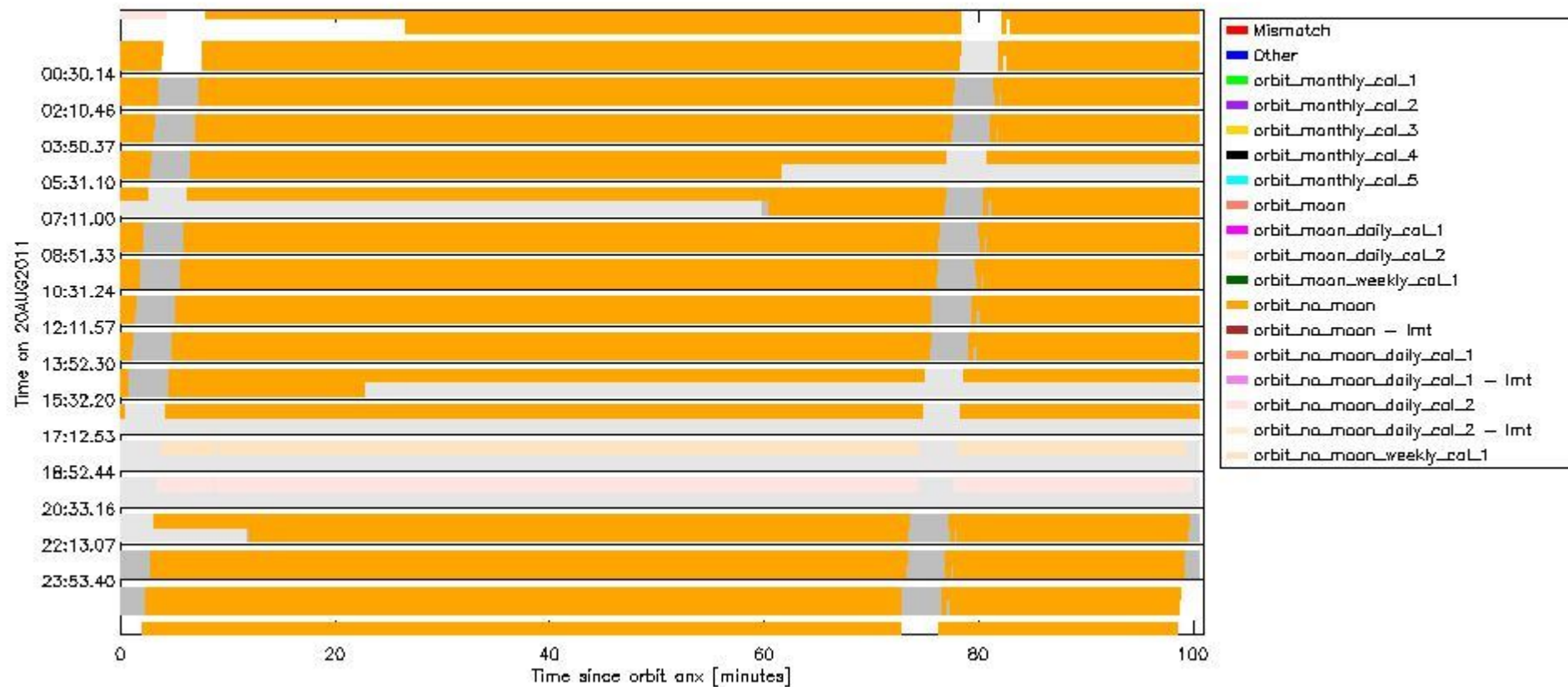
sciamachy_daily_report_level0_KSPT_L0_4504_N_20110820_6.PNG
