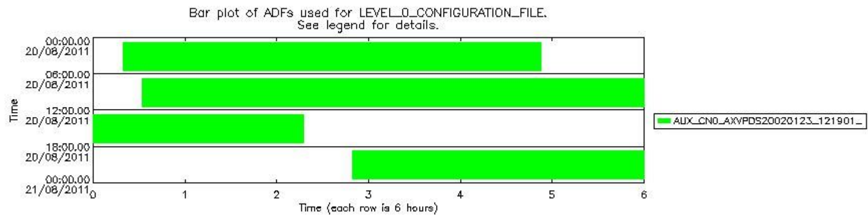
sciamachy_daily_report_level0_KSPT_L0_4504_N_20110820_7.PNG
