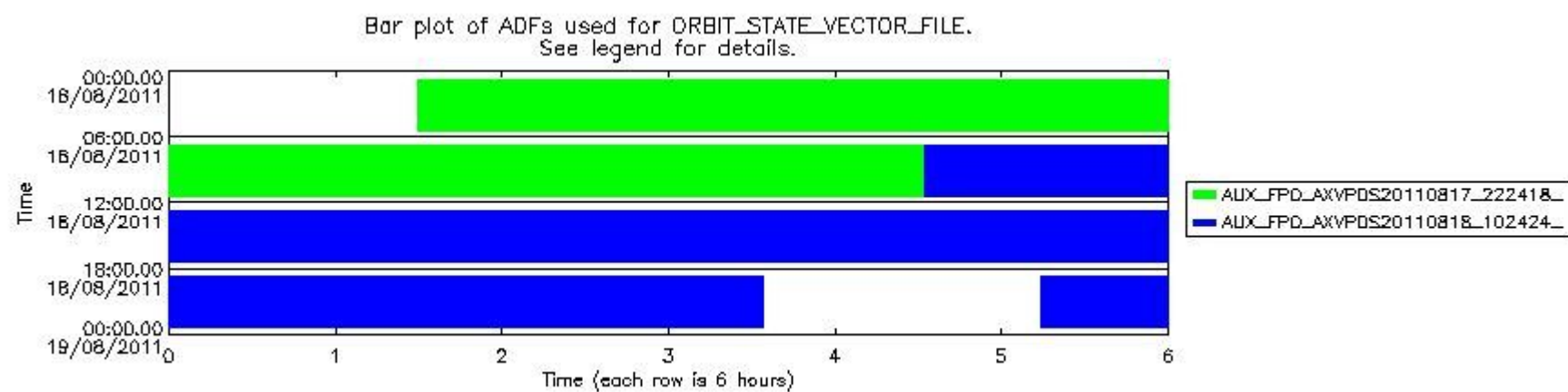
sciamachy_daily_report_level0_KSPT_L0_4504_N_20110818_8.PNG
