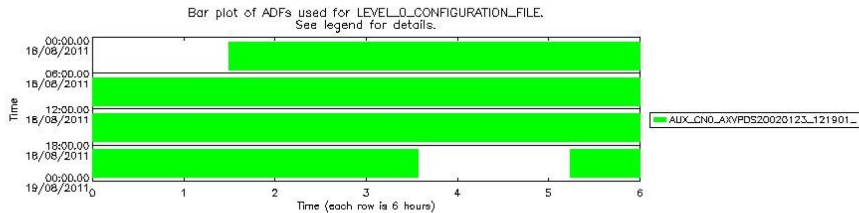
sciamachy_daily_report_level0_KSPT_L0_4504_N_20110818_7.PNG
