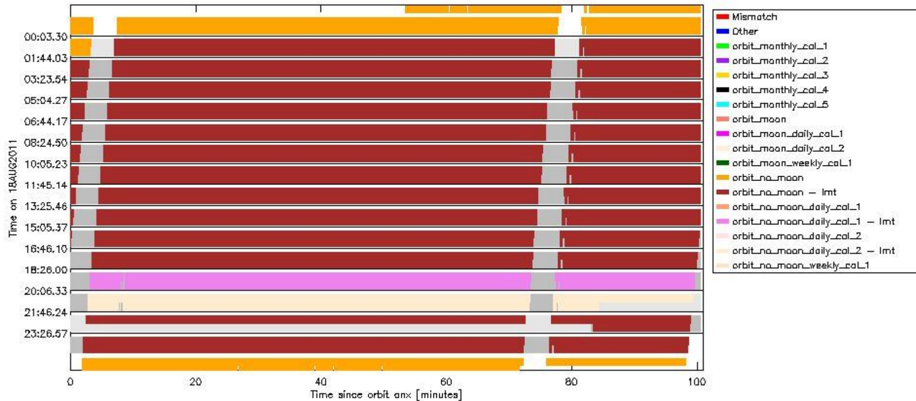
sciamachy_daily_report_level0_KSPT_L0_4504_N_20110818_6.PNG
