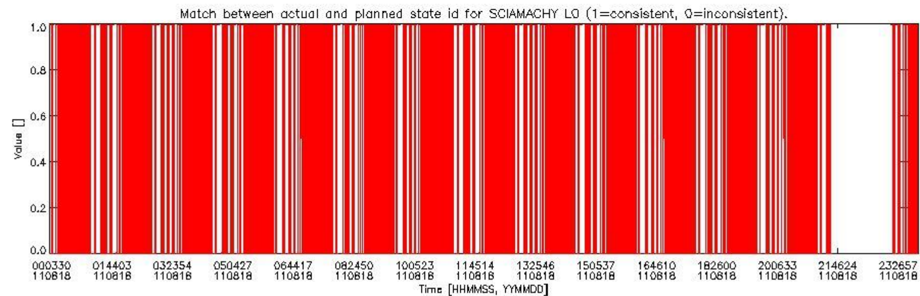
sciamachy_daily_report_level0_KSPT_L0_4504_N_20110818_5.PNG
