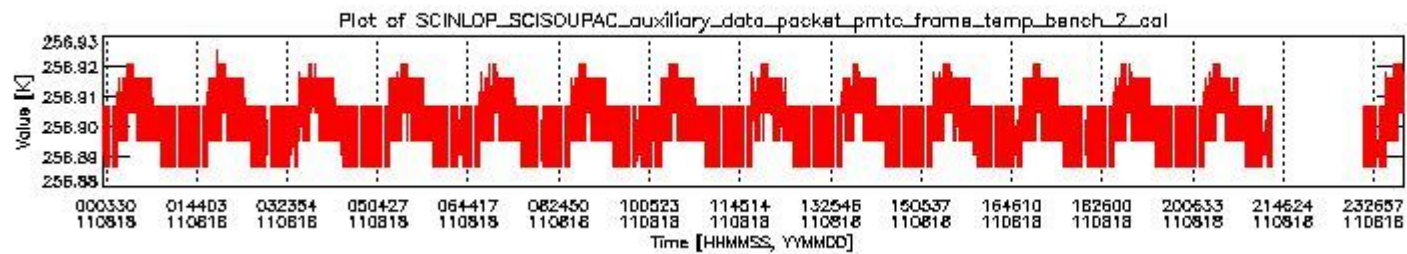
sciamachy_daily_report_level0_KSPT_L0_4504_N_20110818_1.PNG
