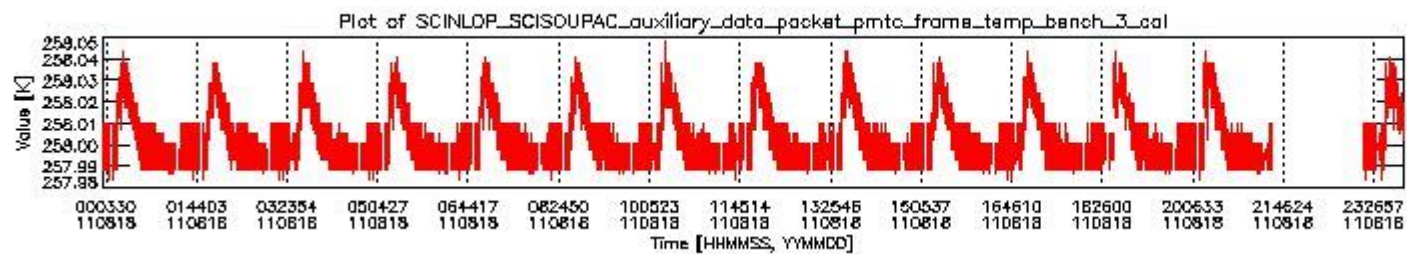
sciamachy_daily_report_level0_KSPT_L0_4504_N_20110818_2.PNG
