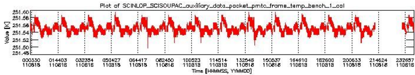
sciamachy_daily_report_level0_KSPT_L0_4504_N_20110818_0.PNG
