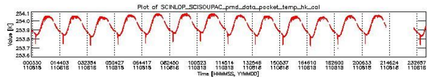
sciamachy_daily_report_level0_KSPT_L0_4504_N_20110818_3.PNG
