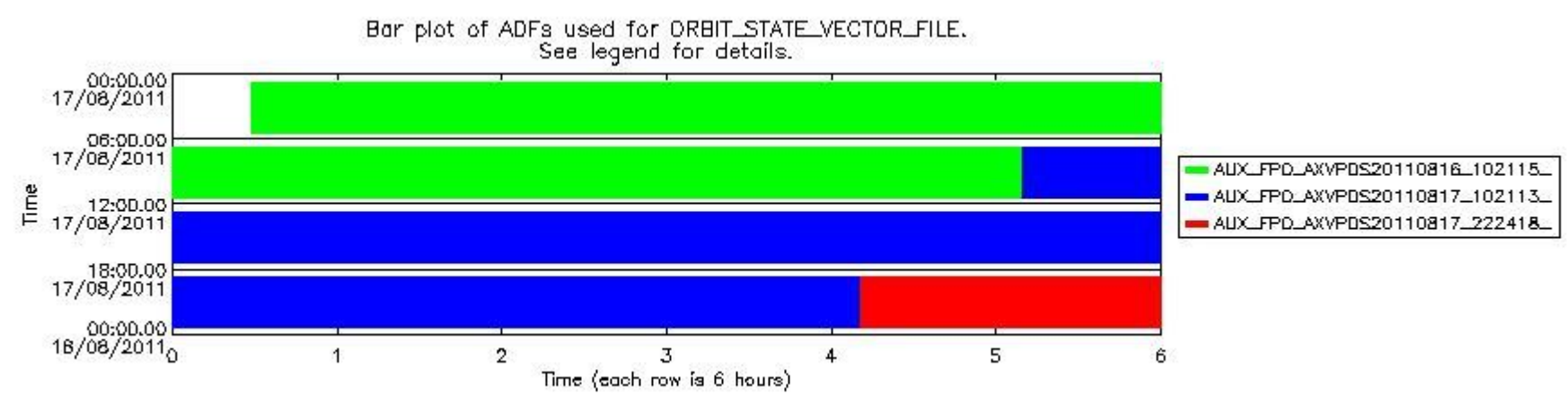
sciamachy_daily_report_level0_KSPT_L0_4504_N_20110817_8.PNG
