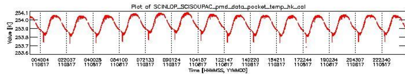
sciamachy_daily_report_level0_KSPT_L0_4504_N_20110817_3.PNG
