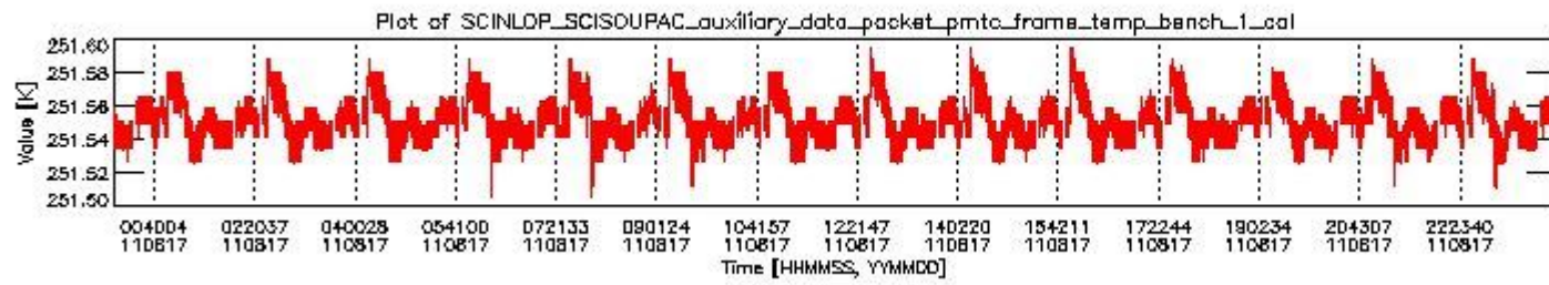
sciamachy_daily_report_level0_KSPT_L0_4504_N_20110817_0.PNG
