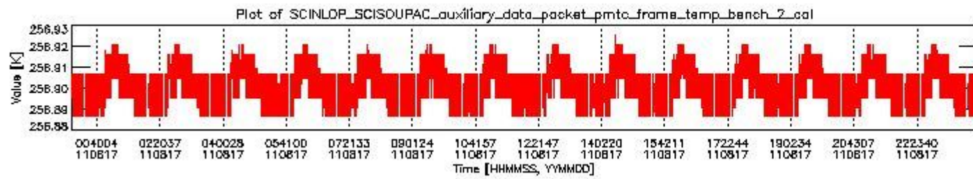
sciamachy_daily_report_level0_KSPT_L0_4504_N_20110817_1.PNG
