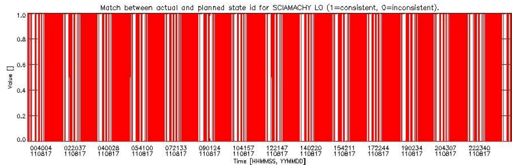
sciamachy_daily_report_level0_KSPT_L0_4504_N_20110817_5.PNG
