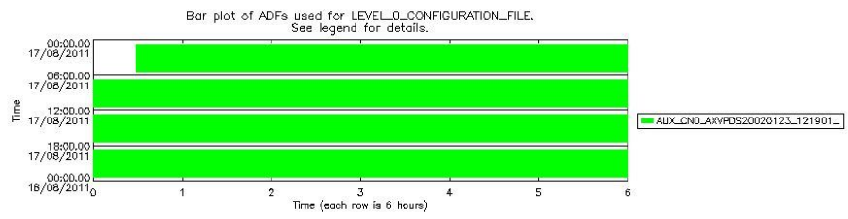
sciamachy_daily_report_level0_KSPT_L0_4504_N_20110817_7.PNG
