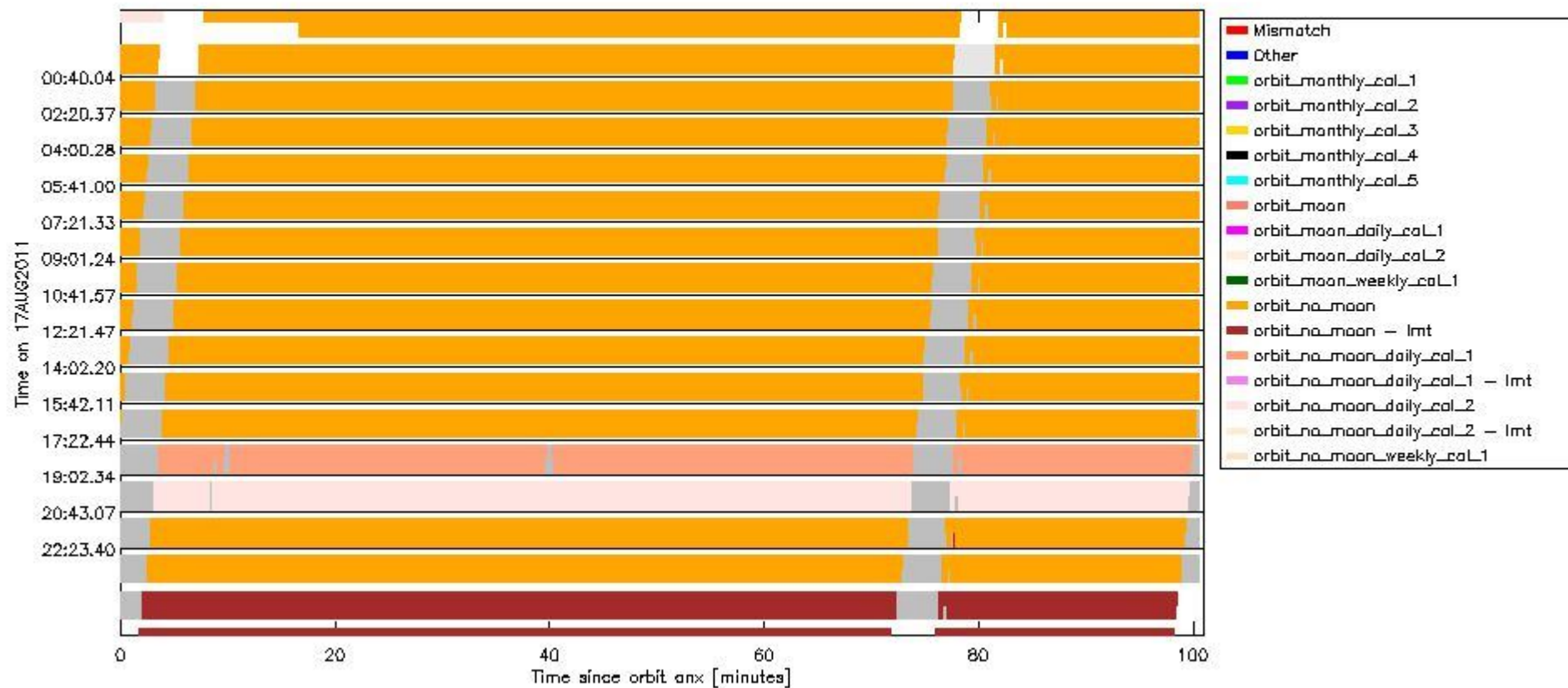
sciamachy_daily_report_level0_KSPT_L0_4504_N_20110817_6.PNG
