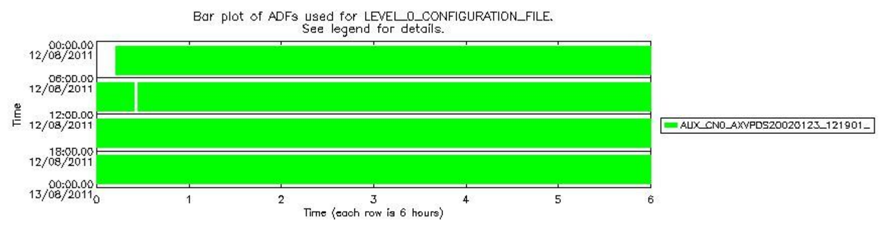
sciamachy_daily_report_level0_KSPT_L0_4504_N_20110812_7.PNG
