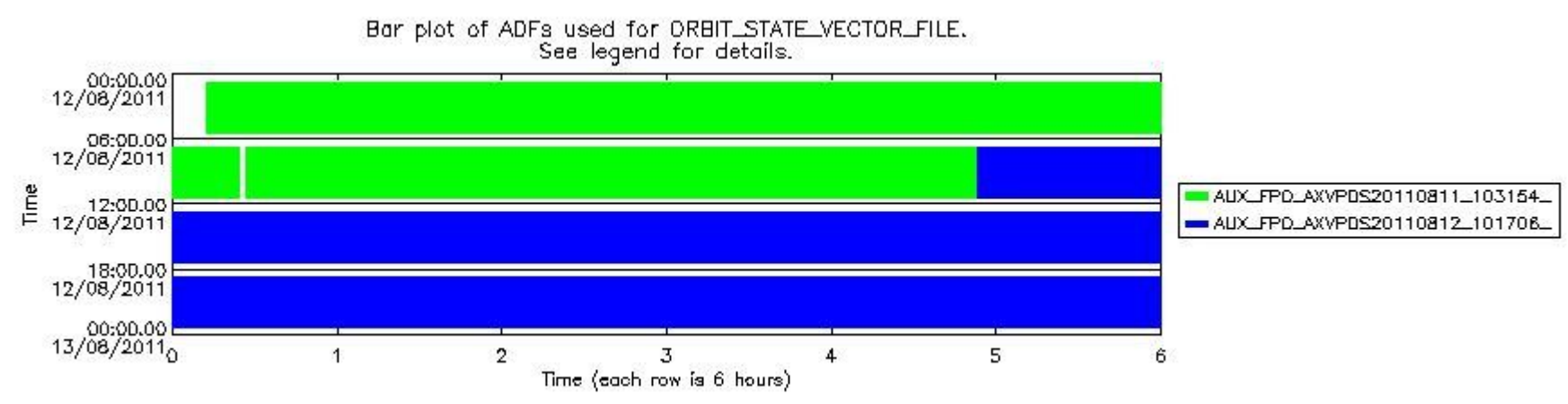
sciamachy_daily_report_level0_KSPT_L0_4504_N_20110812_8.PNG
