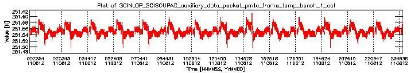
sciamachy_daily_report_level0_KSPT_L0_4504_N_20110812_0.PNG
