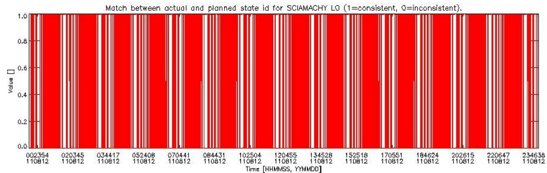
sciamachy_daily_report_level0_KSPT_L0_4504_N_20110812_5.PNG
