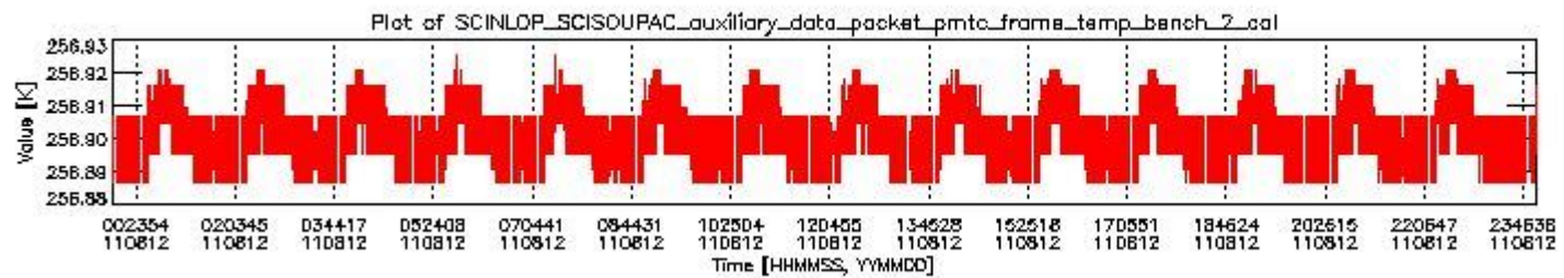
sciamachy_daily_report_level0_KSPT_L0_4504_N_20110812_1.PNG
