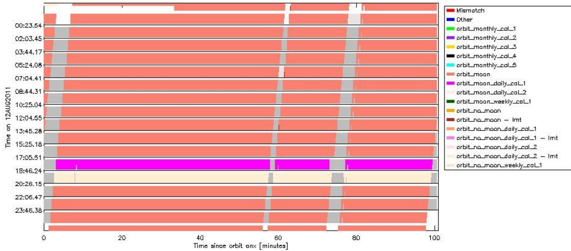
sciamachy_daily_report_level0_KSPT_L0_4504_N_20110812_6.PNG
