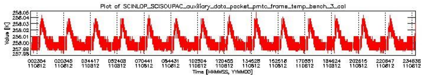
sciamachy_daily_report_level0_KSPT_L0_4504_N_20110812_2.PNG
