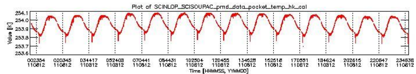
sciamachy_daily_report_level0_KSPT_L0_4504_N_20110812_3.PNG
