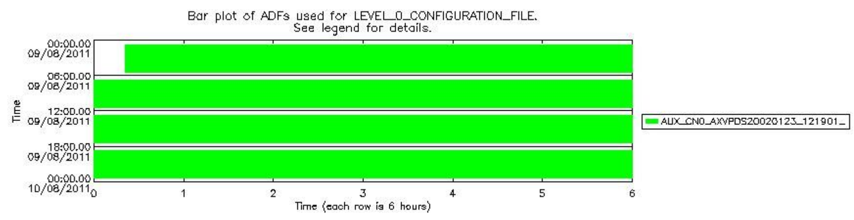
sciamachy_daily_report_level0_KSPT_L0_4504_N_20110809_7.PNG
