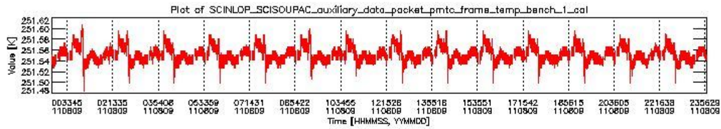
sciamachy_daily_report_level0_KSPT_L0_4504_N_20110809_0.PNG
