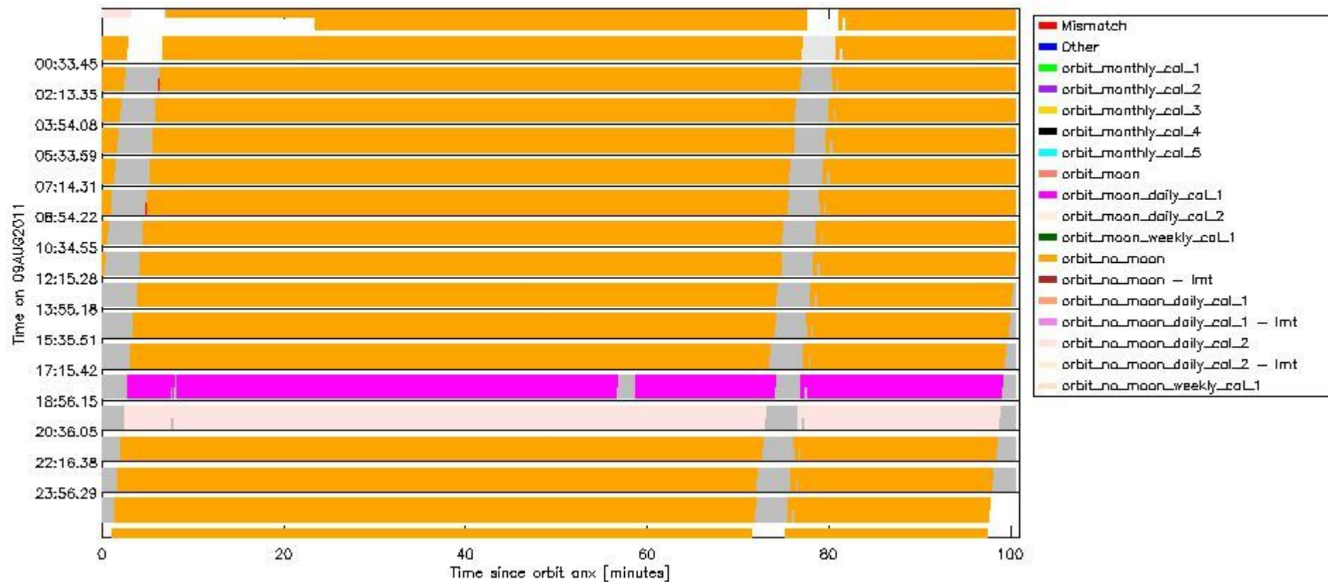
sciamachy_daily_report_level0_KSPT_L0_4504_N_20110809_6.PNG
