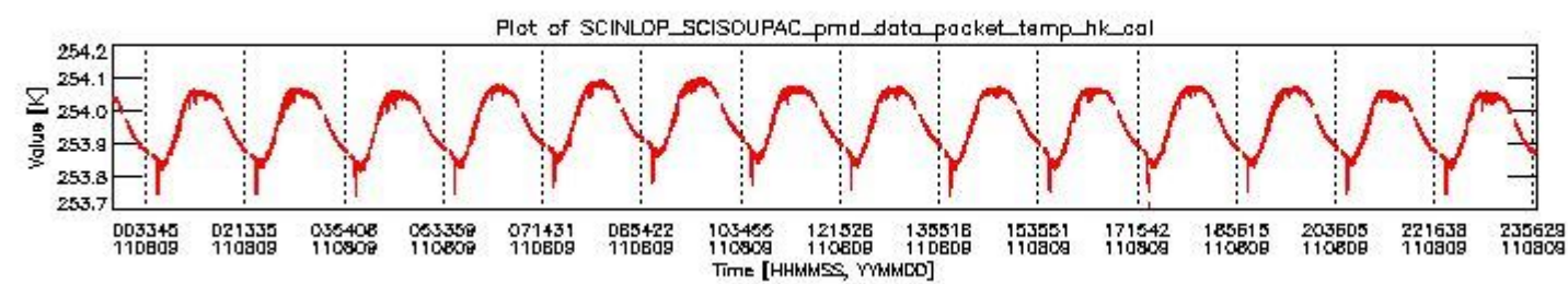
sciamachy_daily_report_level0_KSPT_L0_4504_N_20110809_3.PNG
