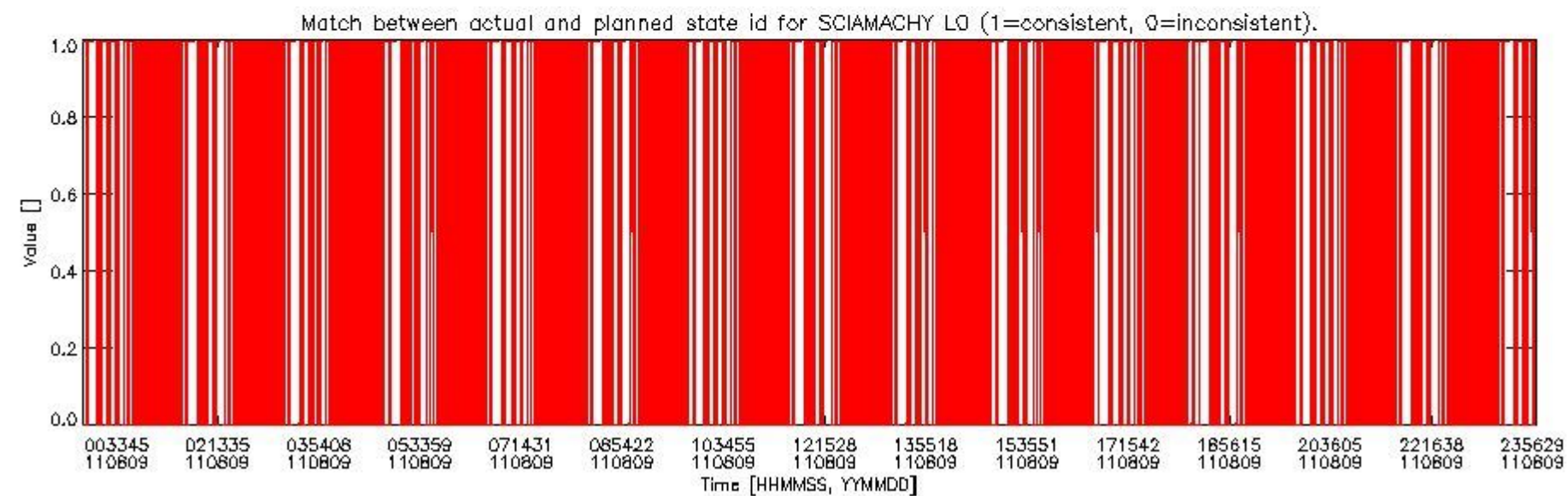
sciamachy_daily_report_level0_KSPT_L0_4504_N_20110809_5.PNG
