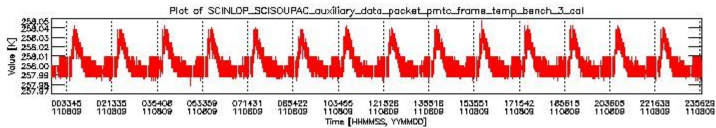
sciamachy_daily_report_level0_KSPT_L0_4504_N_20110809_2.PNG
