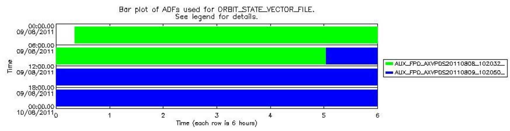
sciamachy_daily_report_level0_KSPT_L0_4504_N_20110809_8.PNG
