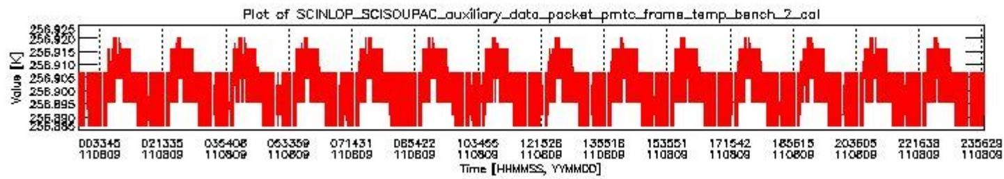
sciamachy_daily_report_level0_KSPT_L0_4504_N_20110809_1.PNG
