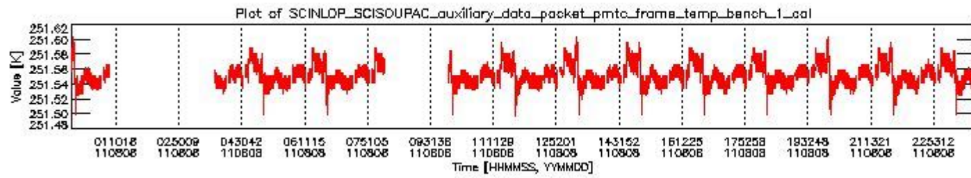
sciamachy_daily_report_level0_KSPT_L0_4504_N_20110808_0.PNG
