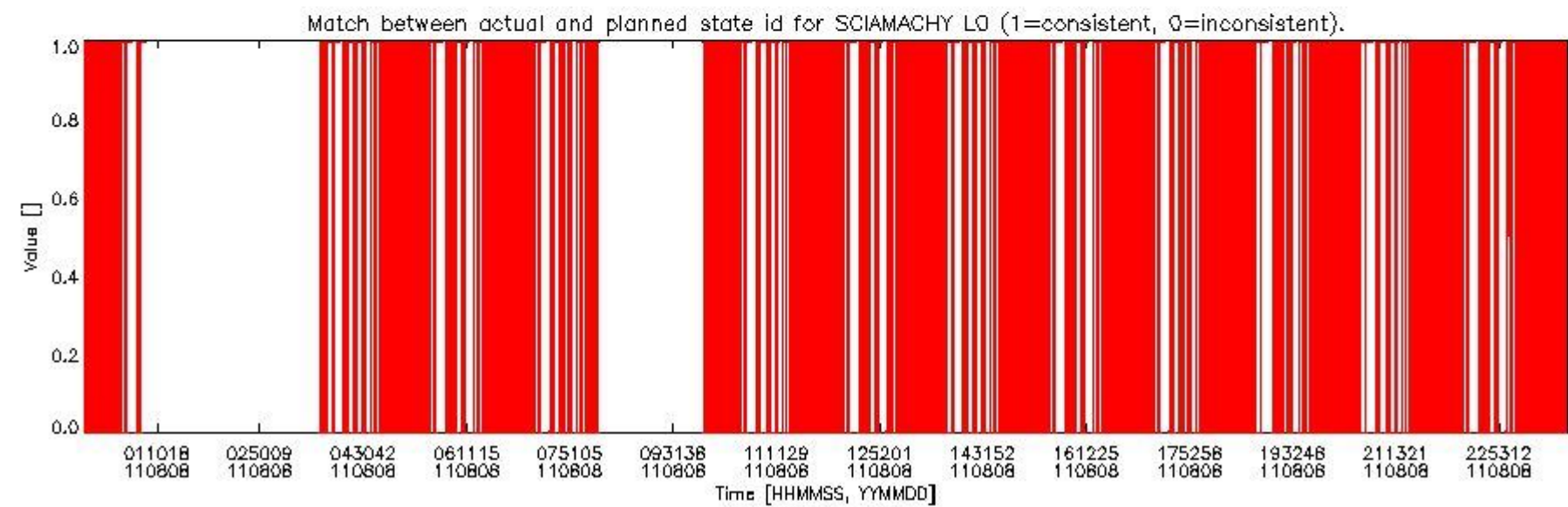
sciamachy_daily_report_level0_KSPT_L0_4504_N_20110808_5.PNG
