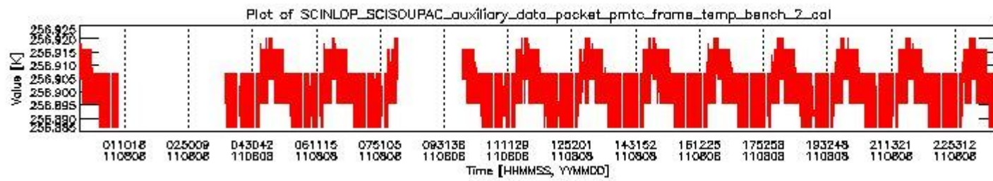
sciamachy_daily_report_level0_KSPT_L0_4504_N_20110808_1.PNG
