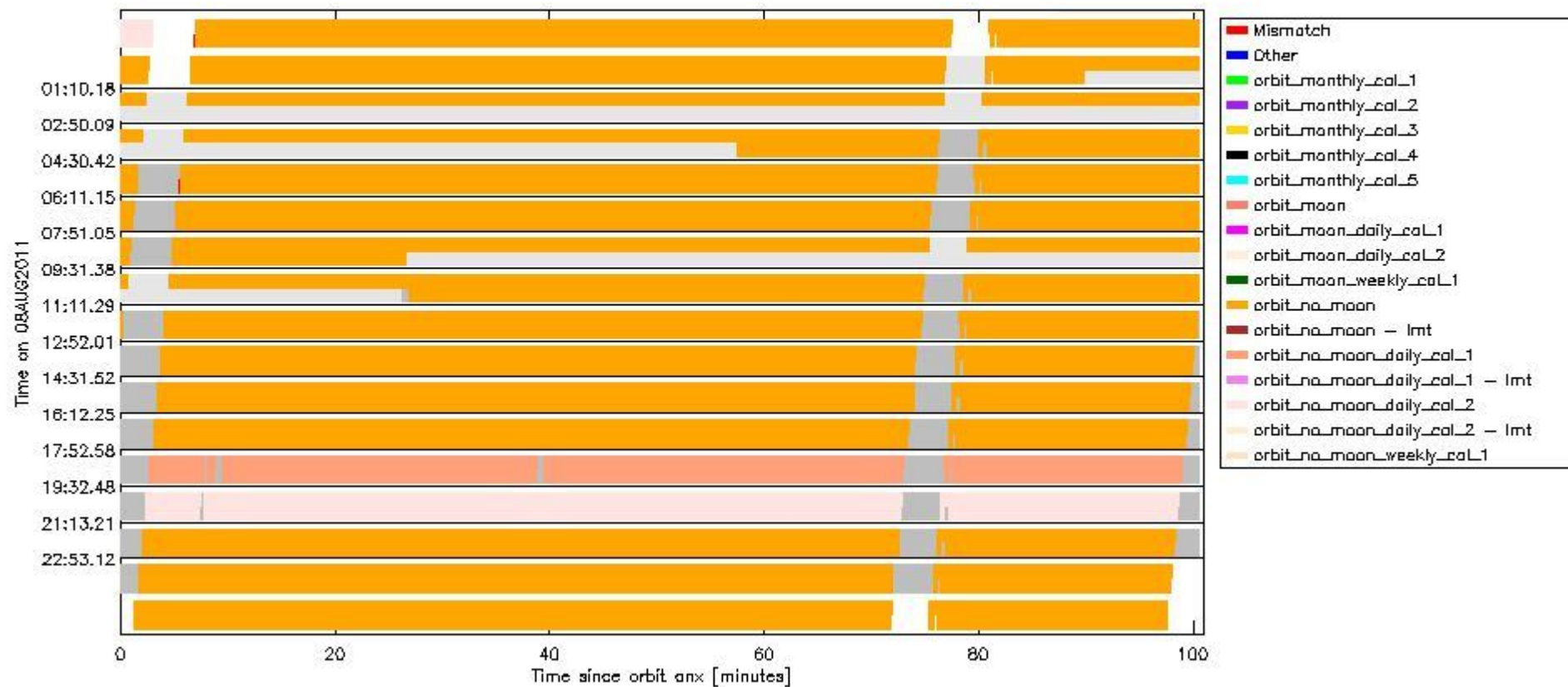
sciamachy_daily_report_level0_KSPT_L0_4504_N_20110808_6.PNG
