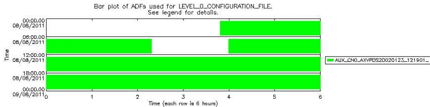
sciamachy_daily_report_level0_KSPT_L0_4504_N_20110808_7.PNG
