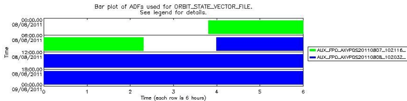
sciamachy_daily_report_level0_KSPT_L0_4504_N_20110808_8.PNG
