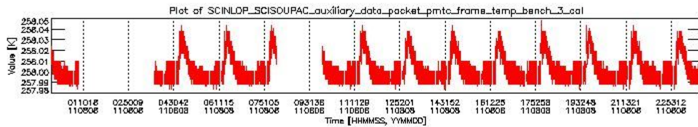
sciamachy_daily_report_level0_KSPT_L0_4504_N_20110808_2.PNG
