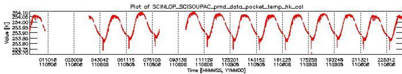
sciamachy_daily_report_level0_KSPT_L0_4504_N_20110808_3.PNG
