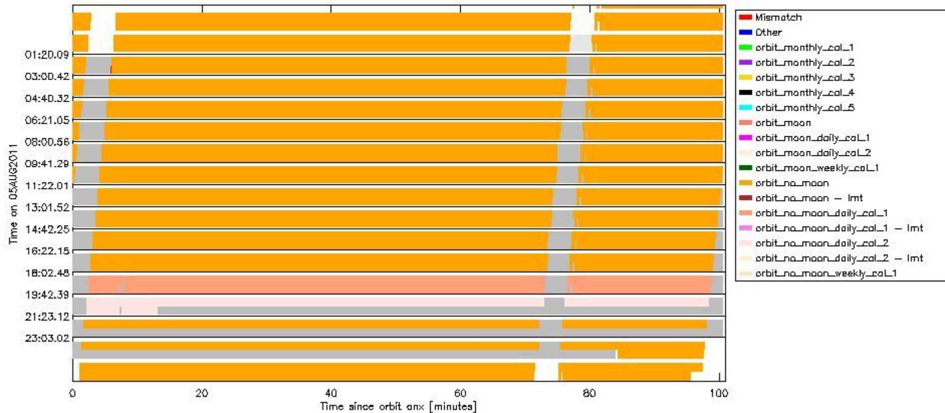
sciamachy_daily_report_level0_KSPT_L0_4504_N_20110805_6.PNG
