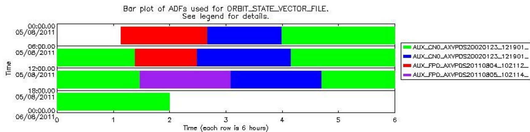
sciamachy_daily_report_level0_KSPT_L0_4504_N_20110805_8.PNG
