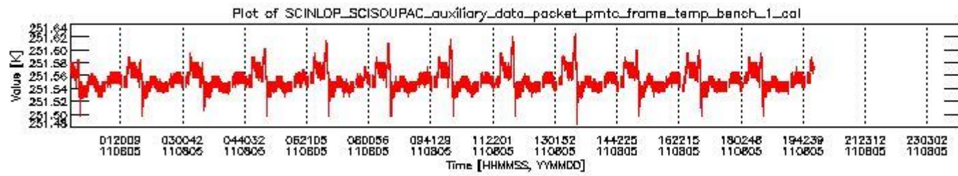
sciamachy_daily_report_level0_KSPT_L0_4504_N_20110805_0.PNG
