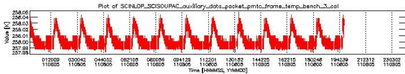
sciamachy_daily_report_level0_KSPT_L0_4504_N_20110805_2.PNG
