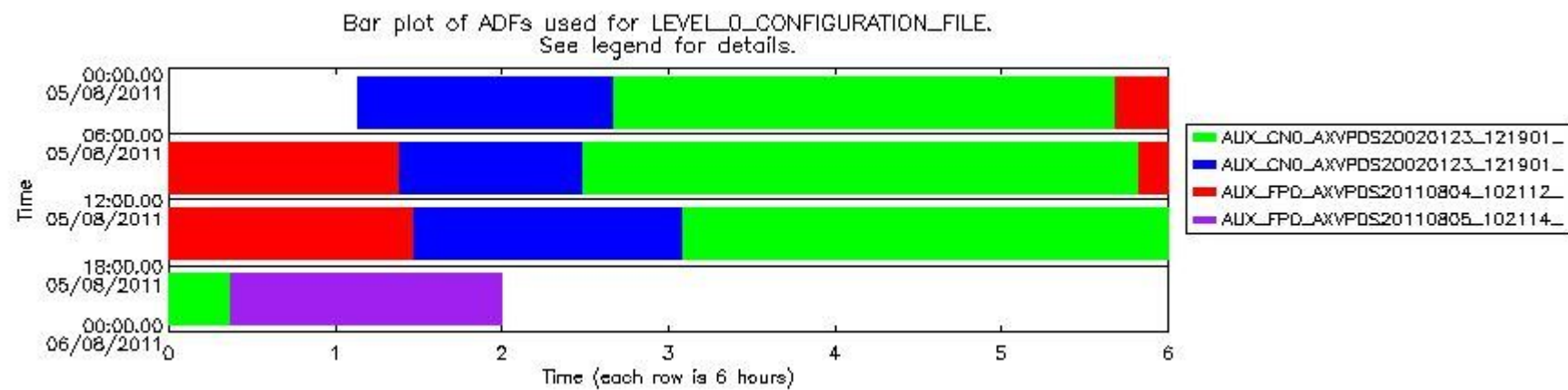
sciamachy_daily_report_level0_KSPT_L0_4504_N_20110805_7.PNG
