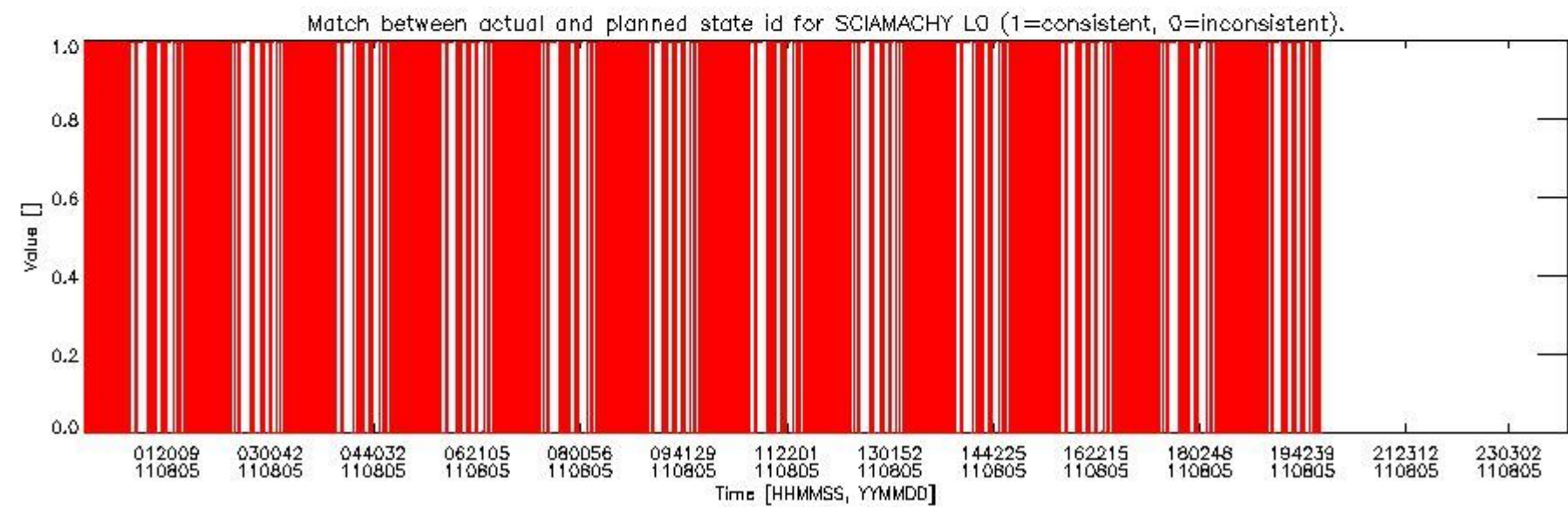
sciamachy_daily_report_level0_KSPT_L0_4504_N_20110805_5.PNG
