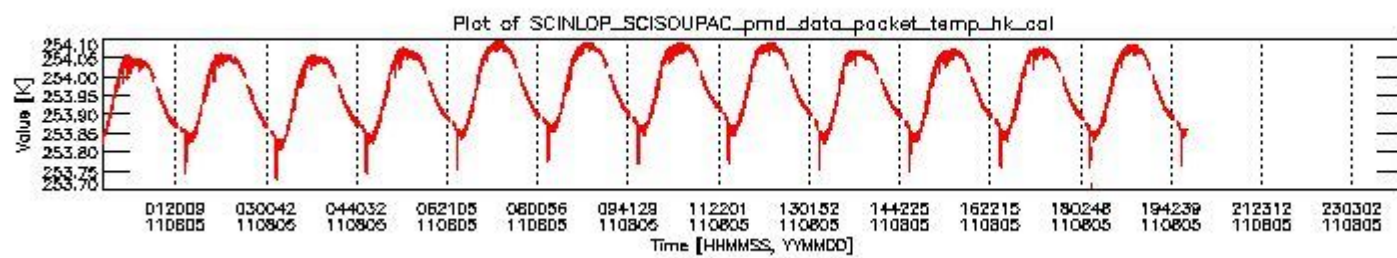
sciamachy_daily_report_level0_KSPT_L0_4504_N_20110805_3.PNG
