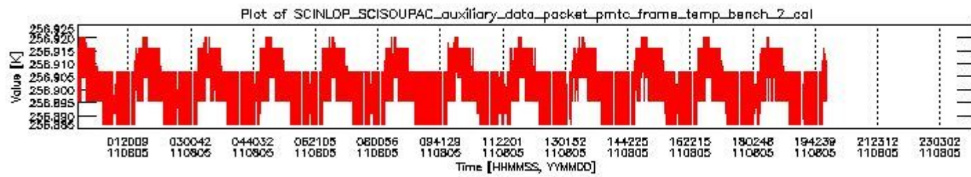
sciamachy_daily_report_level0_KSPT_L0_4504_N_20110805_1.PNG
