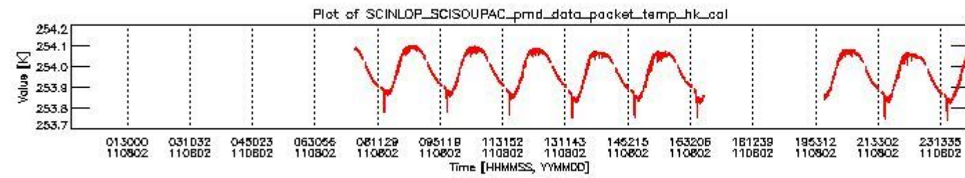
sciamachy_daily_report_level0_KSPT_L0_4504_N_20110802_3.PNG
