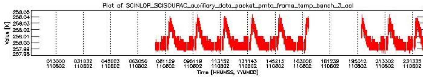
sciamachy_daily_report_level0_KSPT_L0_4504_N_20110802_2.PNG
