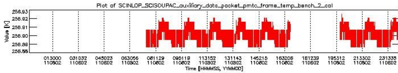
sciamachy_daily_report_level0_KSPT_L0_4504_N_20110802_1.PNG
