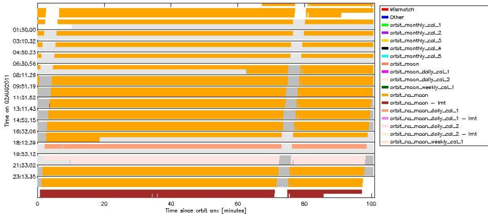
sciamachy_daily_report_level0_KSPT_L0_4504_N_20110802_6.PNG
