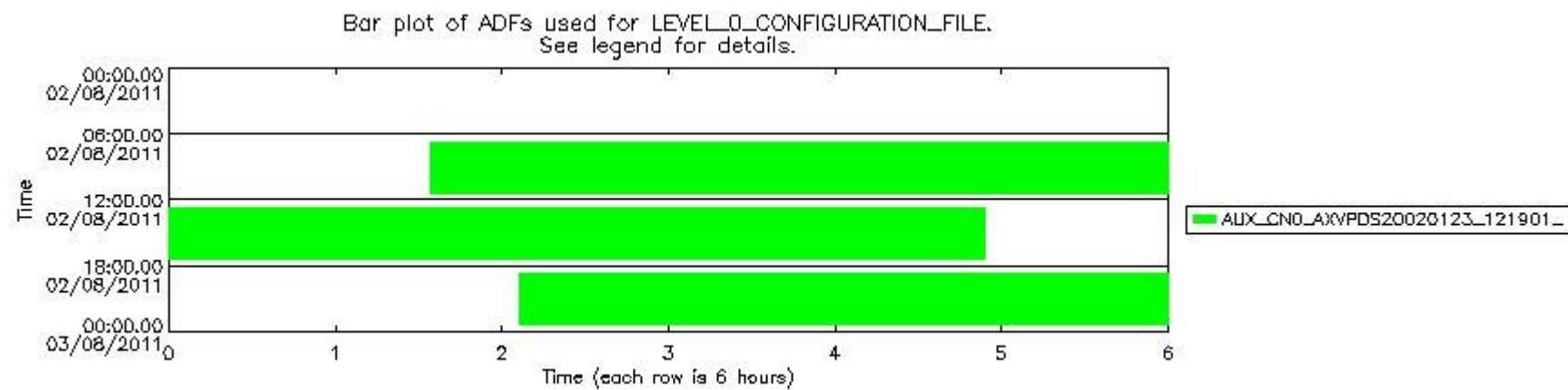
sciamachy_daily_report_level0_KSPT_L0_4504_N_20110802_7.PNG
