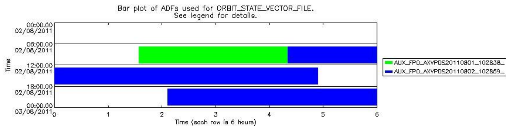
sciamachy_daily_report_level0_KSPT_L0_4504_N_20110802_8.PNG
