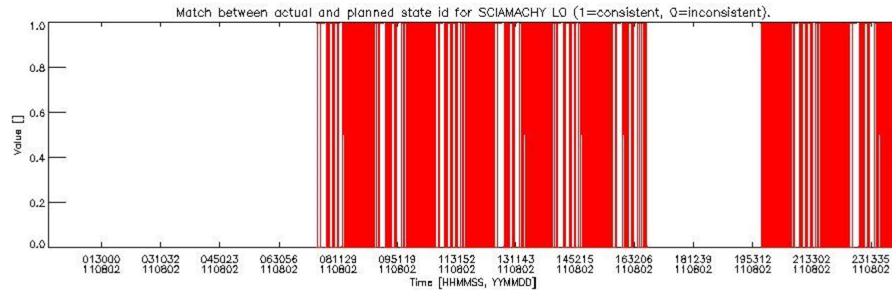
sciamachy_daily_report_level0_KSPT_L0_4504_N_20110802_5.PNG
