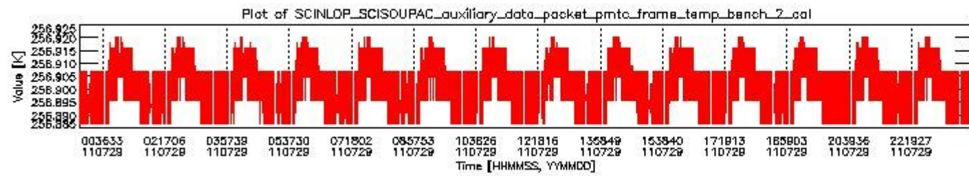
sciamachy_daily_report_level0_KSPT_L0_4504_N_20110729_1.PNG
