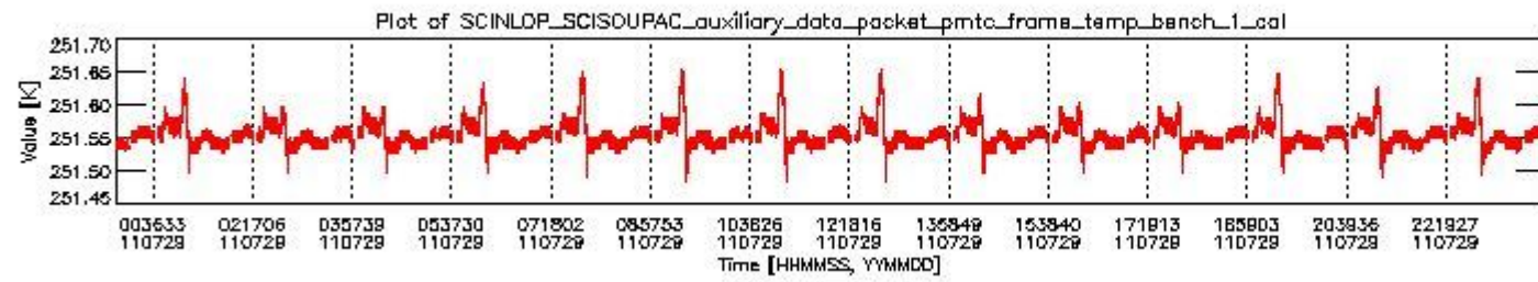
sciamachy_daily_report_level0_KSPT_L0_4504_N_20110729_0.PNG
