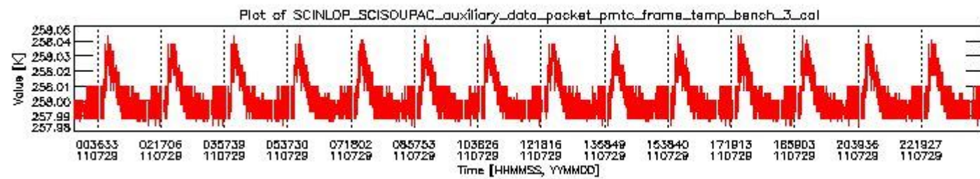
sciamachy_daily_report_level0_KSPT_L0_4504_N_20110729_2.PNG
