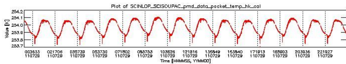
sciamachy_daily_report_level0_KSPT_L0_4504_N_20110729_3.PNG
