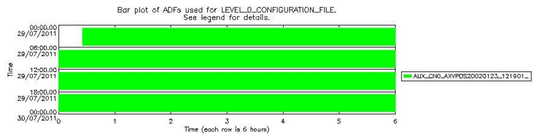
sciamachy_daily_report_level0_KSPT_L0_4504_N_20110729_7.PNG
