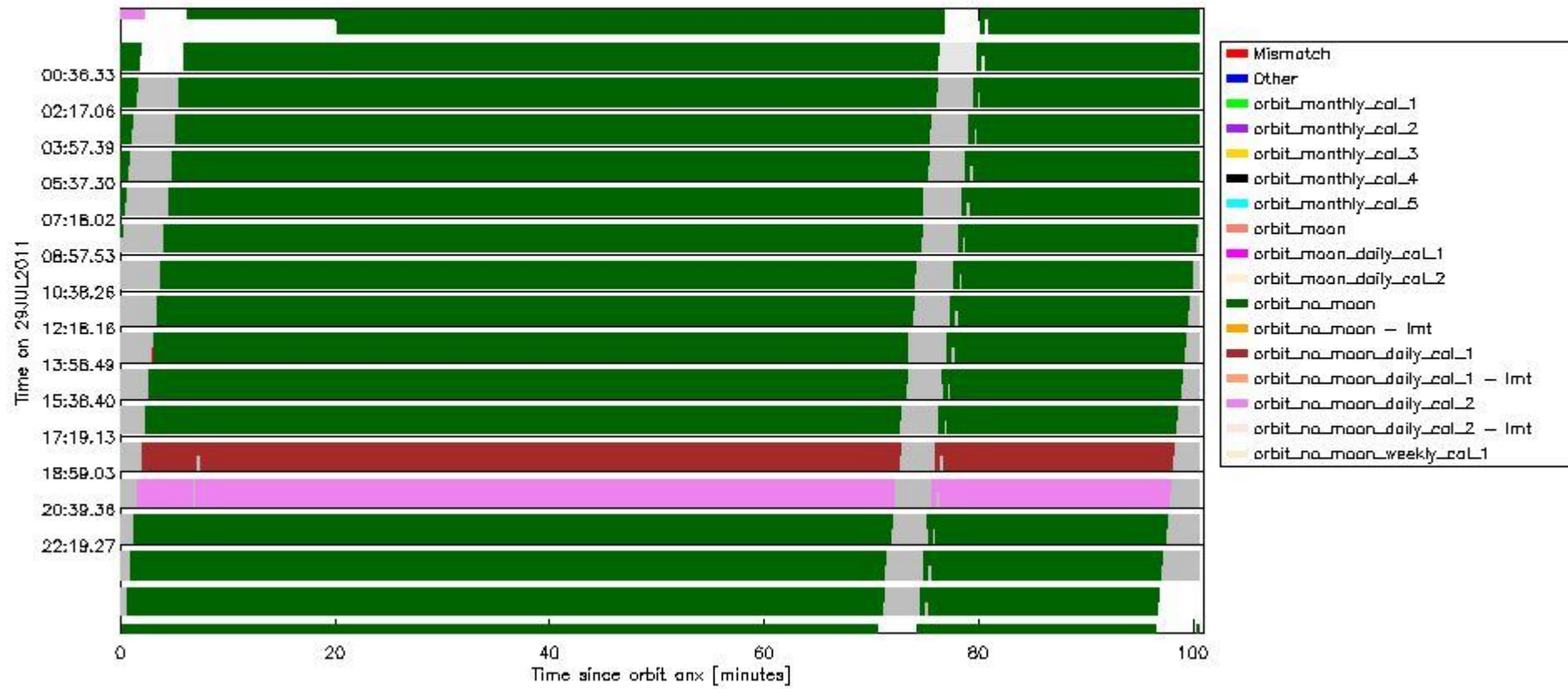
sciamachy_daily_report_level0_KSPT_L0_4504_N_20110729_6.PNG
