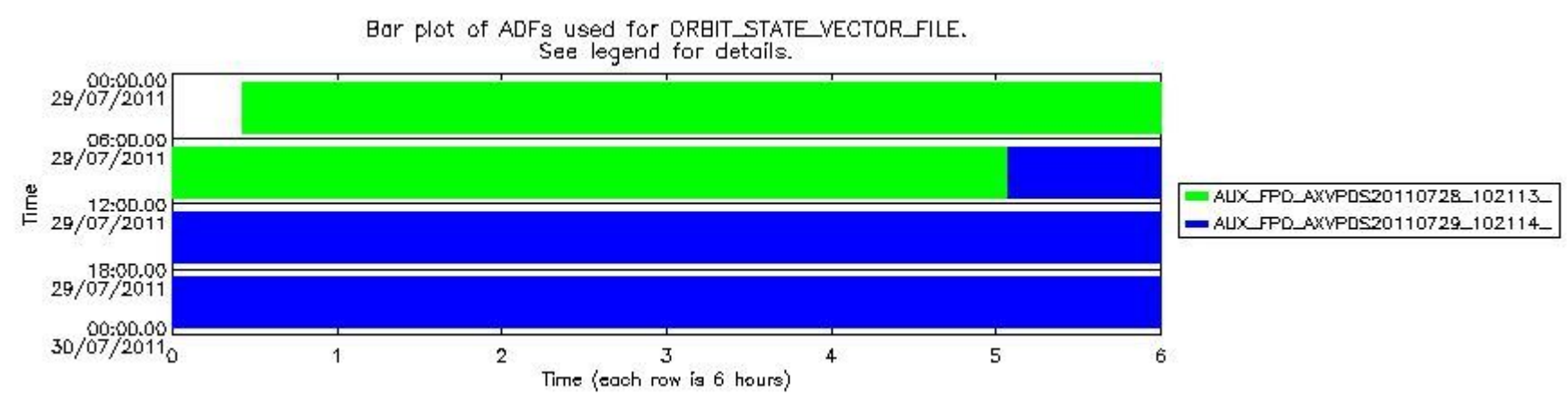
sciamachy_daily_report_level0_KSPT_L0_4504_N_20110729_8.PNG
