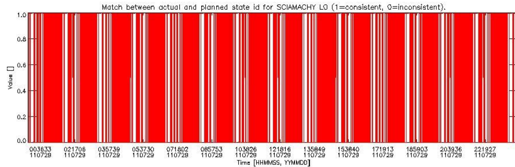
sciamachy_daily_report_level0_KSPT_L0_4504_N_20110729_5.PNG
