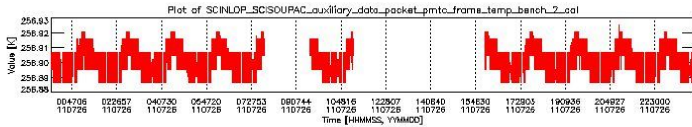
sciamachy_daily_report_level0_KSPT_L0_4504_N_20110726_1.PNG
