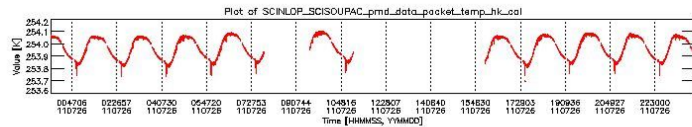
sciamachy_daily_report_level0_KSPT_L0_4504_N_20110726_3.PNG
