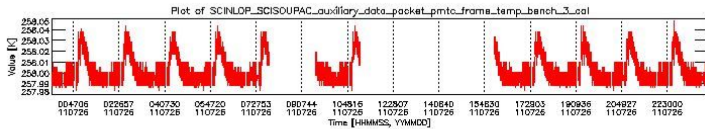
sciamachy_daily_report_level0_KSPT_L0_4504_N_20110726_2.PNG
