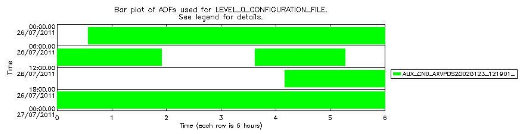
sciamachy_daily_report_level0_KSPT_L0_4504_N_20110726_7.PNG
