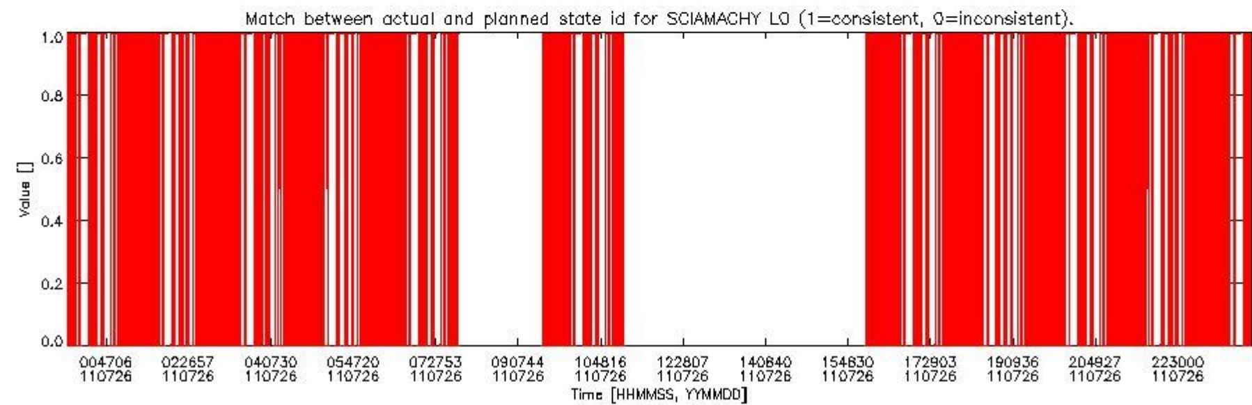
sciamachy_daily_report_level0_KSPT_L0_4504_N_20110726_5.PNG
