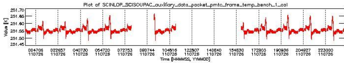
sciamachy_daily_report_level0_KSPT_L0_4504_N_20110726_0.PNG
