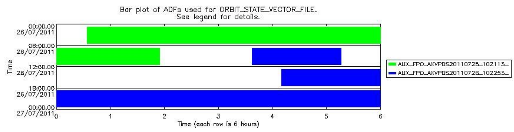
sciamachy_daily_report_level0_KSPT_L0_4504_N_20110726_8.PNG
