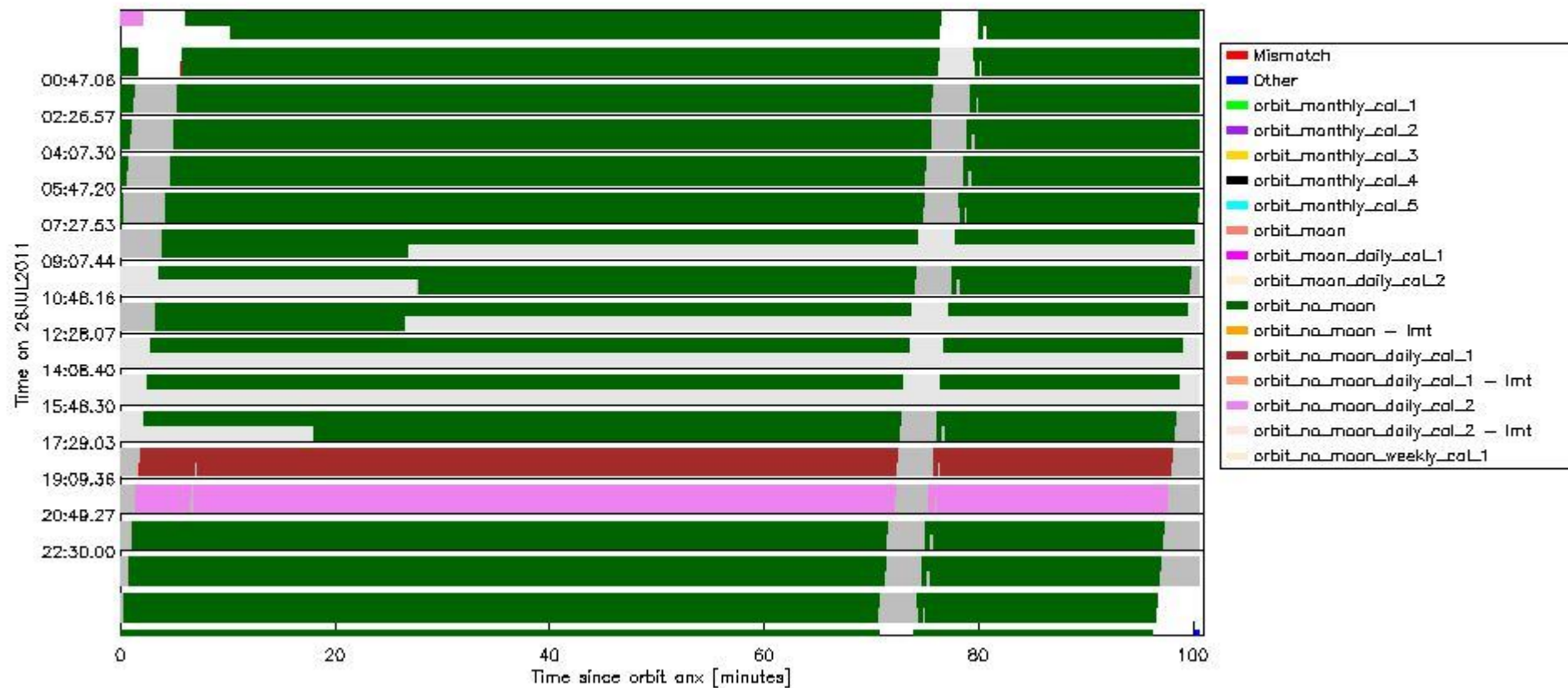
sciamachy_daily_report_level0_KSPT_L0_4504_N_20110726_6.PNG
