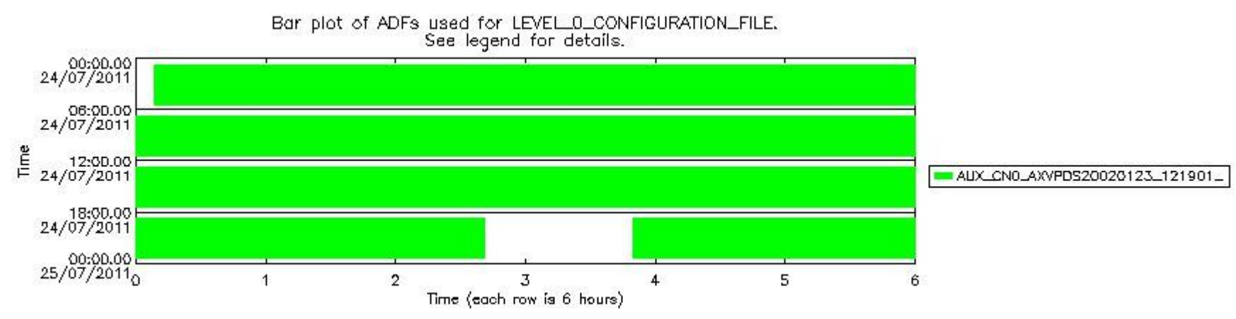
sciamachy_daily_report_level0_KSPT_L0_4504_N_20110724_7.PNG
