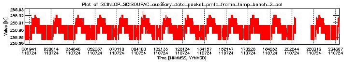
sciamachy_daily_report_level0_KSPT_L0_4504_N_20110724_1.PNG
