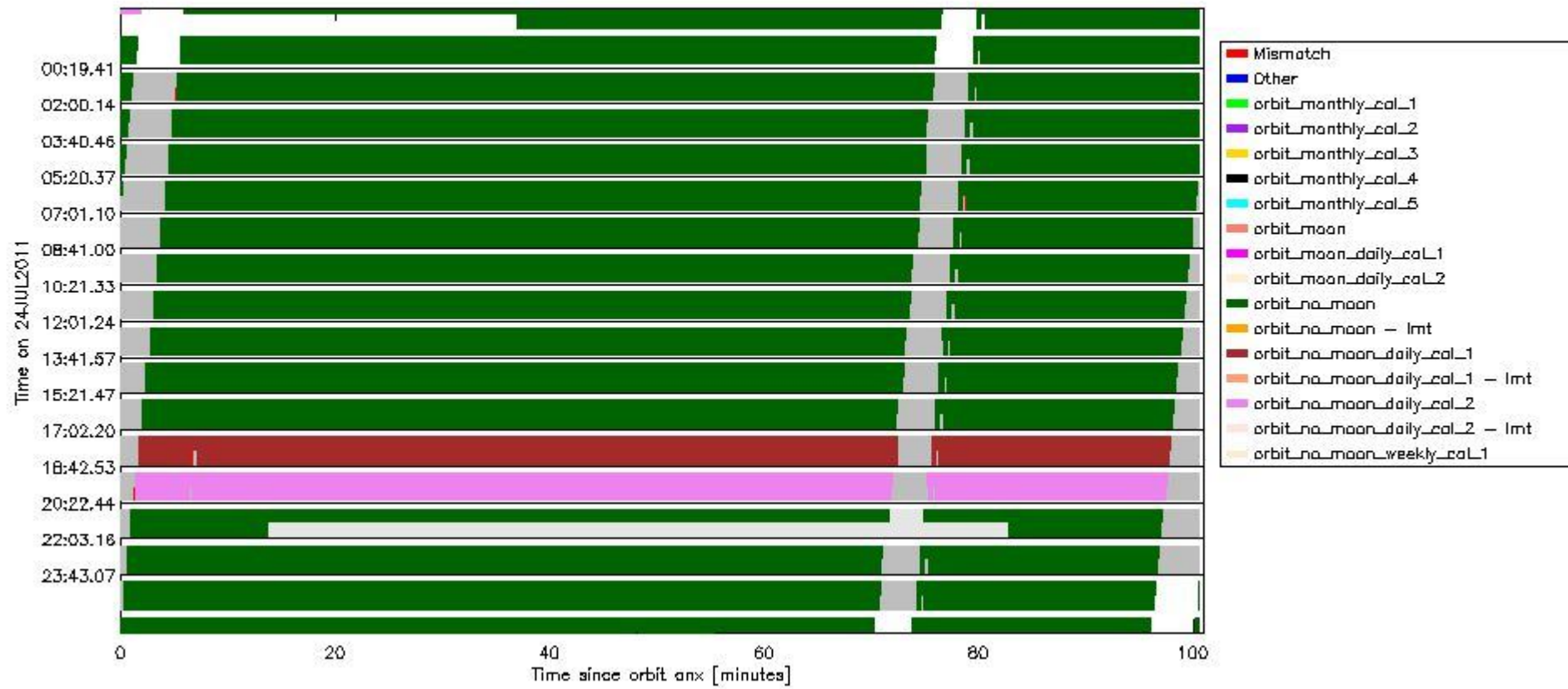
sciamachy_daily_report_level0_KSPT_L0_4504_N_20110724_6.PNG
