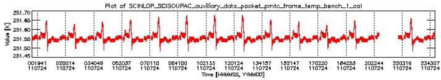
sciamachy_daily_report_level0_KSPT_L0_4504_N_20110724_0.PNG
