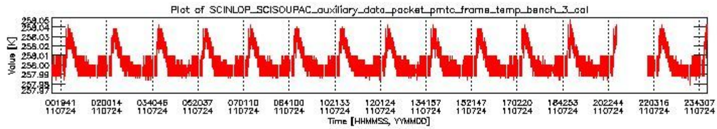
sciamachy_daily_report_level0_KSPT_L0_4504_N_20110724_2.PNG
