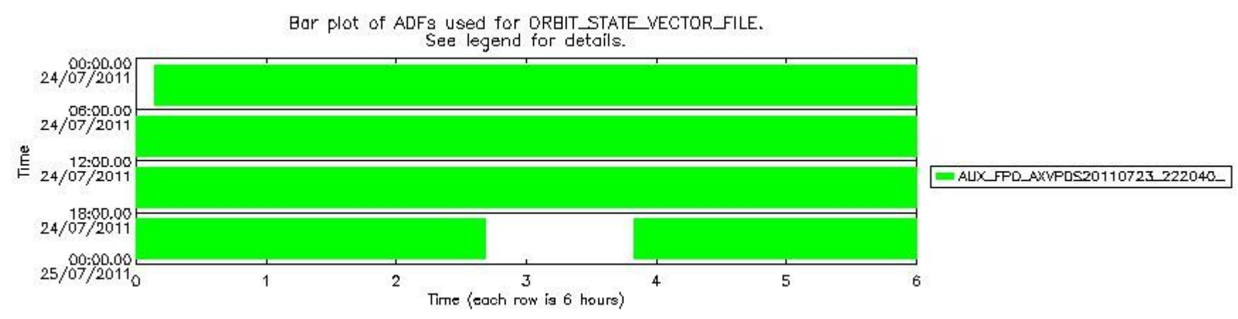
sciamachy_daily_report_level0_KSPT_L0_4504_N_20110724_8.PNG
