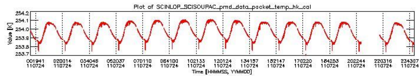
sciamachy_daily_report_level0_KSPT_L0_4504_N_20110724_3.PNG
