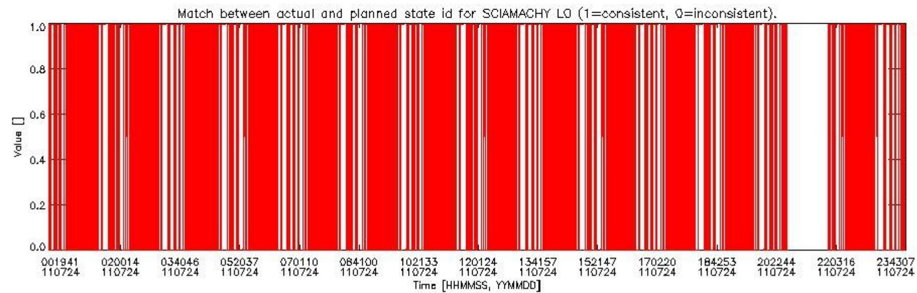
sciamachy_daily_report_level0_KSPT_L0_4504_N_20110724_5.PNG
