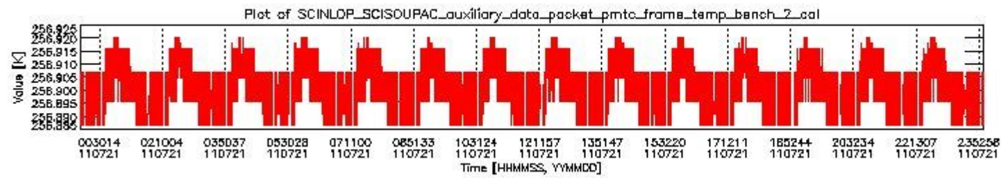
sciamachy_daily_report_level0_KSPT_L0_4504_N_20110721_1.PNG
