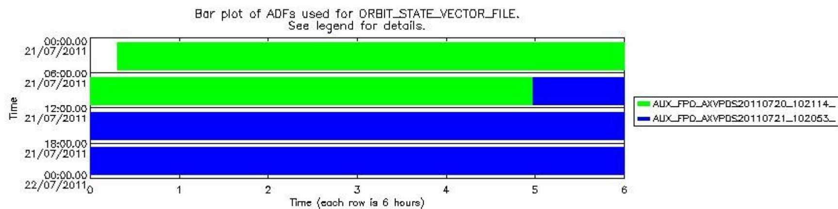
sciamachy_daily_report_level0_KSPT_L0_4504_N_20110721_8.PNG
