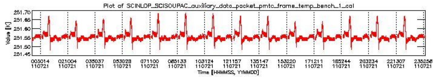
sciamachy_daily_report_level0_KSPT_L0_4504_N_20110721_0.PNG
