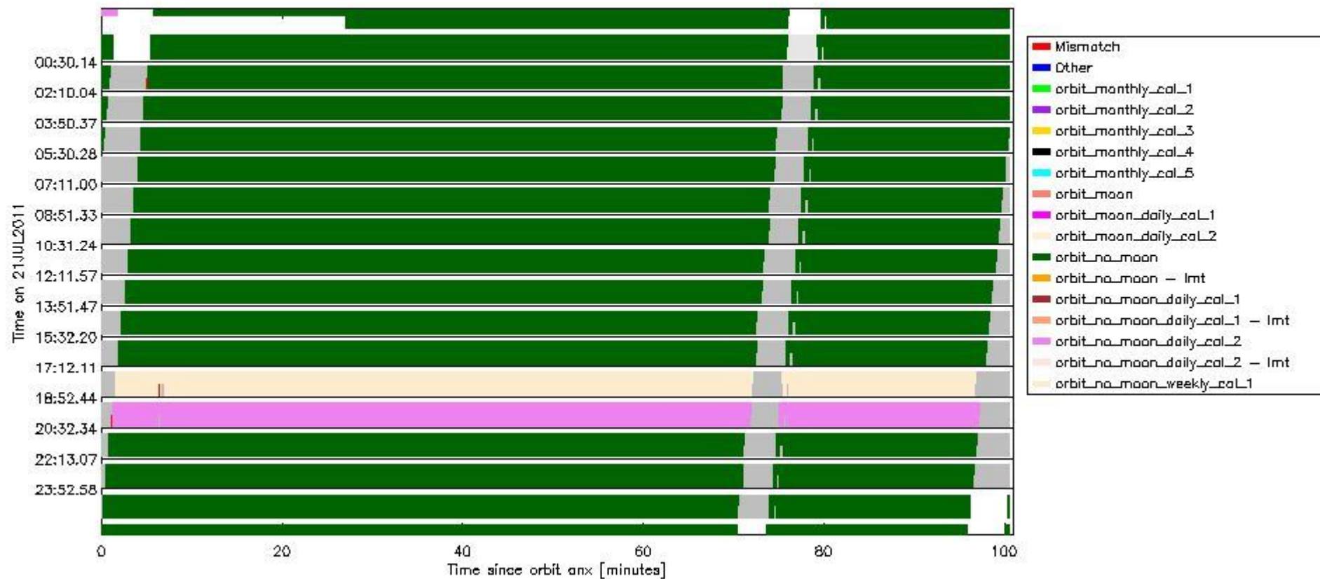
sciamachy_daily_report_level0_KSPT_L0_4504_N_20110721_6.PNG
