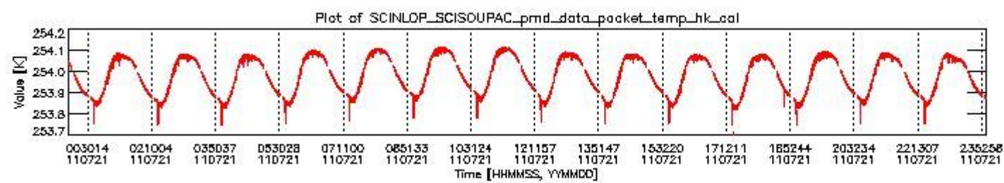
sciamachy_daily_report_level0_KSPT_L0_4504_N_20110721_3.PNG
