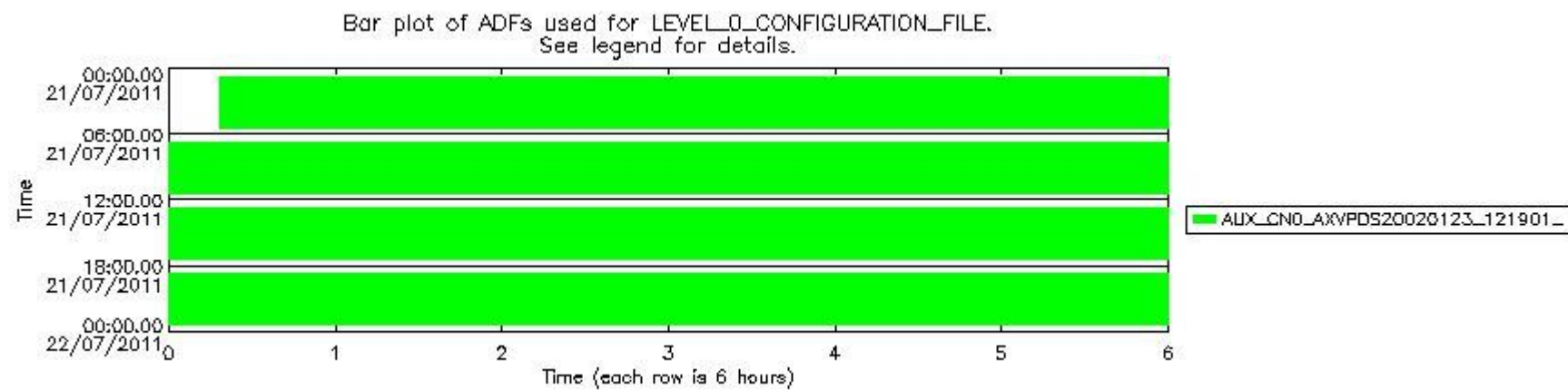
sciamachy_daily_report_level0_KSPT_L0_4504_N_20110721_7.PNG
