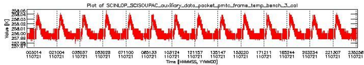
sciamachy_daily_report_level0_KSPT_L0_4504_N_20110721_2.PNG
