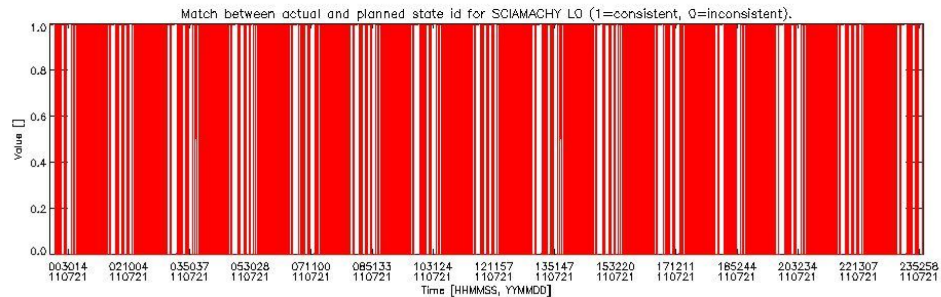
sciamachy_daily_report_level0_KSPT_L0_4504_N_20110721_5.PNG
