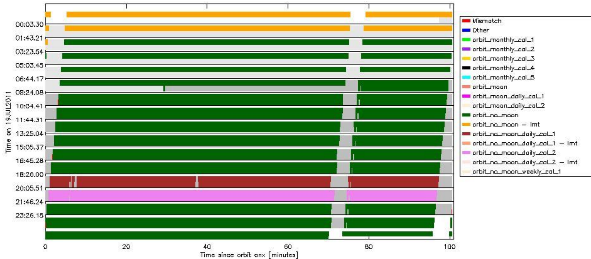
sciamachy_daily_report_level0_KSPT_L0_4504_N_20110719_6.PNG
