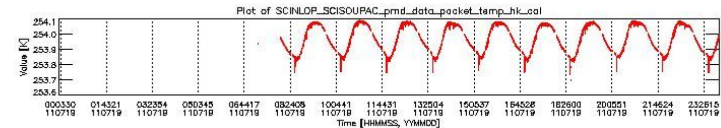
sciamachy_daily_report_level0_KSPT_L0_4504_N_20110719_3.PNG
