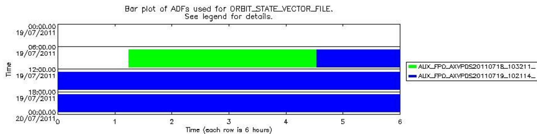
sciamachy_daily_report_level0_KSPT_L0_4504_N_20110719_8.PNG
