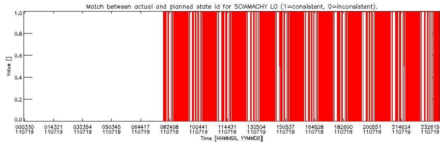
sciamachy_daily_report_level0_KSPT_L0_4504_N_20110719_5.PNG
