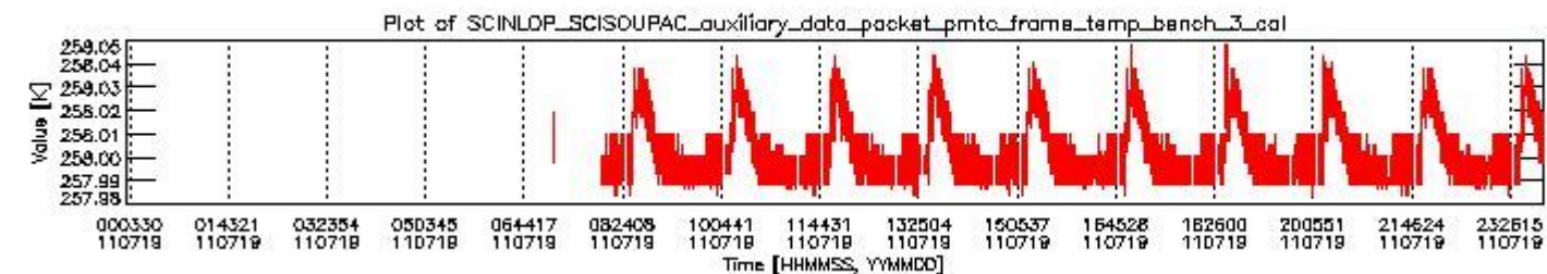
sciamachy_daily_report_level0_KSPT_L0_4504_N_20110719_2.PNG
