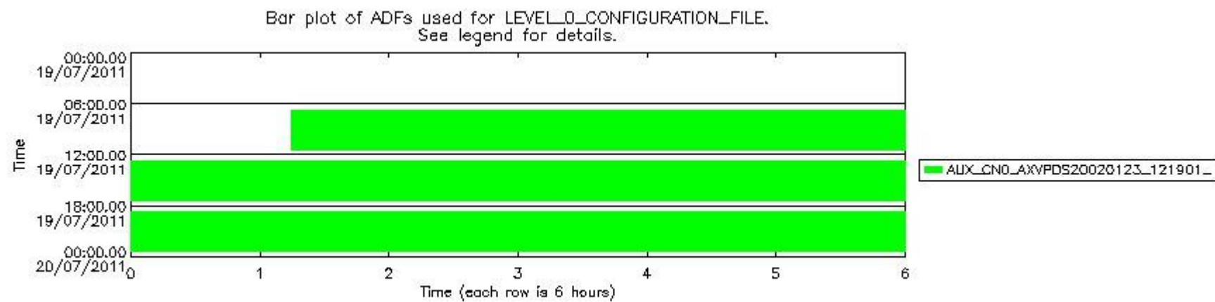
sciamachy_daily_report_level0_KSPT_L0_4504_N_20110719_7.PNG
