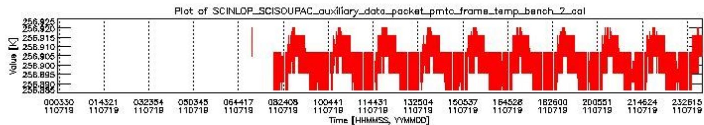
sciamachy_daily_report_level0_KSPT_L0_4504_N_20110719_1.PNG
