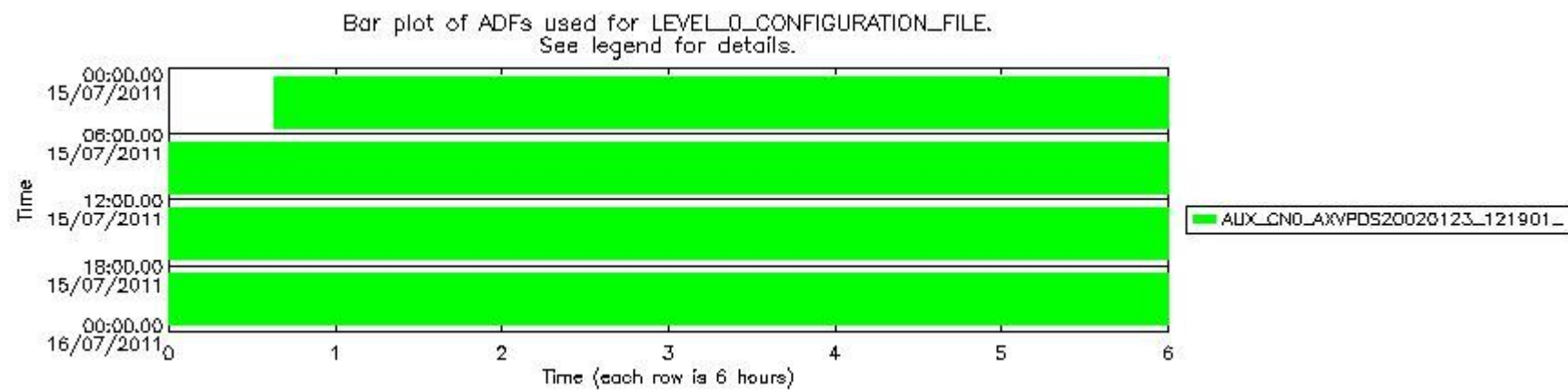
sciamachy_daily_report_level0_KSPT_L0_4504_N_20110715_7.PNG
