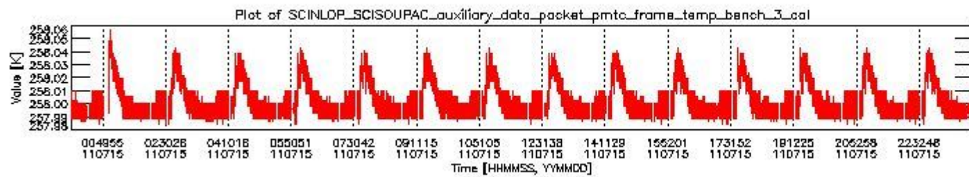
sciamachy_daily_report_level0_KSPT_L0_4504_N_20110715_2.PNG
