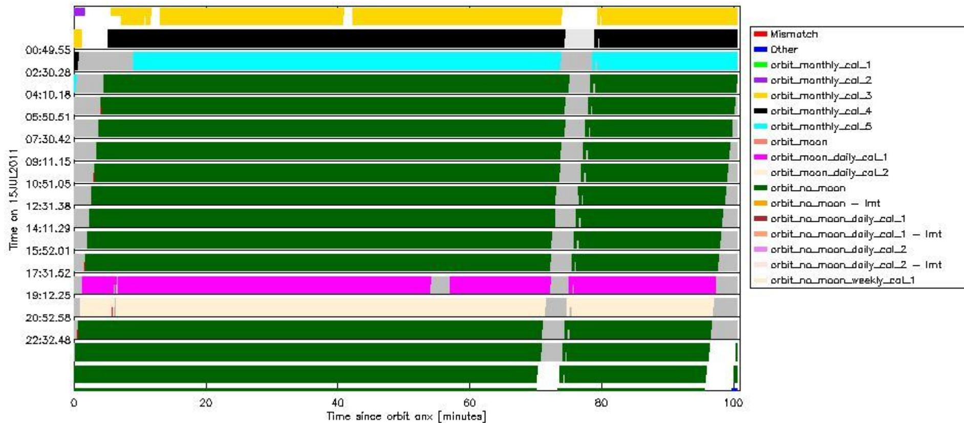
sciamachy_daily_report_level0_KSPT_L0_4504_N_20110715_6.PNG
