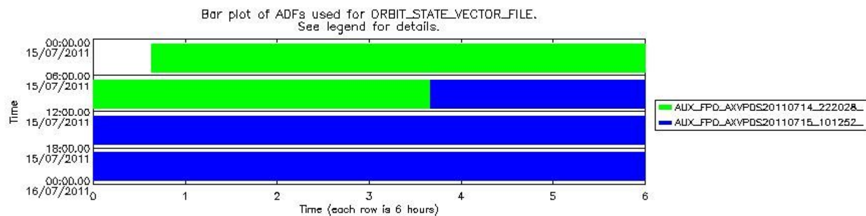
sciamachy_daily_report_level0_KSPT_L0_4504_N_20110715_8.PNG
