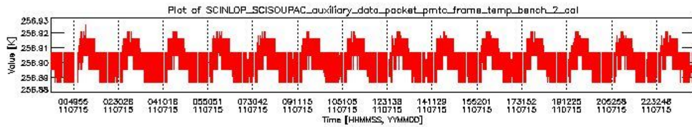
sciamachy_daily_report_level0_KSPT_L0_4504_N_20110715_1.PNG
