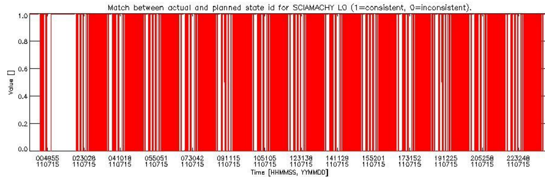
sciamachy_daily_report_level0_KSPT_L0_4504_N_20110715_5.PNG
