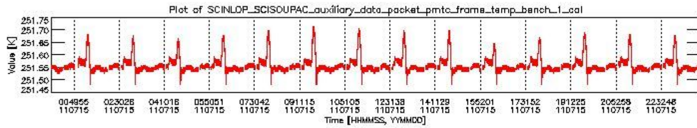
sciamachy_daily_report_level0_KSPT_L0_4504_N_20110715_0.PNG
