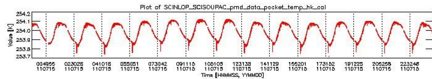
sciamachy_daily_report_level0_KSPT_L0_4504_N_20110715_3.PNG
