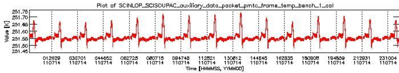
sciamachy_daily_report_level0_KSPT_L0_4504_N_20110714_0.PNG
