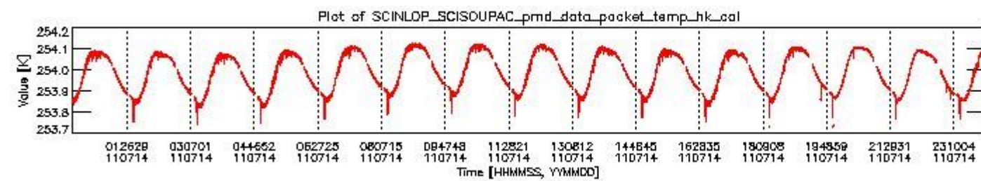
sciamachy_daily_report_level0_KSPT_L0_4504_N_20110714_3.PNG
