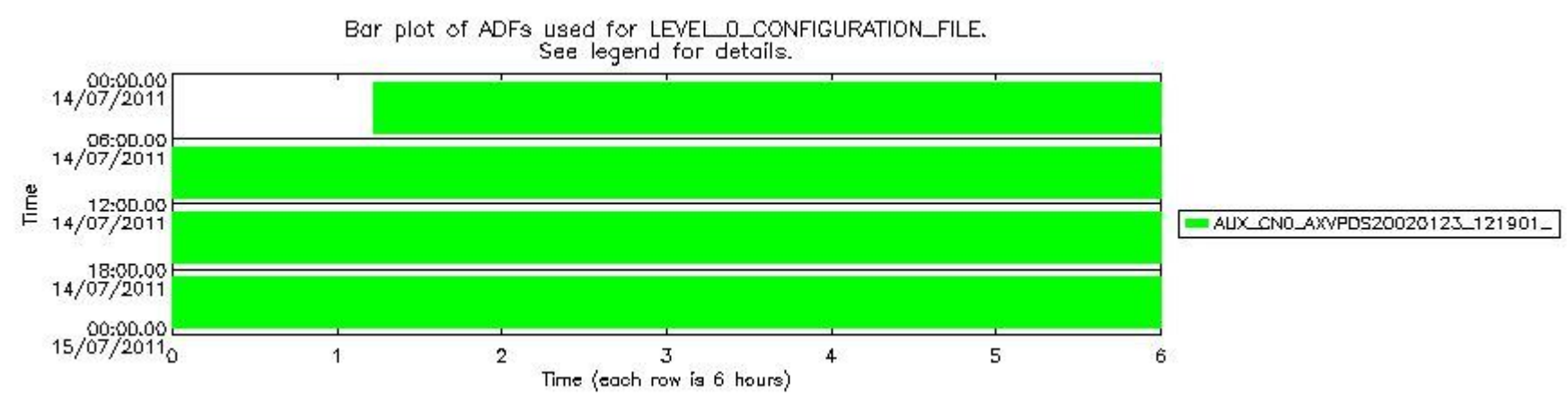
sciamachy_daily_report_level0_KSPT_L0_4504_N_20110714_7.PNG
