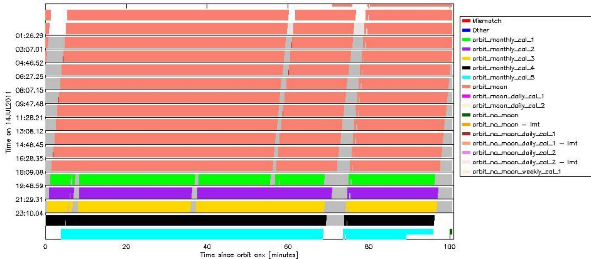
sciamachy_daily_report_level0_KSPT_L0_4504_N_20110714_6.PNG
