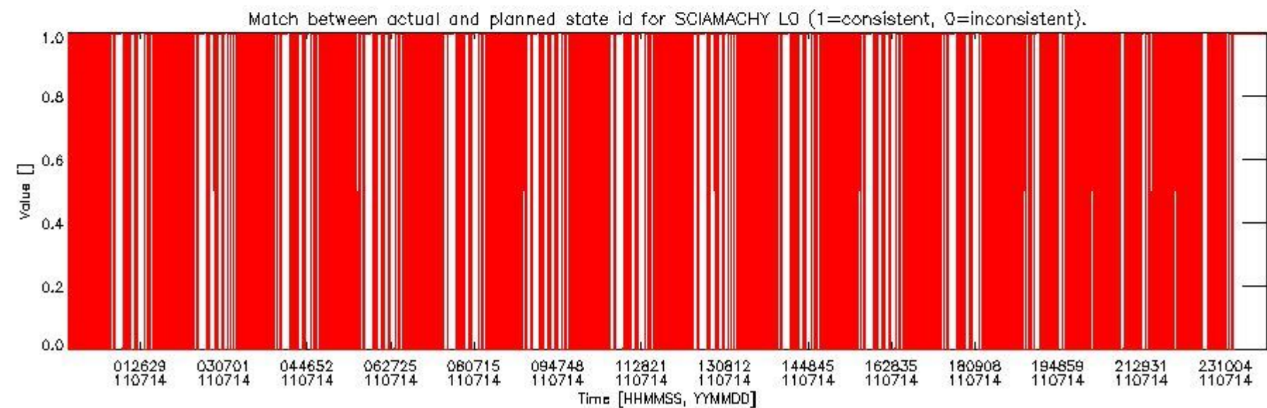
sciamachy_daily_report_level0_KSPT_L0_4504_N_20110714_5.PNG
