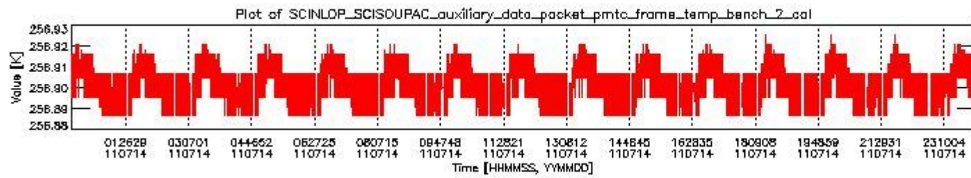
sciamachy_daily_report_level0_KSPT_L0_4504_N_20110714_1.PNG
