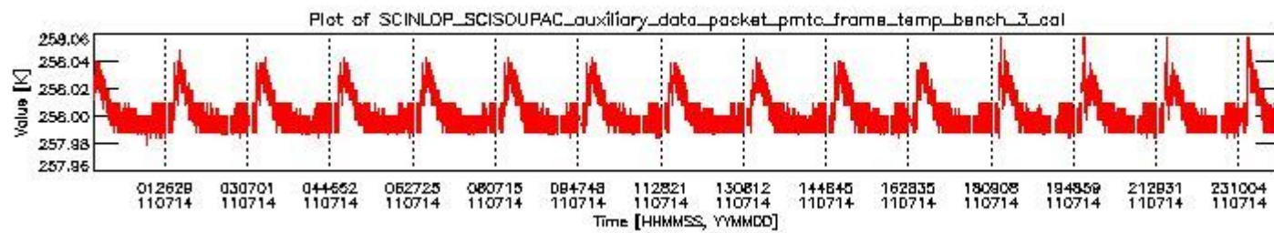
sciamachy_daily_report_level0_KSPT_L0_4504_N_20110714_2.PNG
