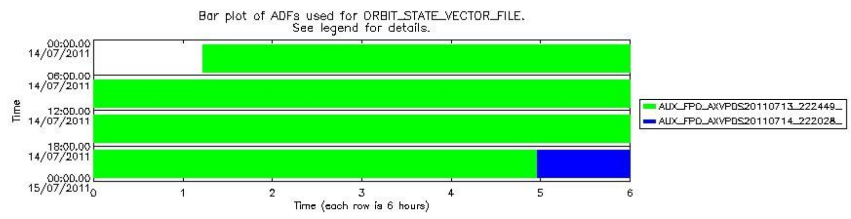
sciamachy_daily_report_level0_KSPT_L0_4504_N_20110714_8.PNG
