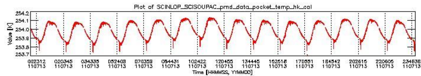
sciamachy_daily_report_level0_KSPT_L0_4504_N_20110713_3.PNG
