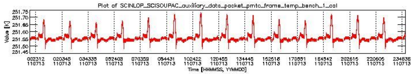
sciamachy_daily_report_level0_KSPT_L0_4504_N_20110713_0.PNG
