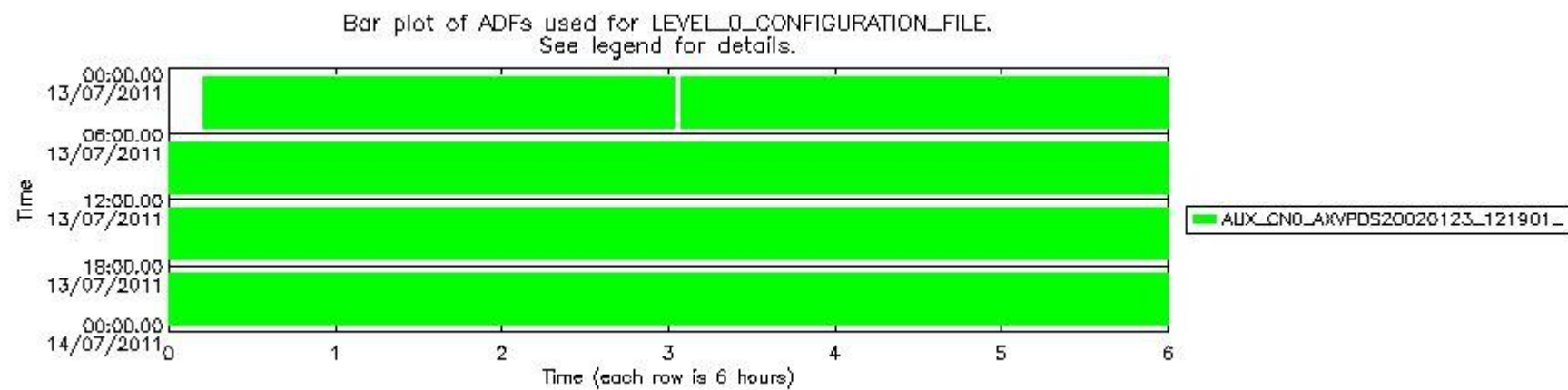
sciamachy_daily_report_level0_KSPT_L0_4504_N_20110713_7.PNG
