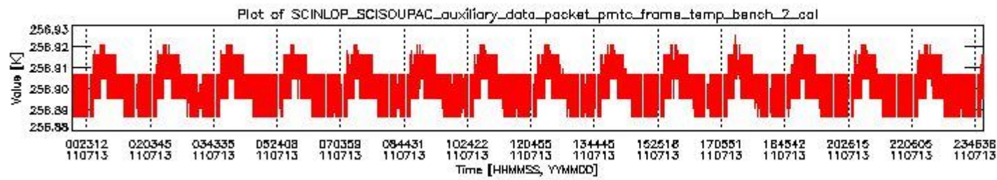
sciamachy_daily_report_level0_KSPT_L0_4504_N_20110713_1.PNG
