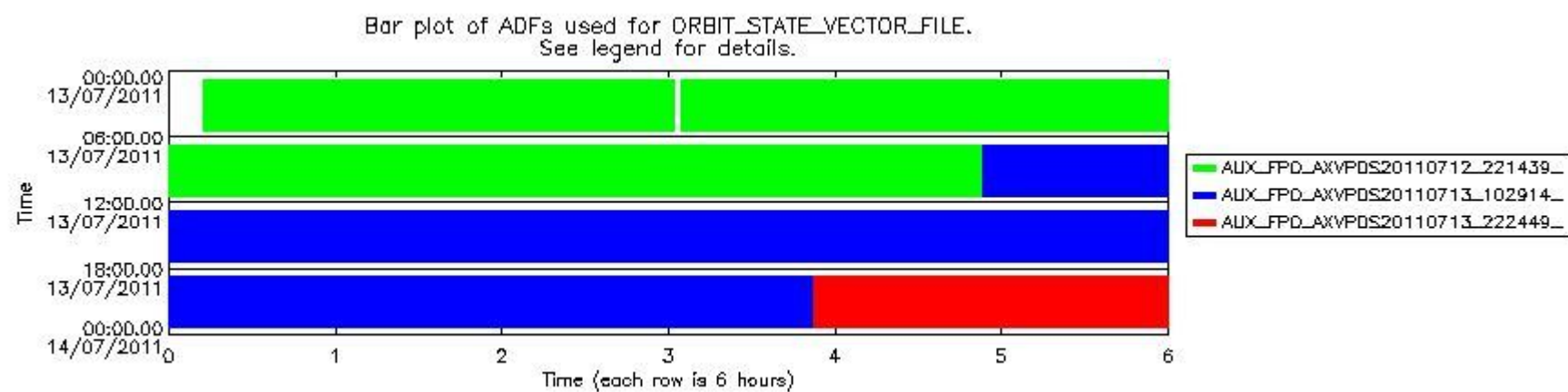
sciamachy_daily_report_level0_KSPT_L0_4504_N_20110713_8.PNG
