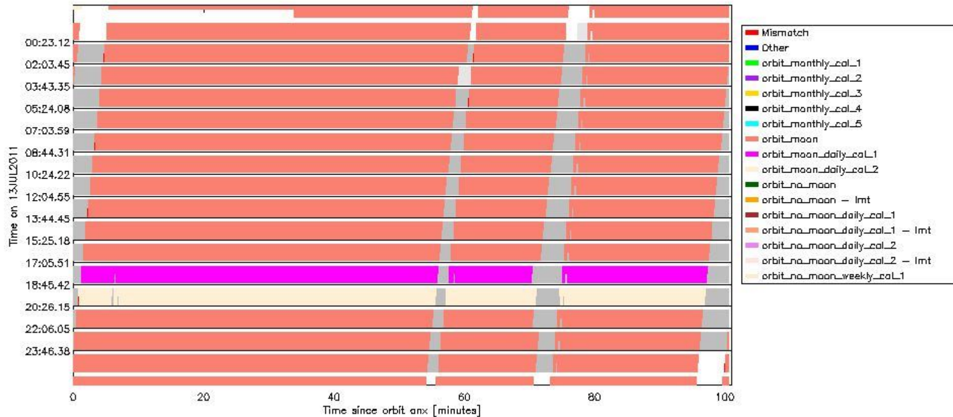
sciamachy_daily_report_level0_KSPT_L0_4504_N_20110713_6.PNG
