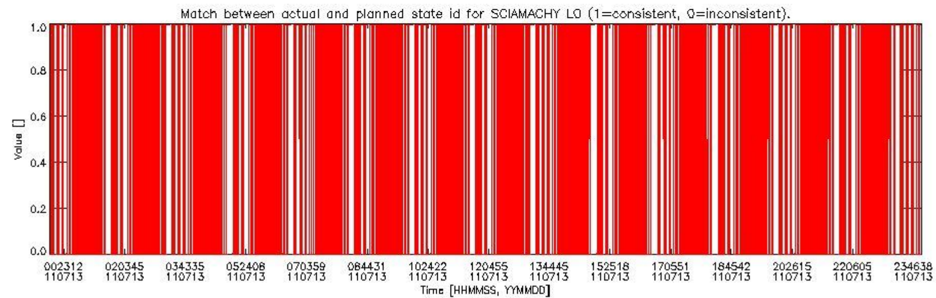
sciamachy_daily_report_level0_KSPT_L0_4504_N_20110713_5.PNG
