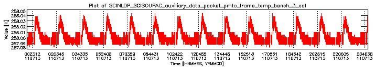
sciamachy_daily_report_level0_KSPT_L0_4504_N_20110713_2.PNG
