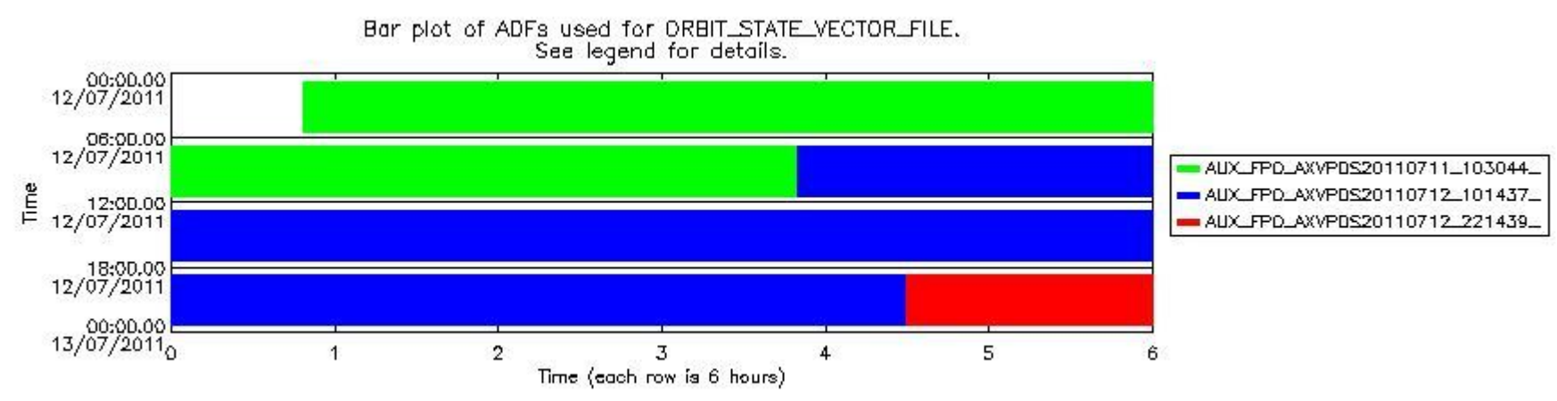
sciamachy_daily_report_level0_KSPT_L0_4504_N_20110712_8.PNG
