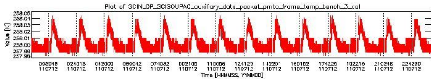
sciamachy_daily_report_level0_KSPT_L0_4504_N_20110712_2.PNG
