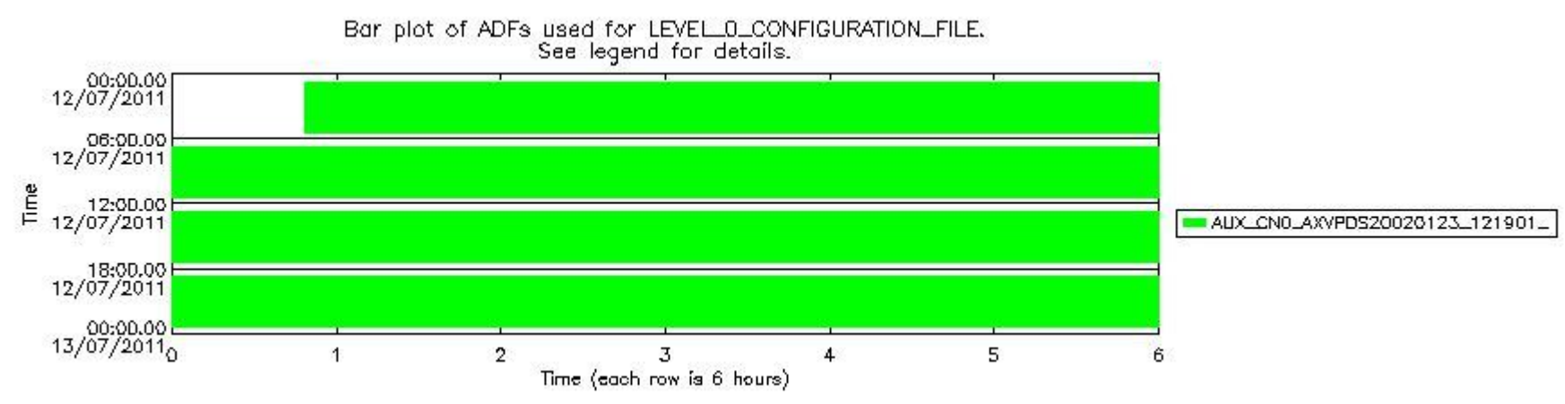
sciamachy_daily_report_level0_KSPT_L0_4504_N_20110712_7.PNG
