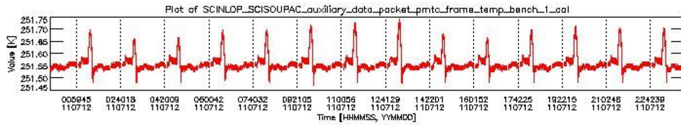
sciamachy_daily_report_level0_KSPT_L0_4504_N_20110712_0.PNG
