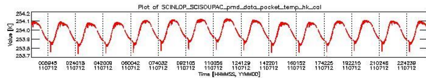
sciamachy_daily_report_level0_KSPT_L0_4504_N_20110712_3.PNG
