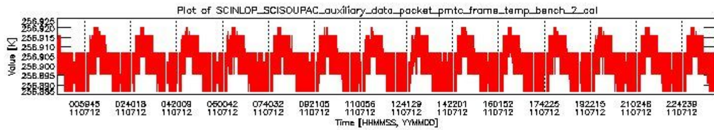
sciamachy_daily_report_level0_KSPT_L0_4504_N_20110712_1.PNG
