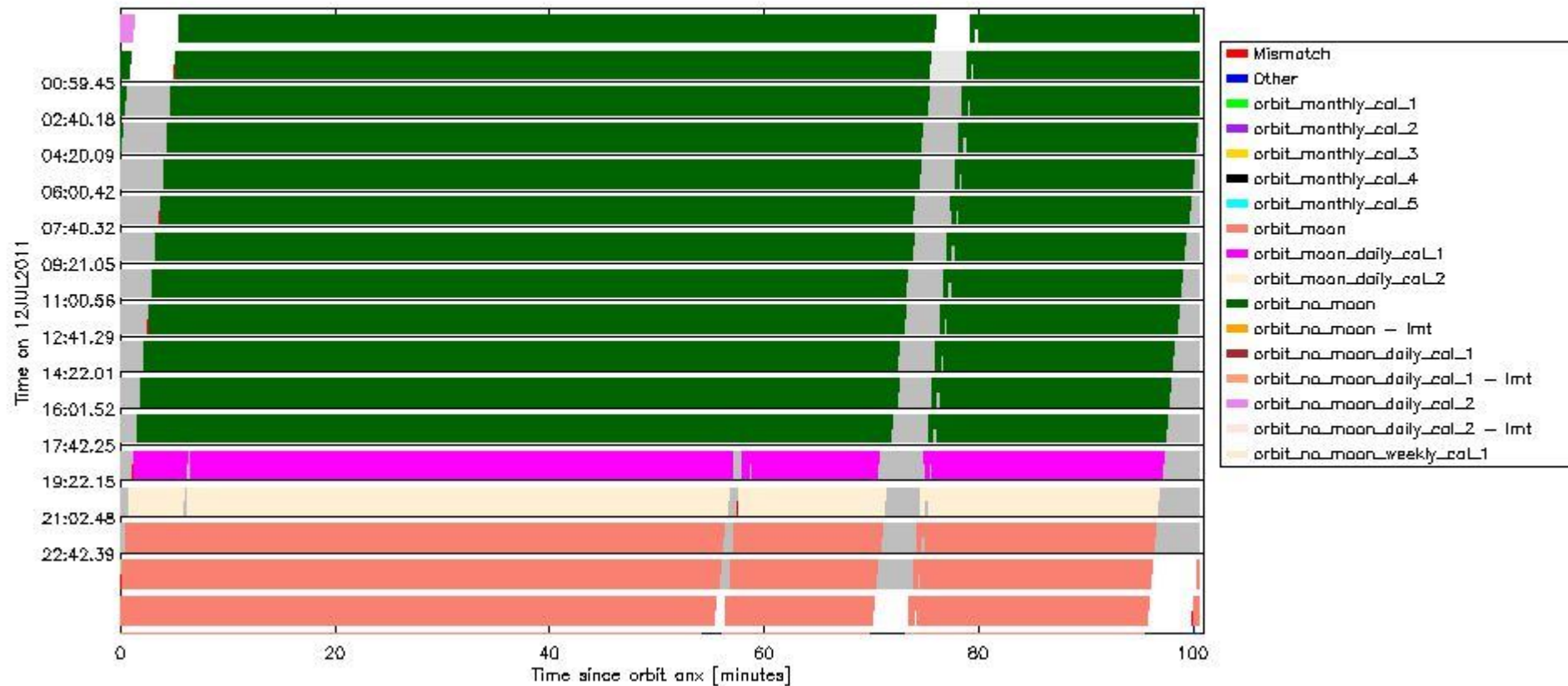
sciamachy_daily_report_level0_KSPT_L0_4504_N_20110712_6.PNG
