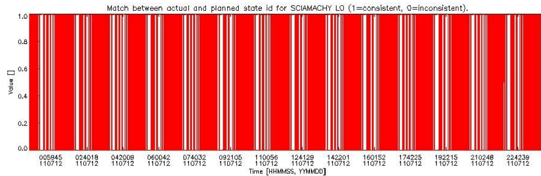
sciamachy_daily_report_level0_KSPT_L0_4504_N_20110712_5.PNG
