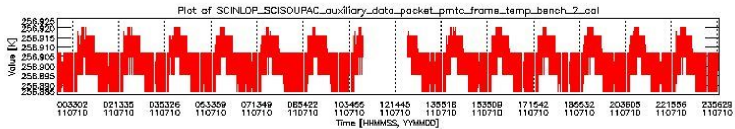
sciamachy_daily_report_level0_KSPT_L0_4504_N_20110710_1.PNG
