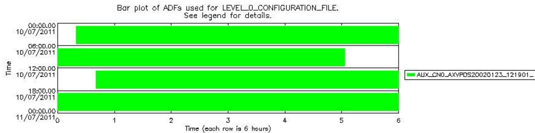
sciamachy_daily_report_level0_KSPT_L0_4504_N_20110710_7.PNG
