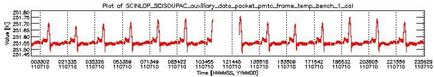
sciamachy_daily_report_level0_KSPT_L0_4504_N_20110710_0.PNG
