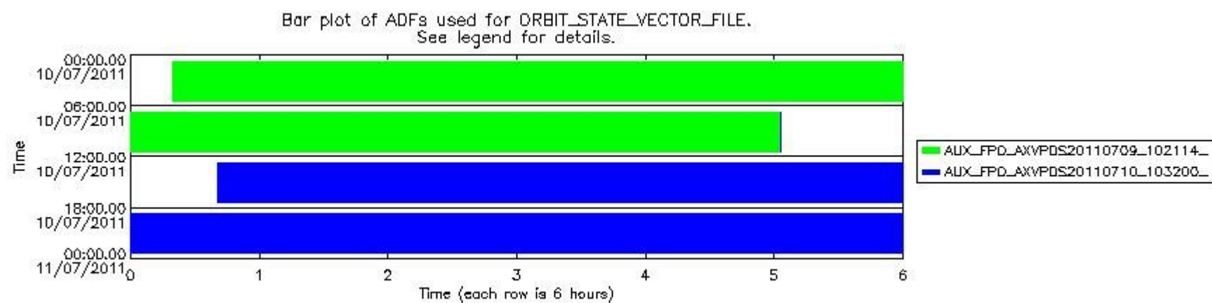
sciamachy_daily_report_level0_KSPT_L0_4504_N_20110710_8.PNG
