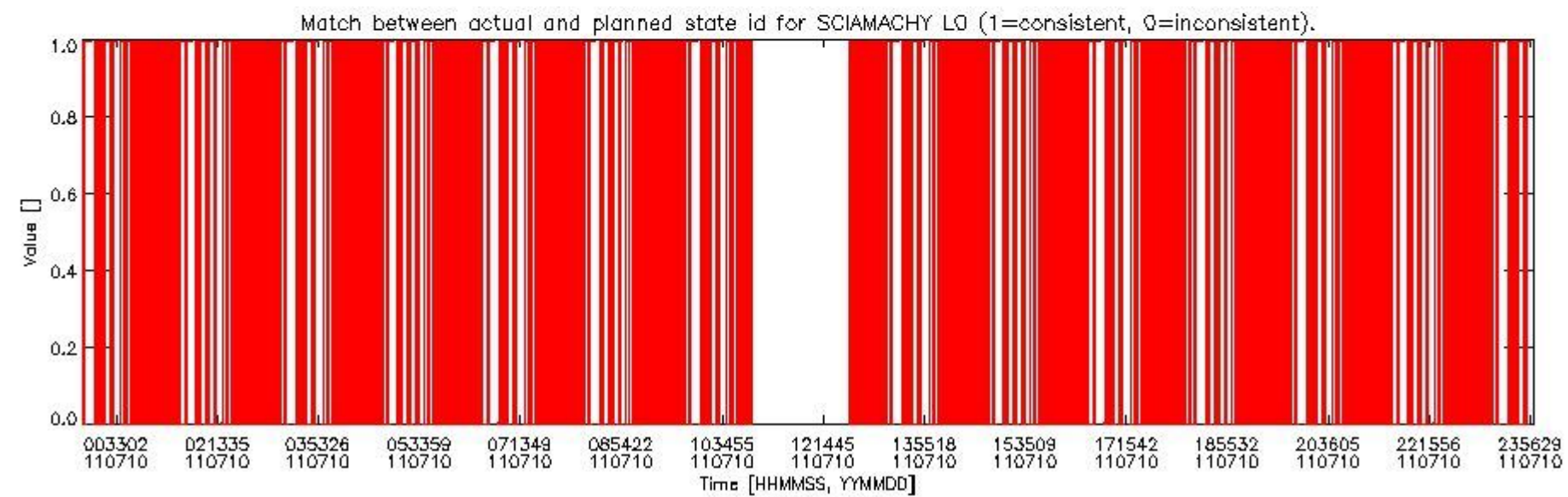
sciamachy_daily_report_level0_KSPT_L0_4504_N_20110710_5.PNG
