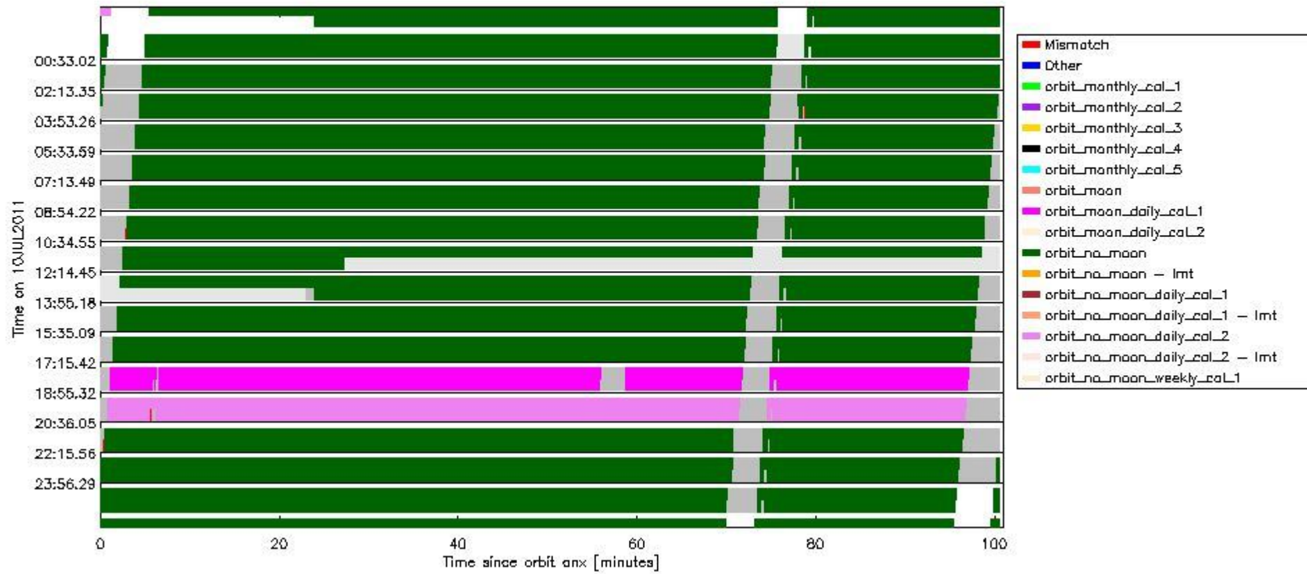
sciamachy_daily_report_level0_KSPT_L0_4504_N_20110710_6.PNG
