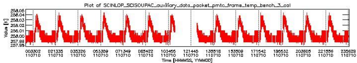
sciamachy_daily_report_level0_KSPT_L0_4504_N_20110710_2.PNG
