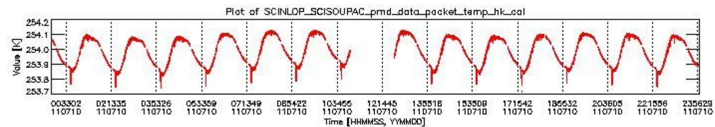
sciamachy_daily_report_level0_KSPT_L0_4504_N_20110710_3.PNG
