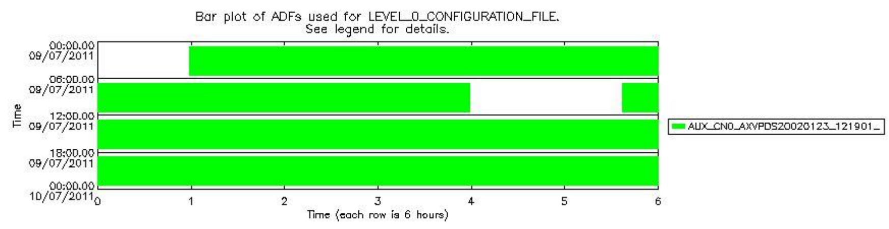
sciamachy_daily_report_level0_KSPT_L0_4504_N_20110709_7.PNG
