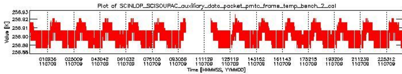
sciamachy_daily_report_level0_KSPT_L0_4504_N_20110709_1.PNG
