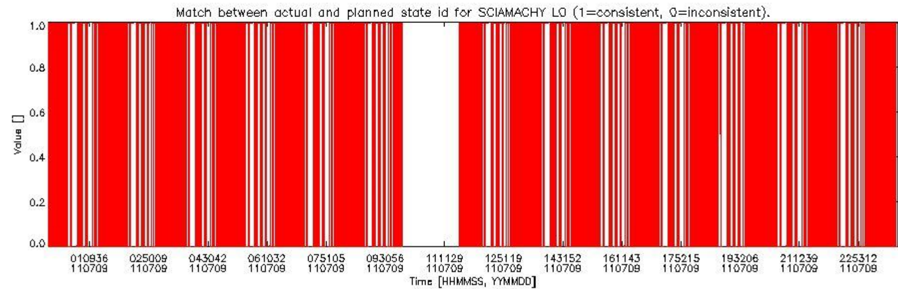
sciamachy_daily_report_level0_KSPT_L0_4504_N_20110709_5.PNG
