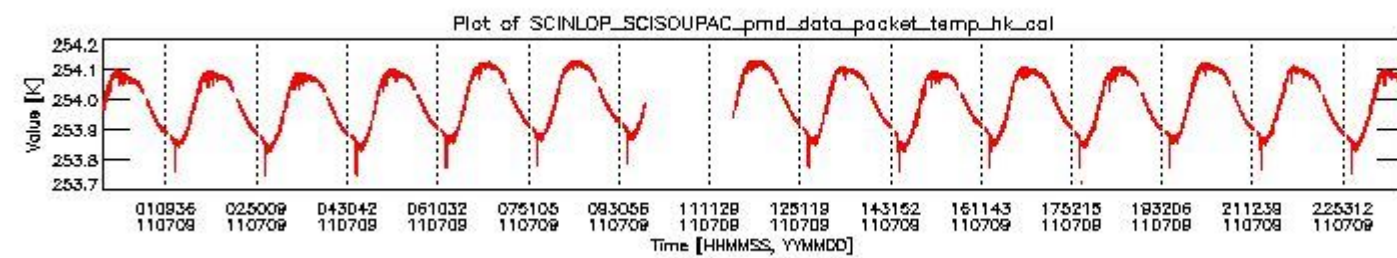
sciamachy_daily_report_level0_KSPT_L0_4504_N_20110709_3.PNG
