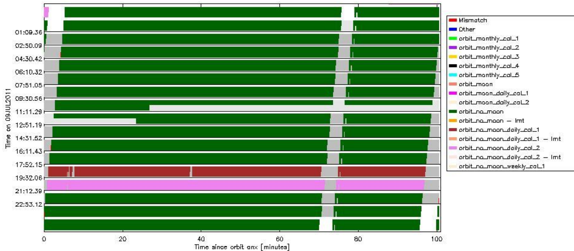
sciamachy_daily_report_level0_KSPT_L0_4504_N_20110709_6.PNG
