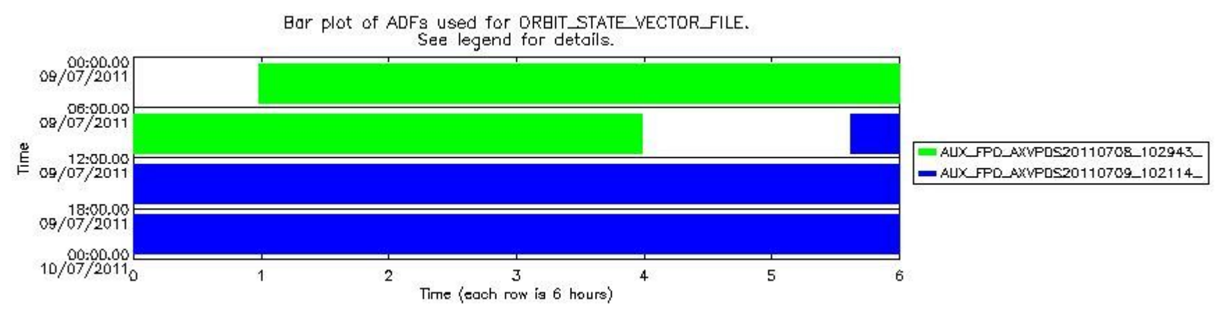
sciamachy_daily_report_level0_KSPT_L0_4504_N_20110709_8.PNG
