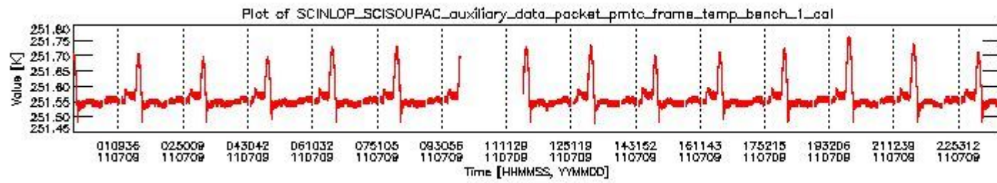
sciamachy_daily_report_level0_KSPT_L0_4504_N_20110709_0.PNG
