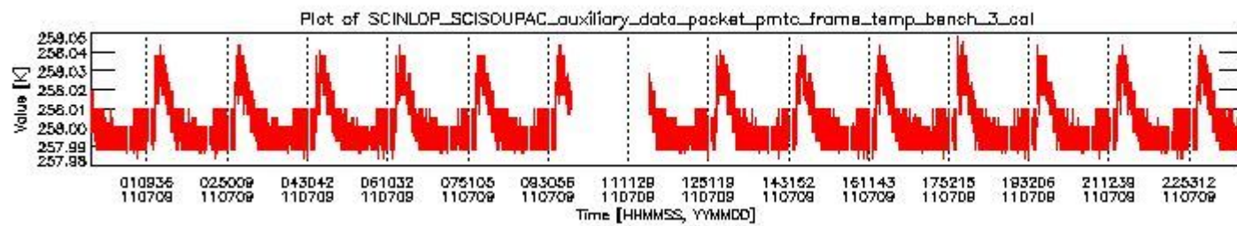
sciamachy_daily_report_level0_KSPT_L0_4504_N_20110709_2.PNG
