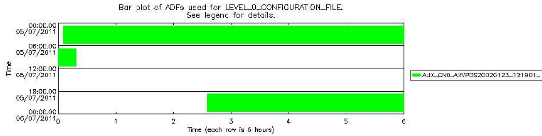
sciamachy_daily_report_level0_KSPT_L0_4504_N_20110705_7.PNG
