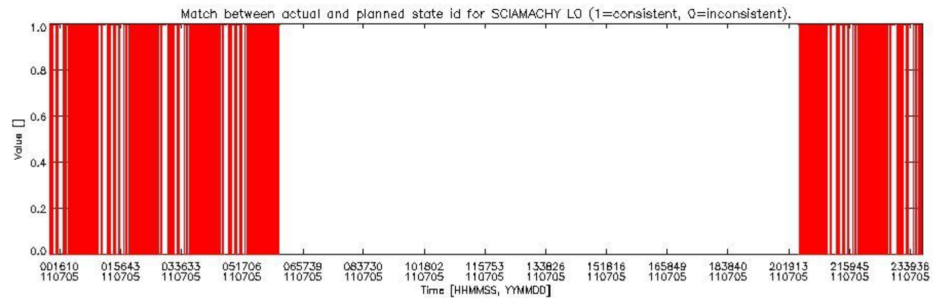
sciamachy_daily_report_level0_KSPT_L0_4504_N_20110705_5.PNG
