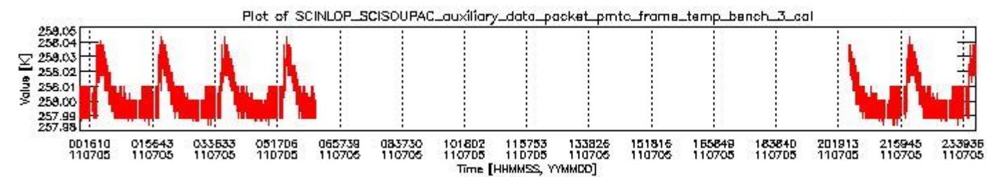
sciamachy_daily_report_level0_KSPT_L0_4504_N_20110705_2.PNG
