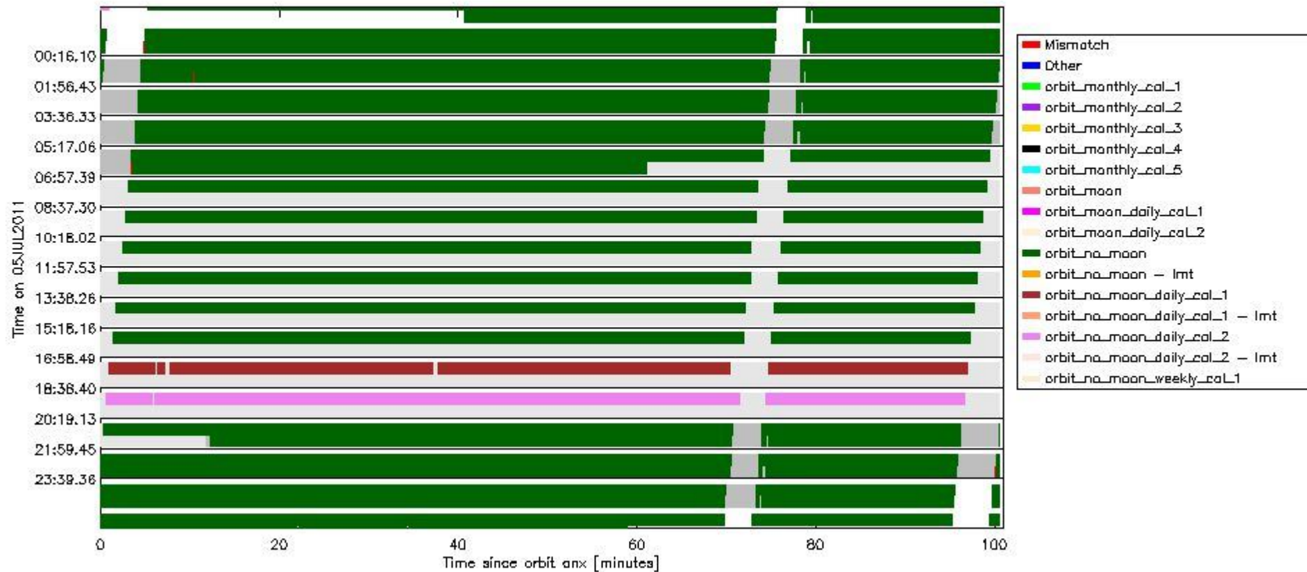
sciamachy_daily_report_level0_KSPT_L0_4504_N_20110705_6.PNG
