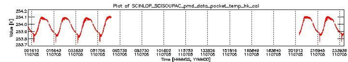
sciamachy_daily_report_level0_KSPT_L0_4504_N_20110705_3.PNG
