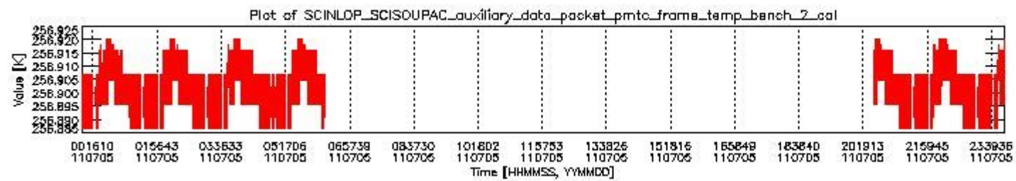
sciamachy_daily_report_level0_KSPT_L0_4504_N_20110705_1.PNG
