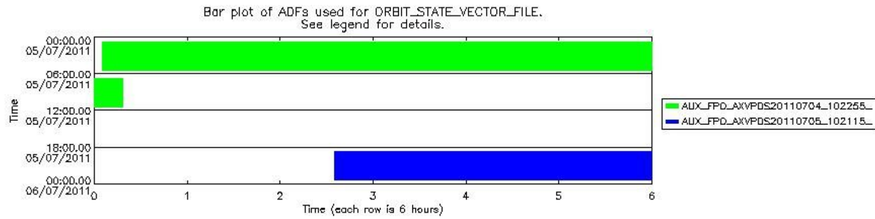
sciamachy_daily_report_level0_KSPT_L0_4504_N_20110705_8.PNG
