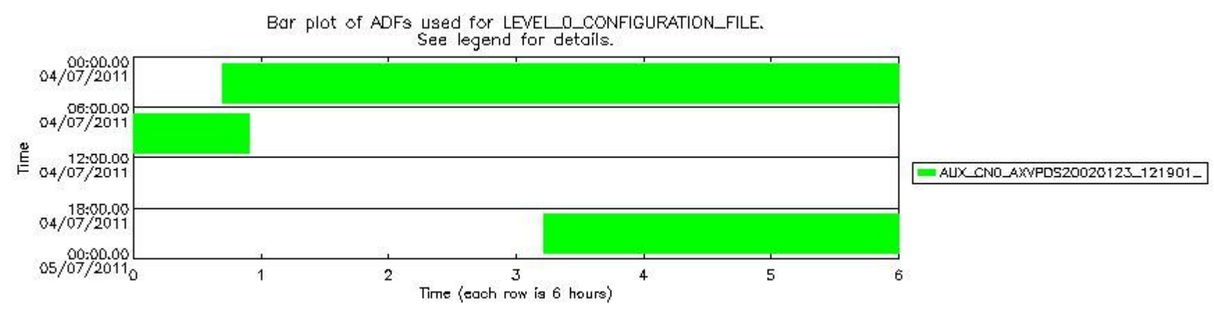
sciamachy_daily_report_level0_KSPT_L0_4504_N_20110704_7.PNG
