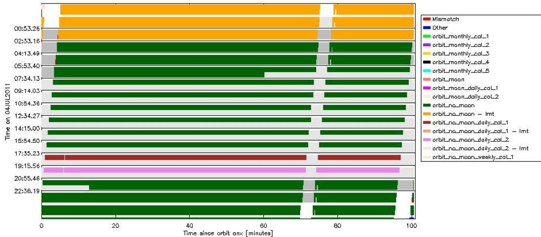
sciamachy_daily_report_level0_KSPT_L0_4504_N_20110704_6.PNG
