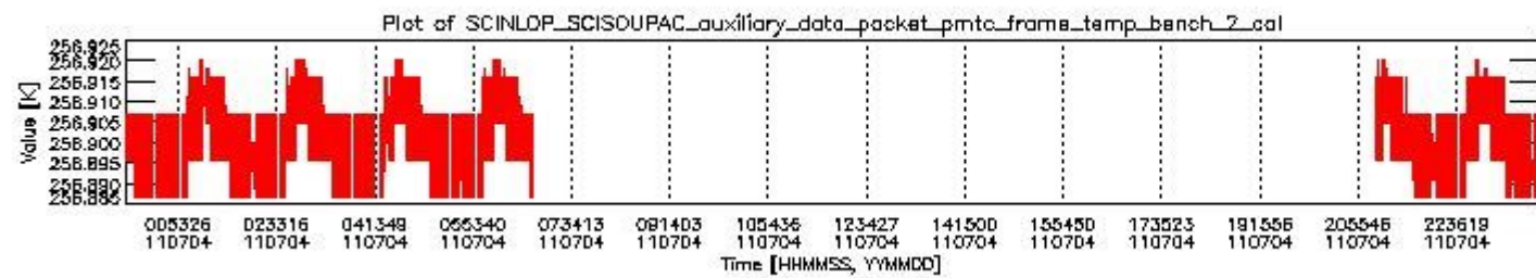
sciamachy_daily_report_level0_KSPT_L0_4504_N_20110704_1.PNG
