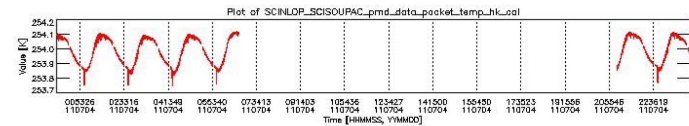
sciamachy_daily_report_level0_KSPT_L0_4504_N_20110704_3.PNG
