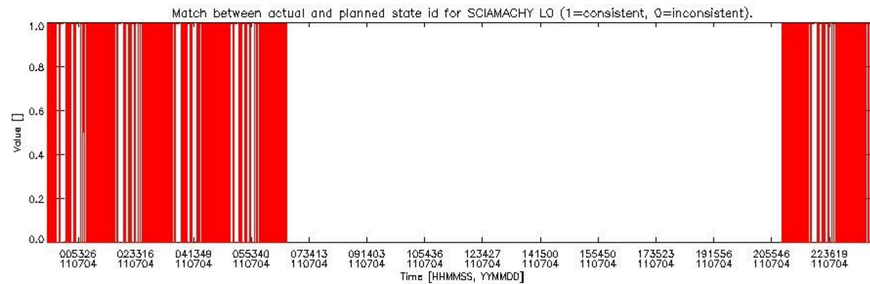
sciamachy_daily_report_level0_KSPT_L0_4504_N_20110704_5.PNG
