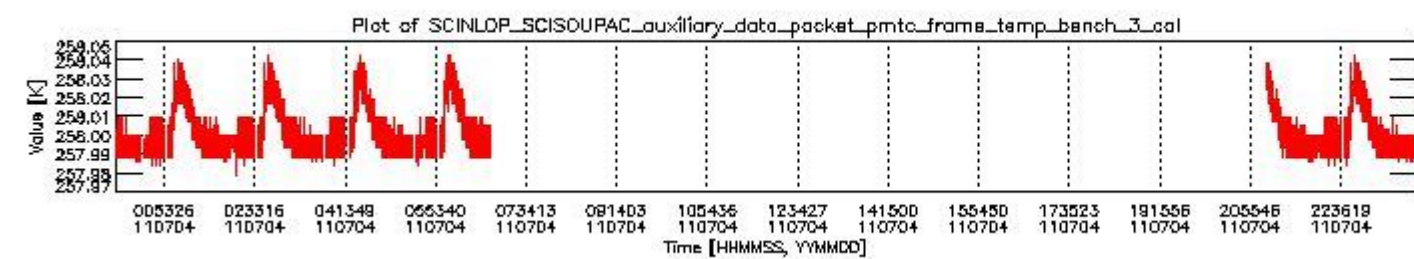
sciamachy_daily_report_level0_KSPT_L0_4504_N_20110704_2.PNG
