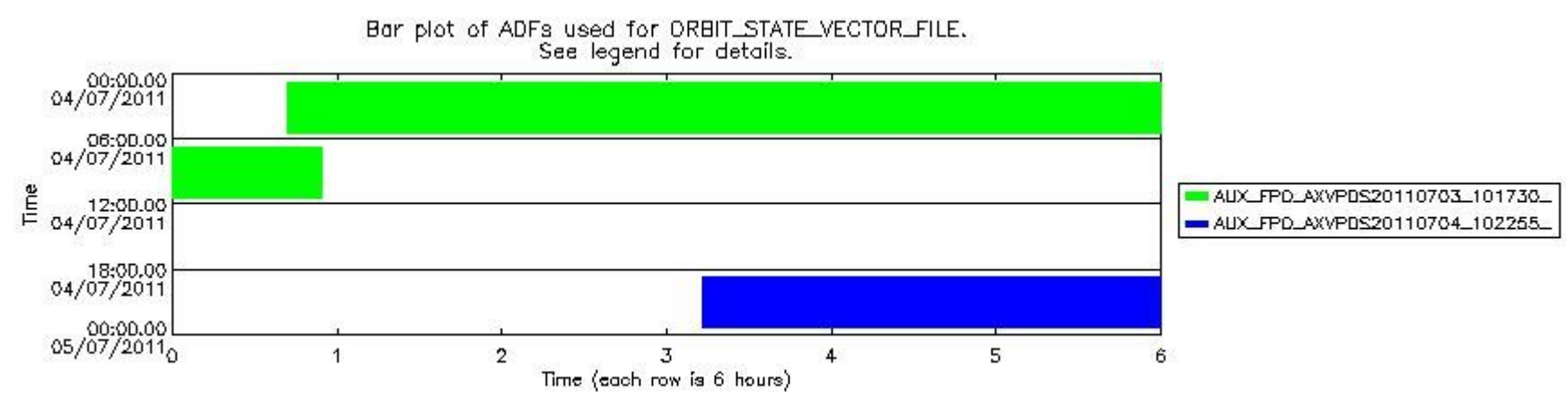
sciamachy_daily_report_level0_KSPT_L0_4504_N_20110704_8.PNG
