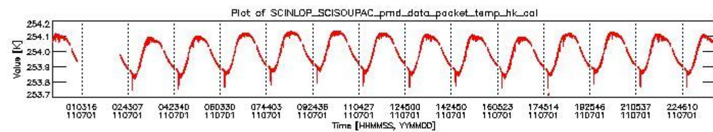
sciamachy_daily_report_level0_KSPT_L0_4504_N_20110701_3.PNG
