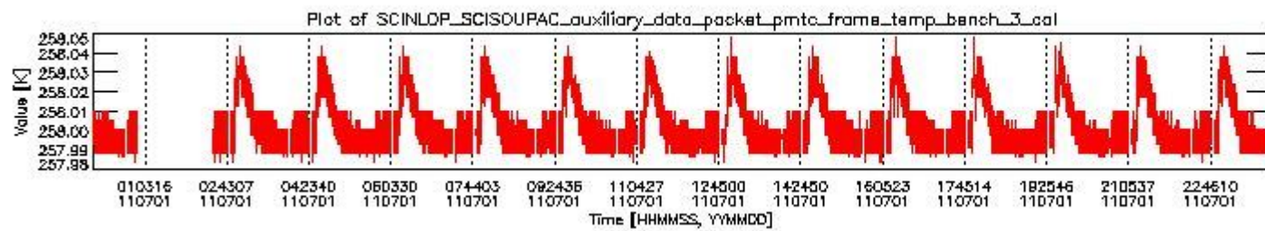
sciamachy_daily_report_level0_KSPT_L0_4504_N_20110701_2.PNG
