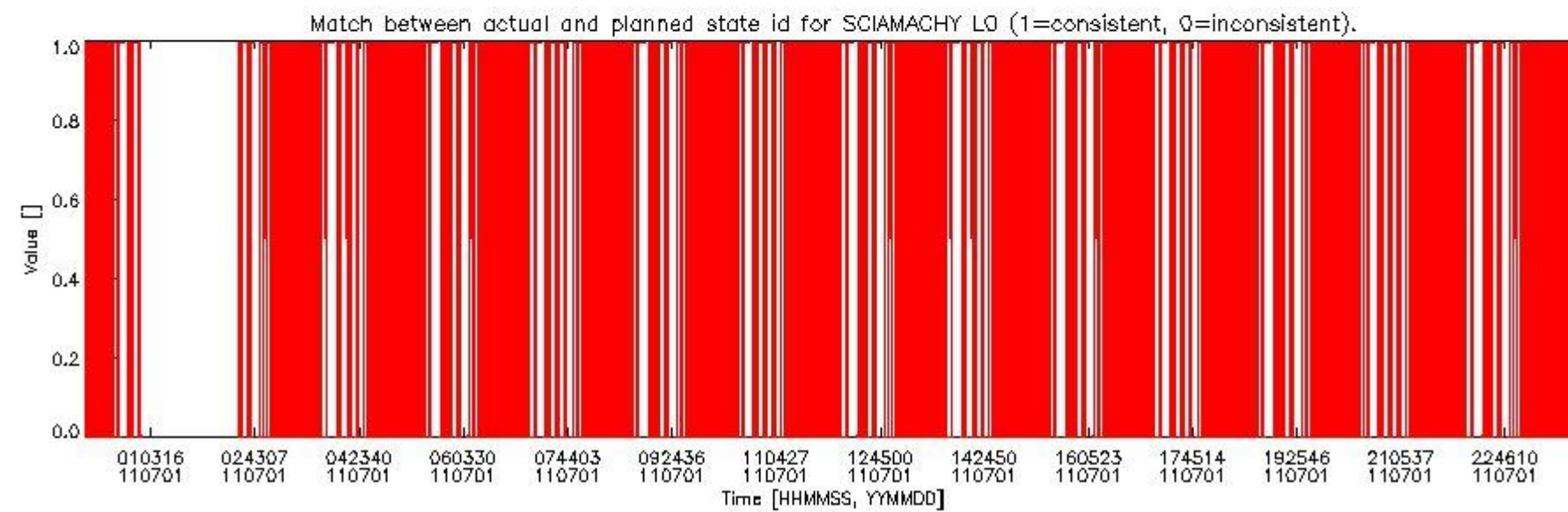
sciamachy_daily_report_level0_KSPT_L0_4504_N_20110701_5.PNG
