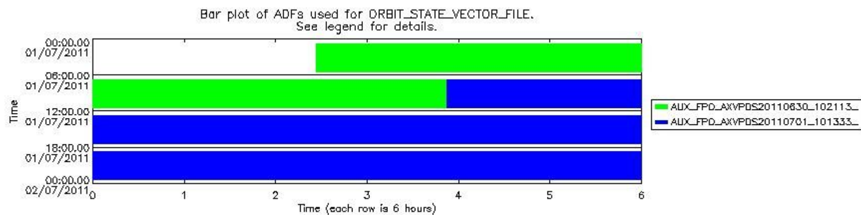
sciamachy_daily_report_level0_KSPT_L0_4504_N_20110701_8.PNG
