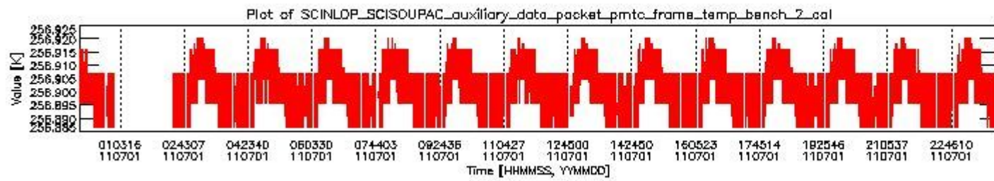
sciamachy_daily_report_level0_KSPT_L0_4504_N_20110701_1.PNG
