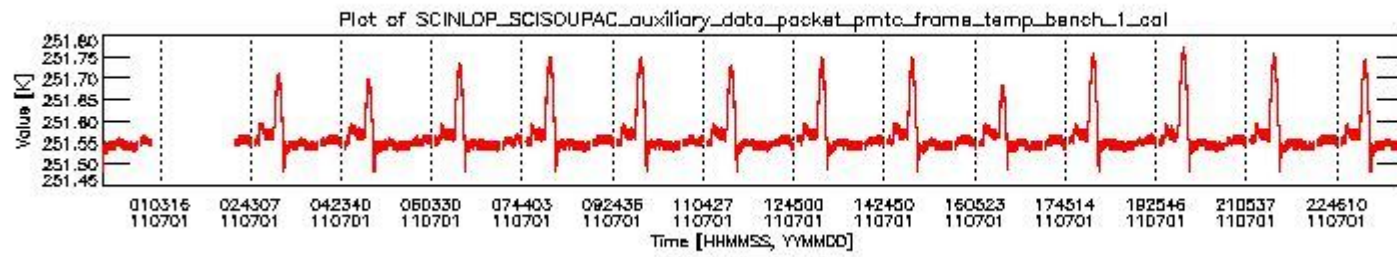
sciamachy_daily_report_level0_KSPT_L0_4504_N_20110701_0.PNG
