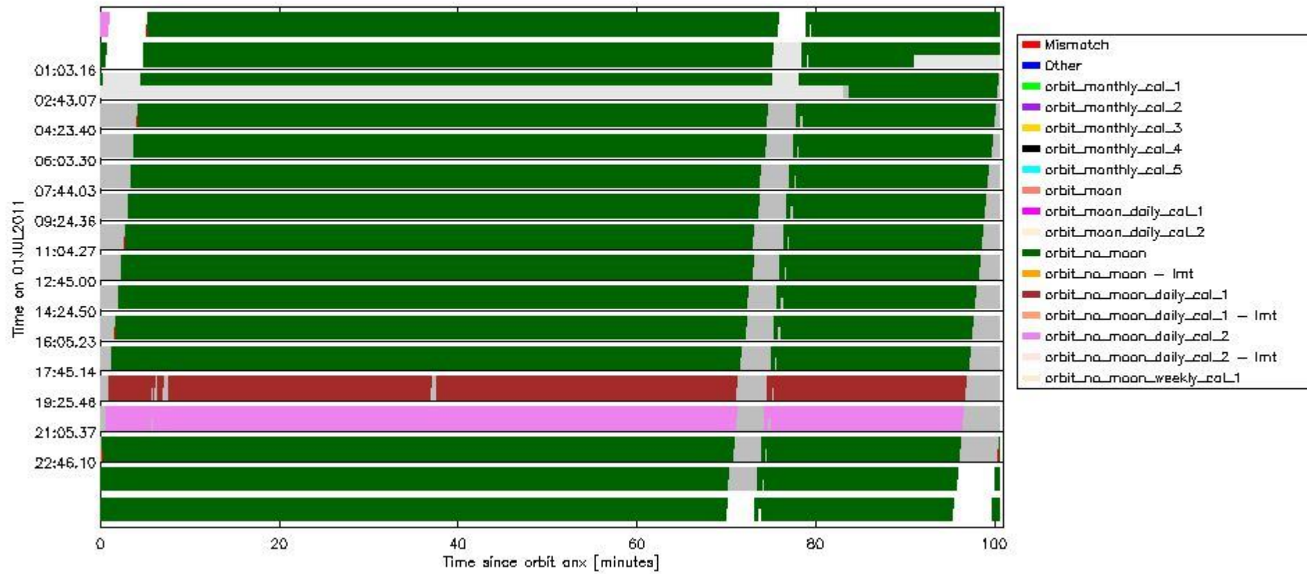
sciamachy_daily_report_level0_KSPT_L0_4504_N_20110701_6.PNG
