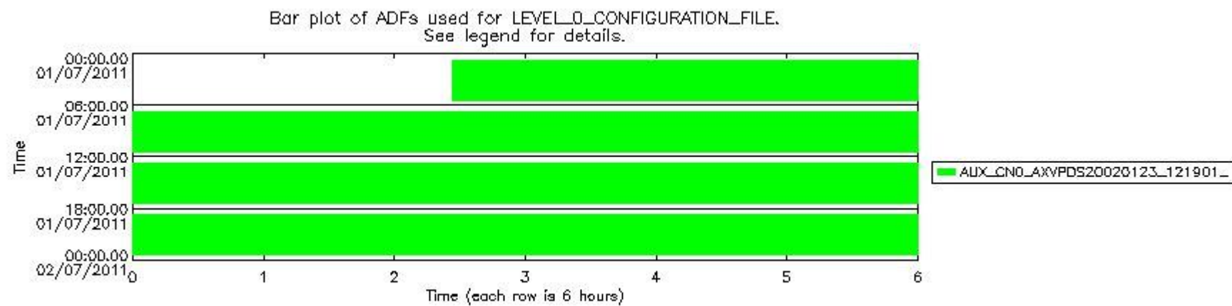
sciamachy_daily_report_level0_KSPT_L0_4504_N_20110701_7.PNG
