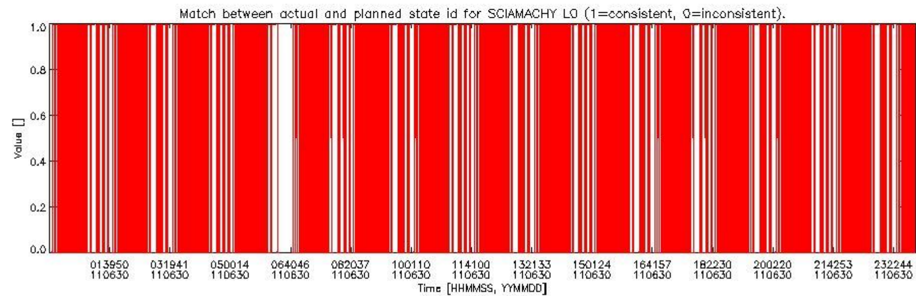
sciamachy_daily_report_level0_KSPT_L0_4504_N_20110630_5.PNG
