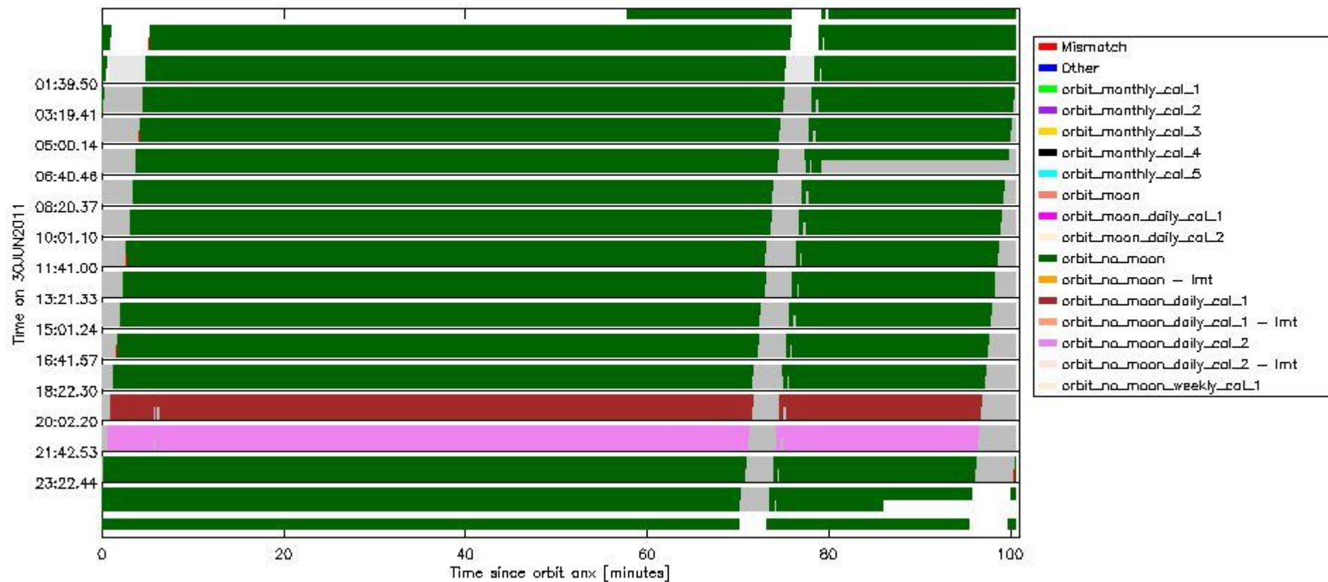
sciamachy_daily_report_level0_KSPT_L0_4504_N_20110630_6.PNG
