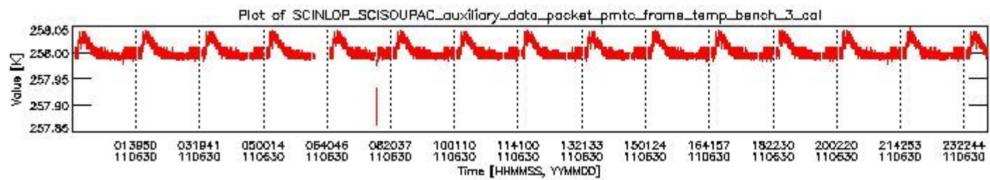
sciamachy_daily_report_level0_KSPT_L0_4504_N_20110630_2.PNG
