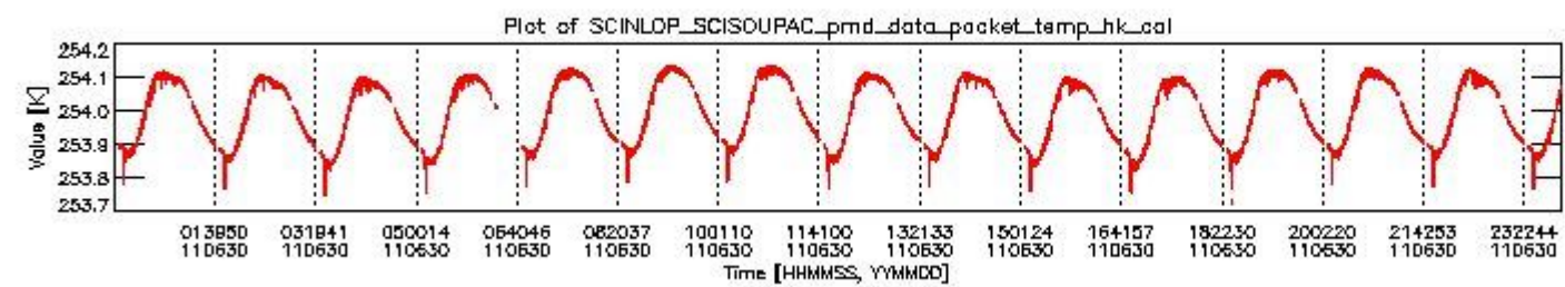
sciamachy_daily_report_level0_KSPT_L0_4504_N_20110630_3.PNG
