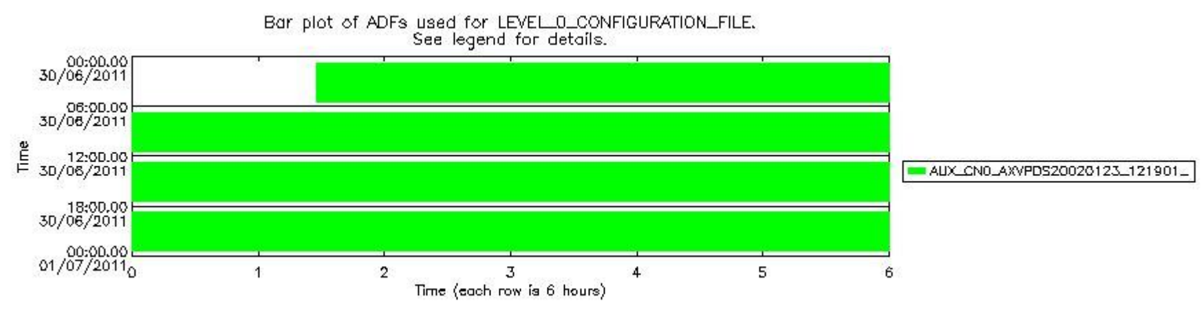
sciamachy_daily_report_level0_KSPT_L0_4504_N_20110630_7.PNG
