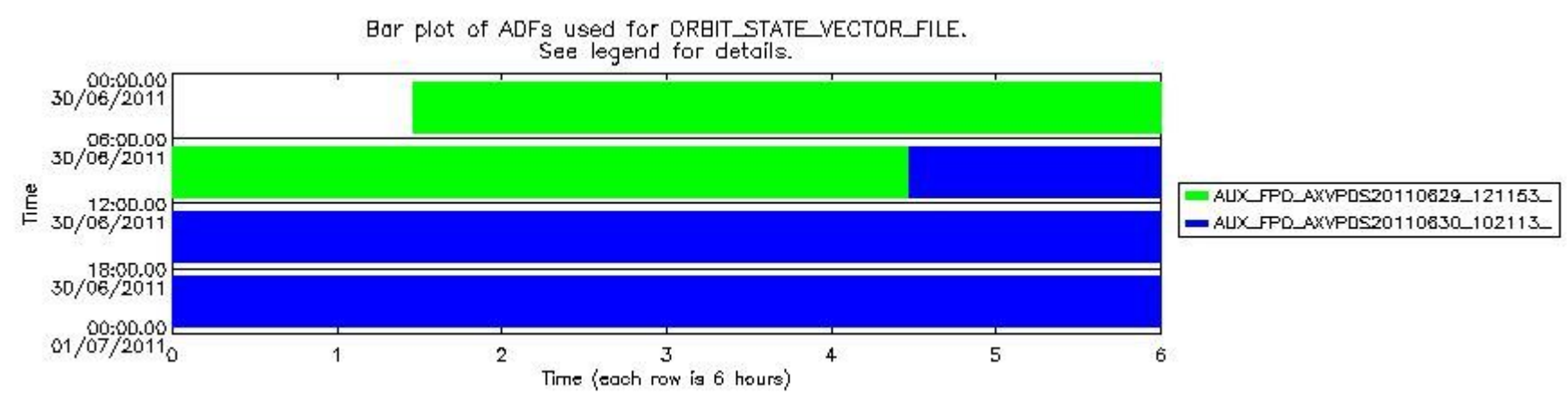
sciamachy_daily_report_level0_KSPT_L0_4504_N_20110630_8.PNG
