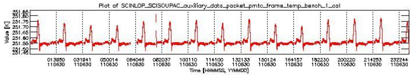
sciamachy_daily_report_level0_KSPT_L0_4504_N_20110630_0.PNG
