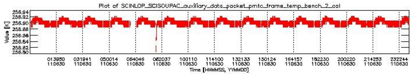
sciamachy_daily_report_level0_KSPT_L0_4504_N_20110630_1.PNG
