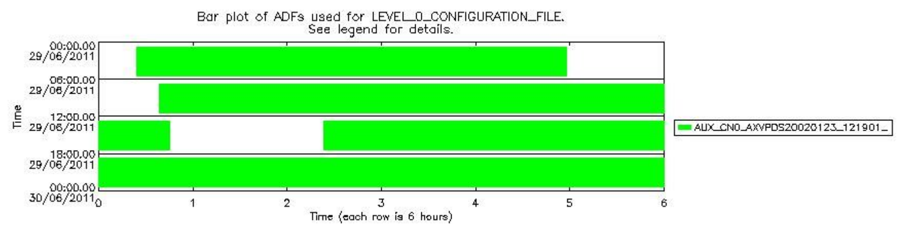
sciamachy_daily_report_level0_KSPT_L0_4504_N_20110629_7.PNG
