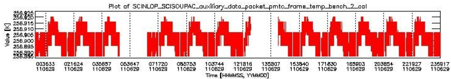
sciamachy_daily_report_level0_KSPT_L0_4504_N_20110629_1.PNG
