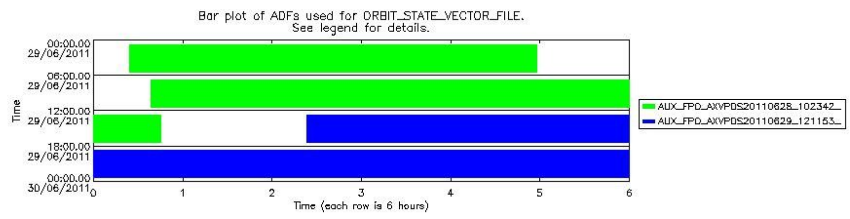
sciamachy_daily_report_level0_KSPT_L0_4504_N_20110629_8.PNG
