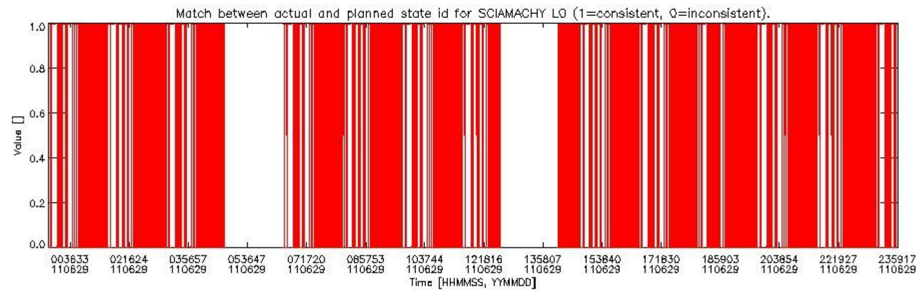
sciamachy_daily_report_level0_KSPT_L0_4504_N_20110629_5.PNG
