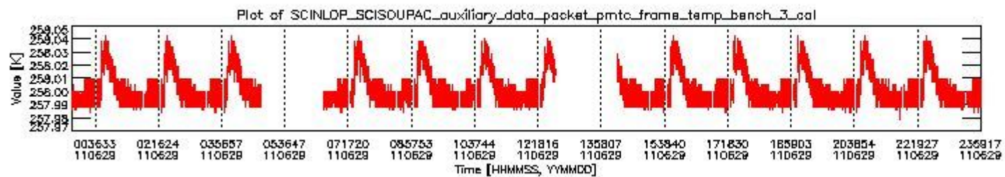
sciamachy_daily_report_level0_KSPT_L0_4504_N_20110629_2.PNG
