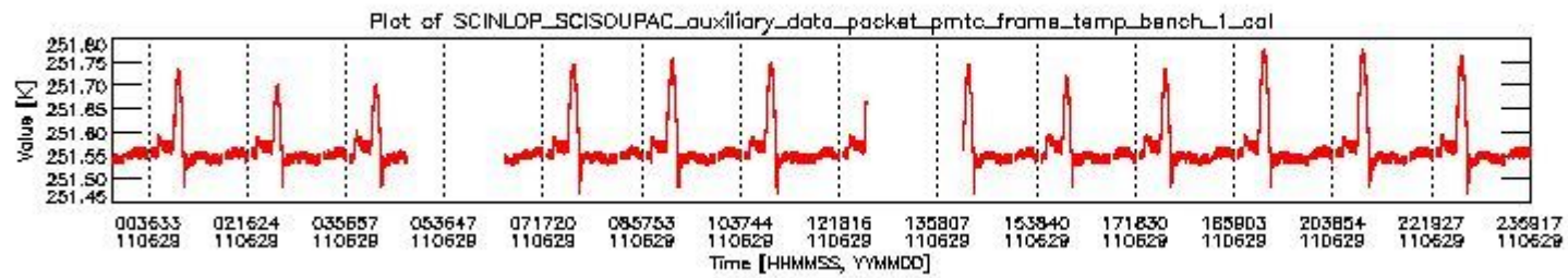
sciamachy_daily_report_level0_KSPT_L0_4504_N_20110629_0.PNG
