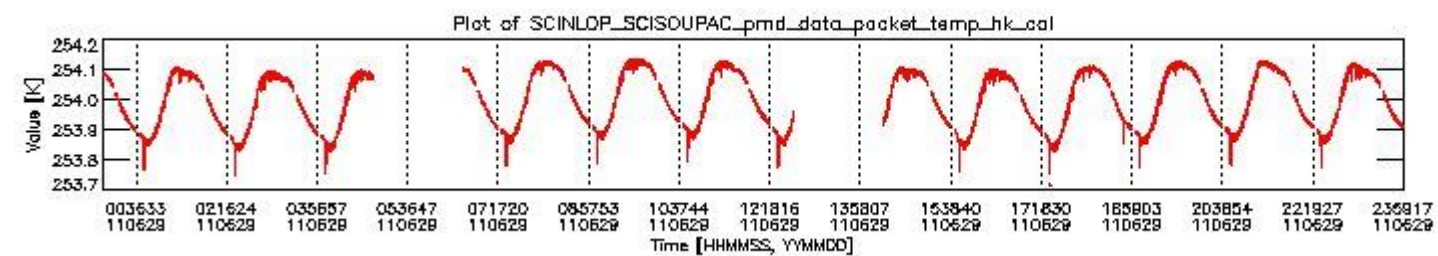
sciamachy_daily_report_level0_KSPT_L0_4504_N_20110629_3.PNG
