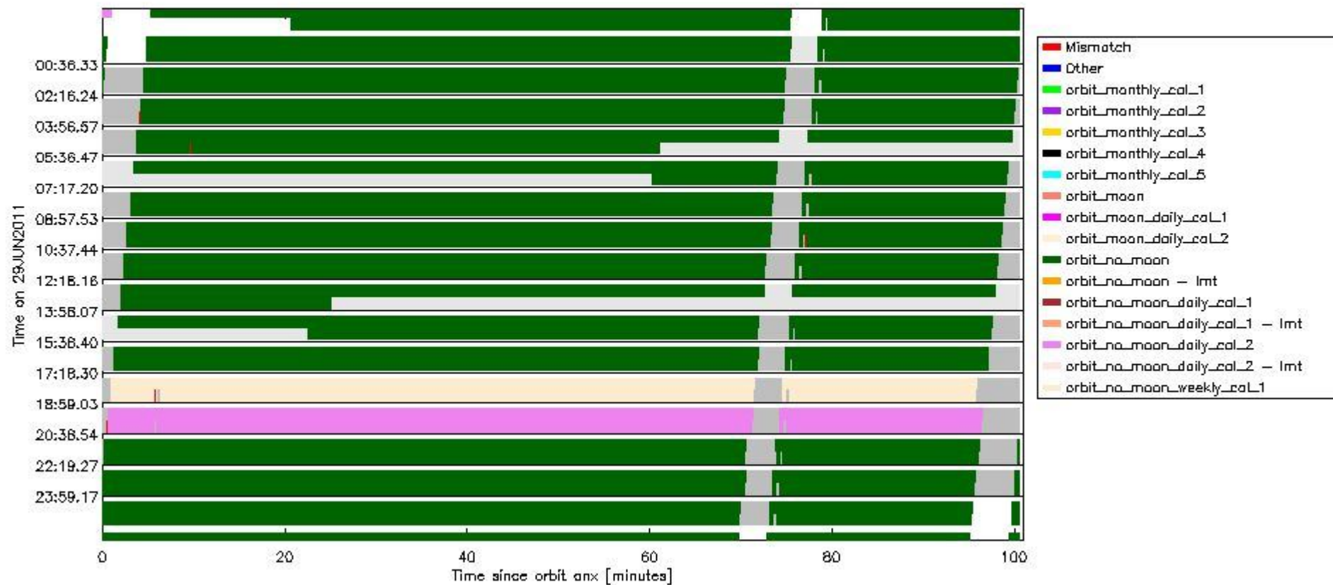
sciamachy_daily_report_level0_KSPT_L0_4504_N_20110629_6.PNG
