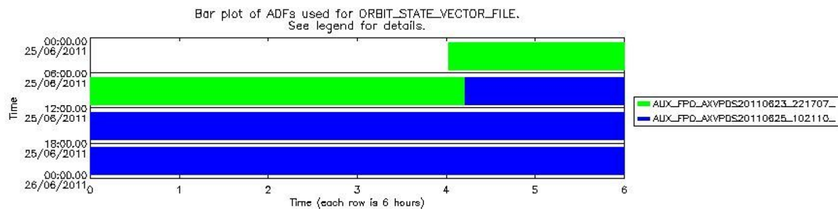
sciamachy_daily_report_level0_KSPT_L0_4504_N_20110625_8.PNG
