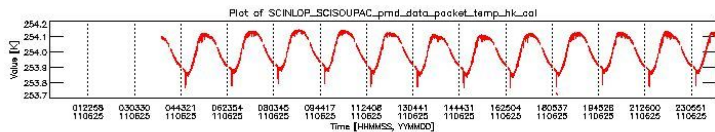
sciamachy_daily_report_level0_KSPT_L0_4504_N_20110625_3.PNG
