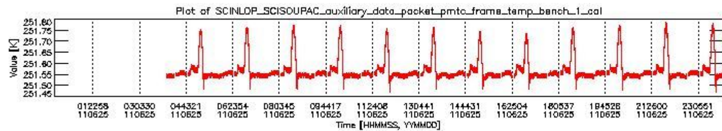
sciamachy_daily_report_level0_KSPT_L0_4504_N_20110625_0.PNG
