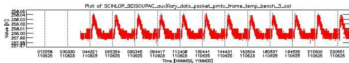
sciamachy_daily_report_level0_KSPT_L0_4504_N_20110625_2.PNG
