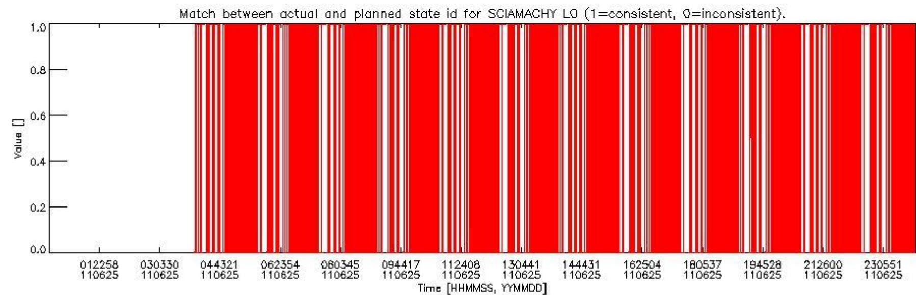
sciamachy_daily_report_level0_KSPT_L0_4504_N_20110625_5.PNG
