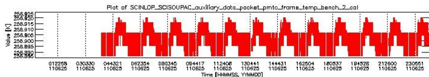
sciamachy_daily_report_level0_KSPT_L0_4504_N_20110625_1.PNG
