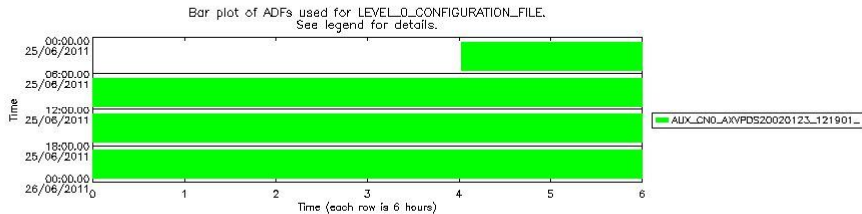
sciamachy_daily_report_level0_KSPT_L0_4504_N_20110625_7.PNG
