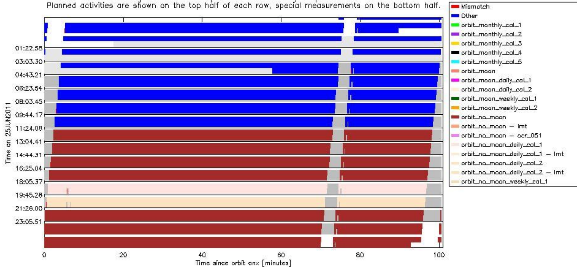
sciamachy_daily_report_level0_KSPT_L0_4504_N_20110625_6.PNG
