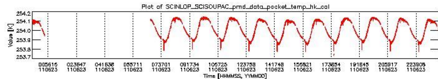
sciamachy_daily_report_level0_KSPT_L0_4504_N_20110623_3.PNG
