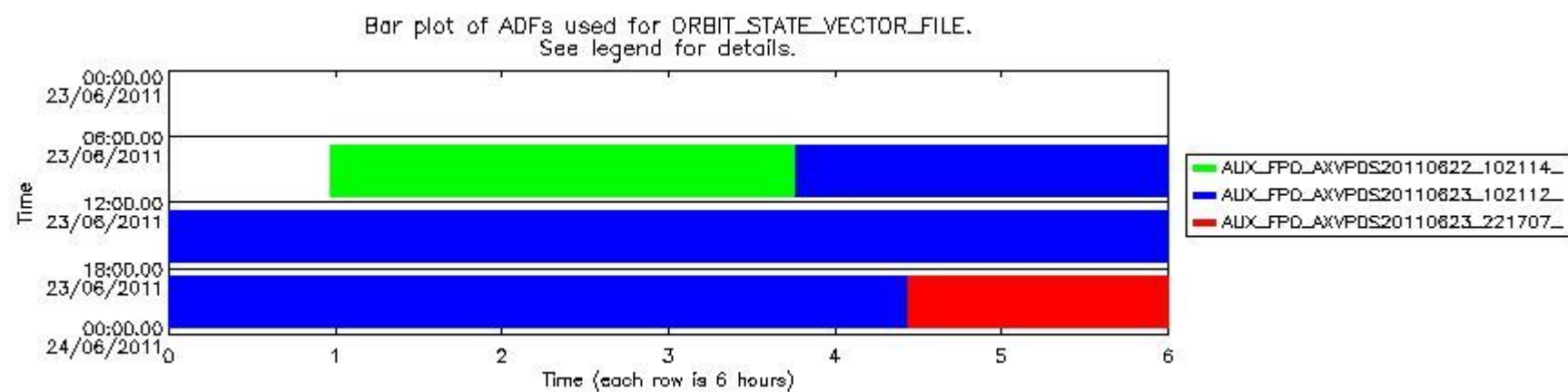
sciamachy_daily_report_level0_KSPT_L0_4504_N_20110623_8.PNG
