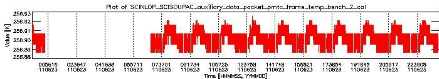
sciamachy_daily_report_level0_KSPT_L0_4504_N_20110623_1.PNG
