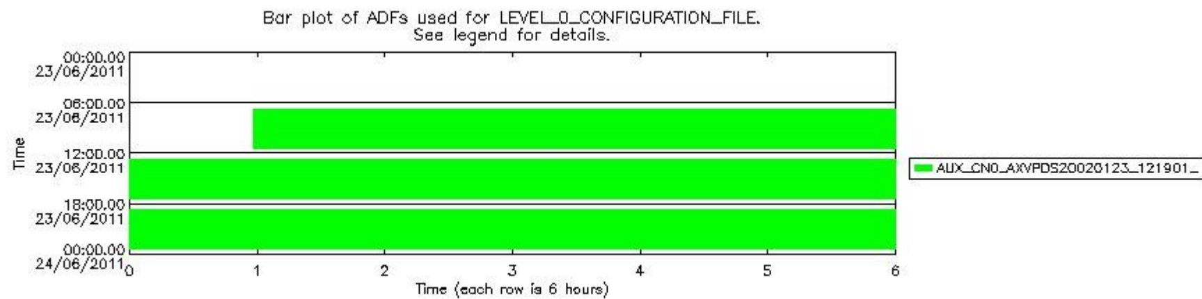
sciamachy_daily_report_level0_KSPT_L0_4504_N_20110623_7.PNG
