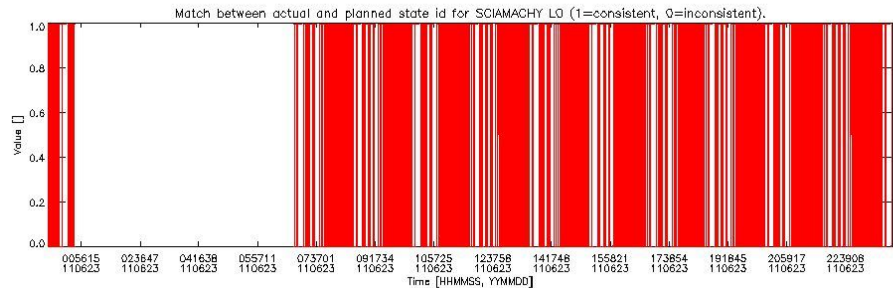
sciamachy_daily_report_level0_KSPT_L0_4504_N_20110623_5.PNG
