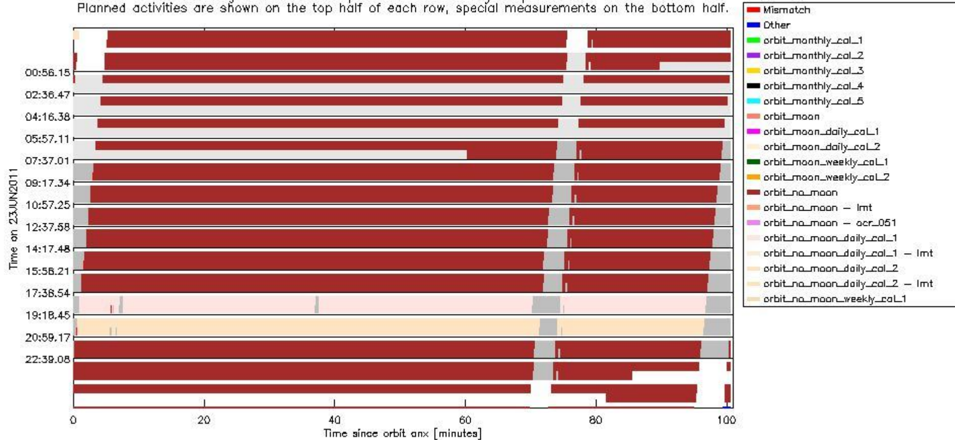
sciamachy_daily_report_level0_KSPT_L0_4504_N_20110623_6.PNG
