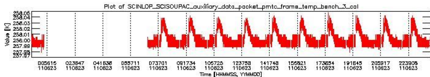
sciamachy_daily_report_level0_KSPT_L0_4504_N_20110623_2.PNG
