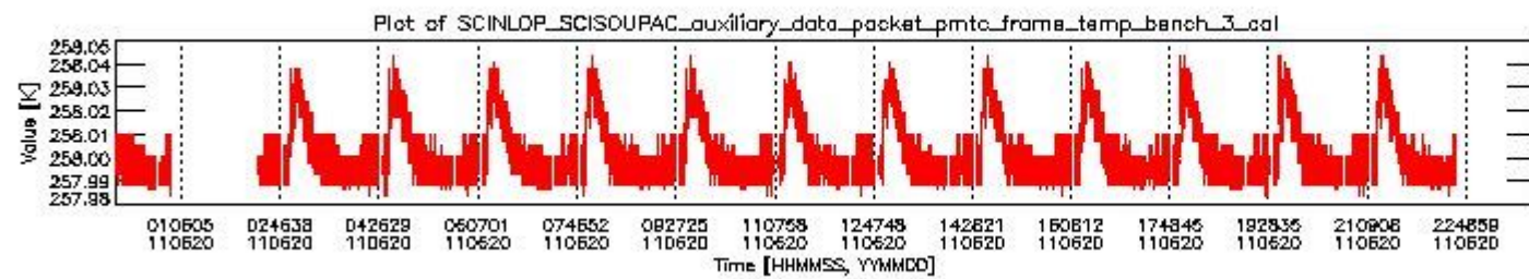
sciamachy_daily_report_level0_KSPT_L0_4504_N_20110620_2.PNG
