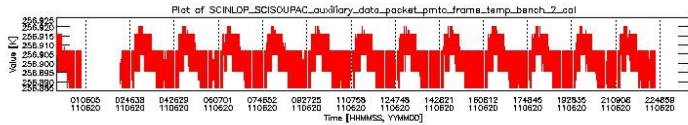
sciamachy_daily_report_level0_KSPT_L0_4504_N_20110620_1.PNG
