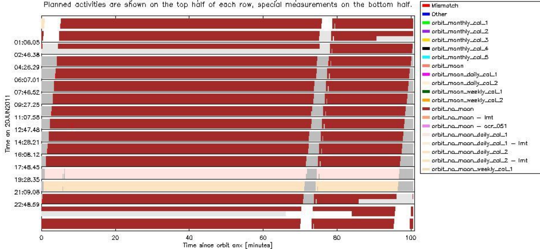
sciamachy_daily_report_level0_KSPT_L0_4504_N_20110620_6.PNG
