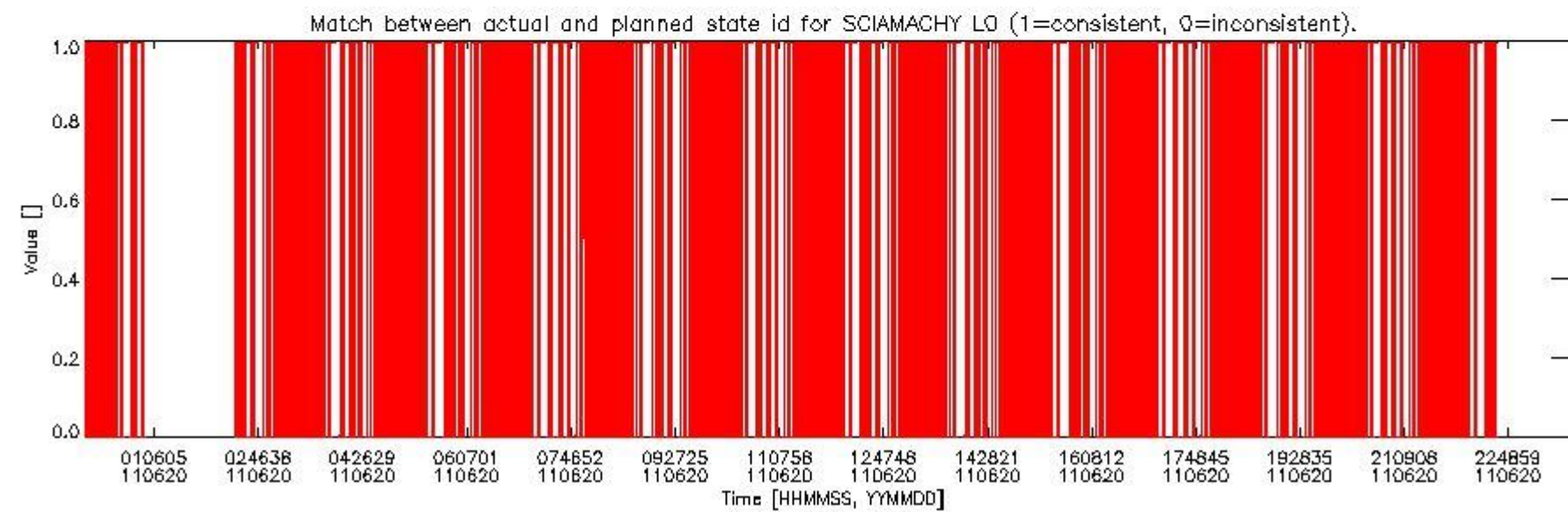
sciamachy_daily_report_level0_KSPT_L0_4504_N_20110620_5.PNG
