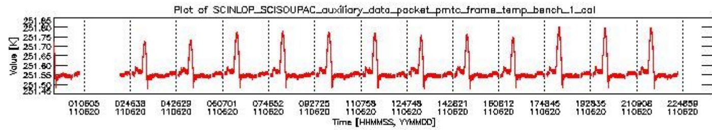
sciamachy_daily_report_level0_KSPT_L0_4504_N_20110620_0.PNG
