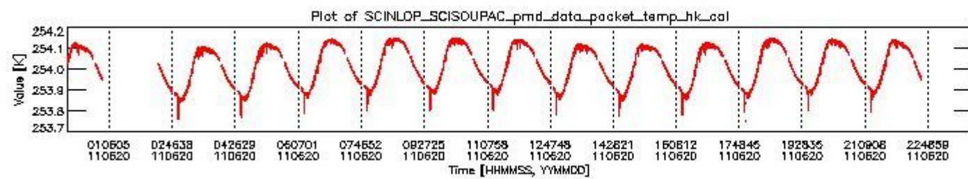
sciamachy_daily_report_level0_KSPT_L0_4504_N_20110620_3.PNG
