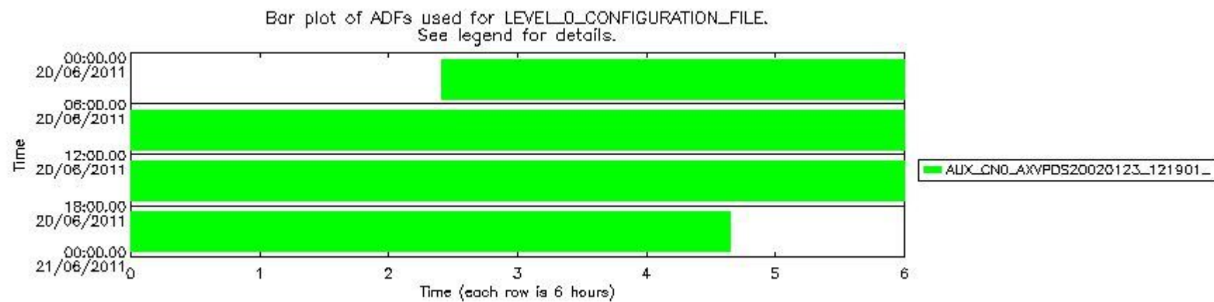
sciamachy_daily_report_level0_KSPT_L0_4504_N_20110620_7.PNG
