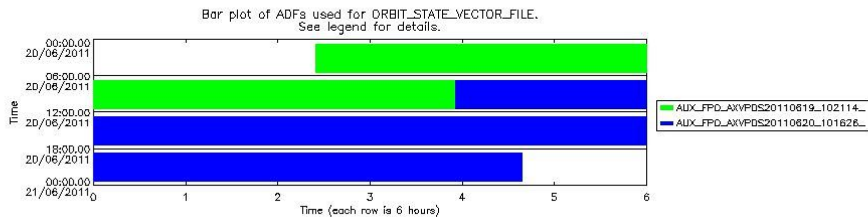
sciamachy_daily_report_level0_KSPT_L0_4504_N_20110620_8.PNG
