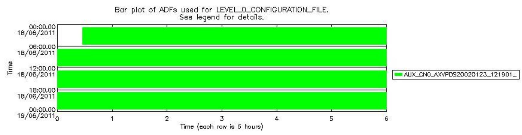
sciamachy_daily_report_level0_KSPT_L0_4504_N_20110618_7.PNG
