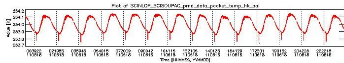
sciamachy_daily_report_level0_KSPT_L0_4504_N_20110618_3.PNG
