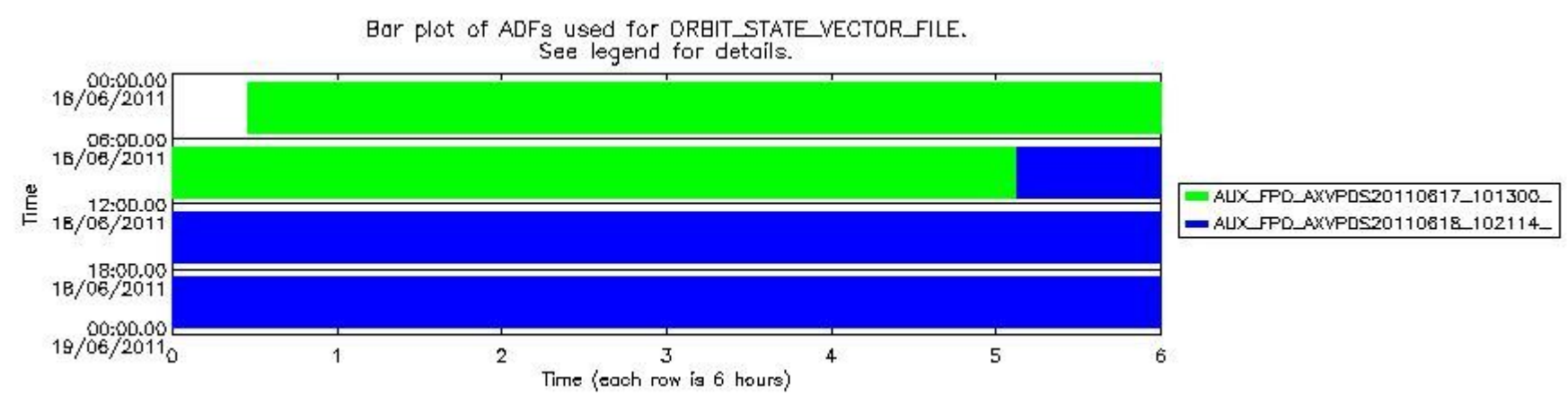
sciamachy_daily_report_level0_KSPT_L0_4504_N_20110618_8.PNG
