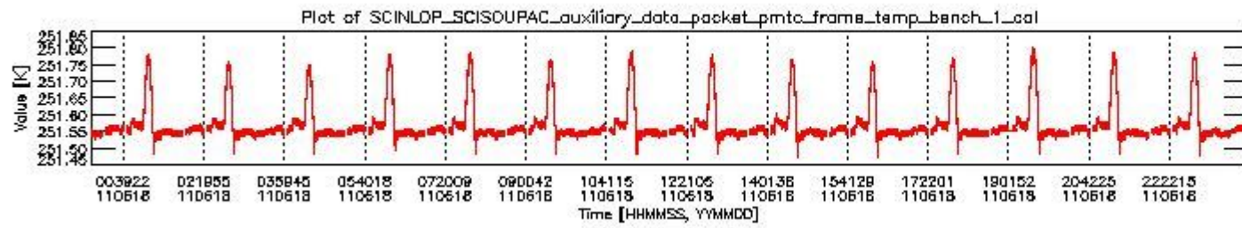
sciamachy_daily_report_level0_KSPT_L0_4504_N_20110618_0.PNG
