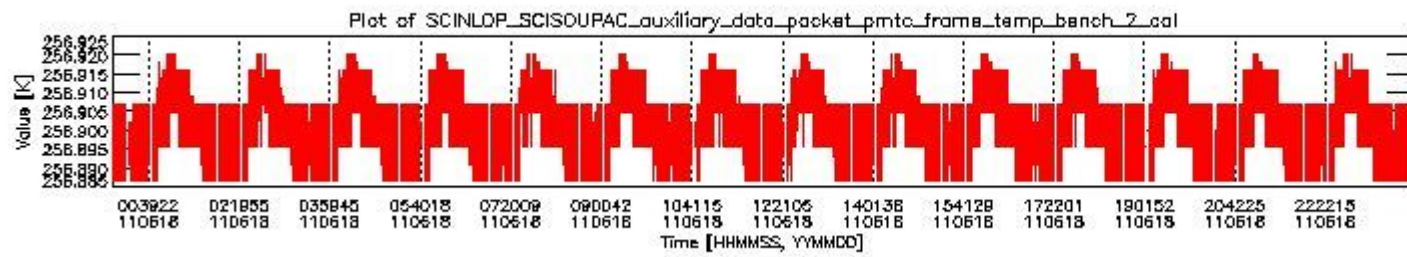
sciamachy_daily_report_level0_KSPT_L0_4504_N_20110618_1.PNG
