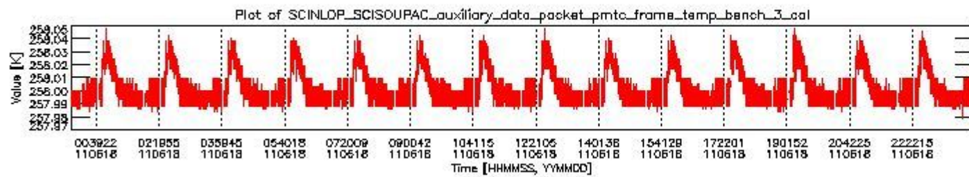
sciamachy_daily_report_level0_KSPT_L0_4504_N_20110618_2.PNG
