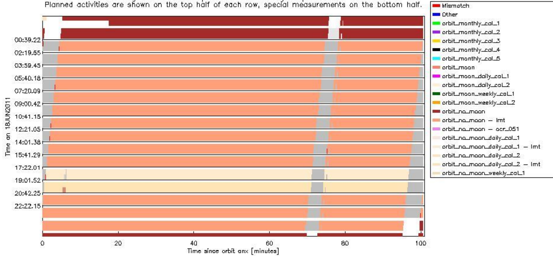
sciamachy_daily_report_level0_KSPT_L0_4504_N_20110618_6.PNG
