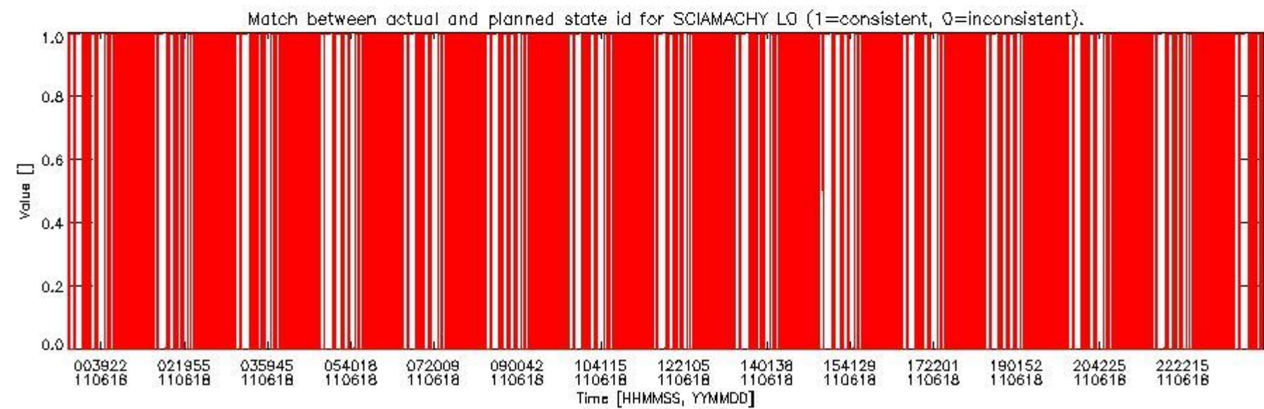
sciamachy_daily_report_level0_KSPT_L0_4504_N_20110618_5.PNG
