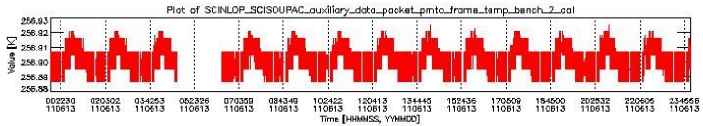
sciamachy_daily_report_level0_KSPT_L0_4504_N_20110613_1.PNG
