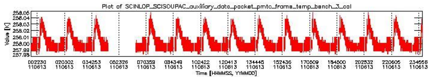
sciamachy_daily_report_level0_KSPT_L0_4504_N_20110613_2.PNG
