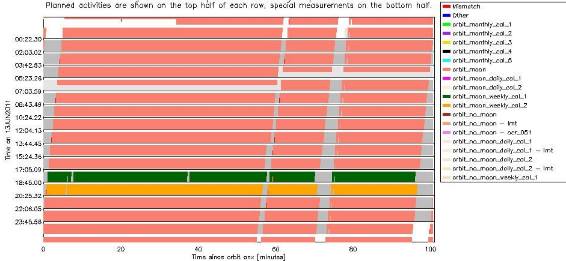
sciamachy_daily_report_level0_KSPT_L0_4504_N_20110613_6.PNG
