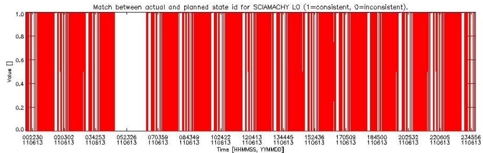
sciamachy_daily_report_level0_KSPT_L0_4504_N_20110613_5.PNG
