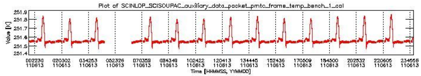
sciamachy_daily_report_level0_KSPT_L0_4504_N_20110613_0.PNG
