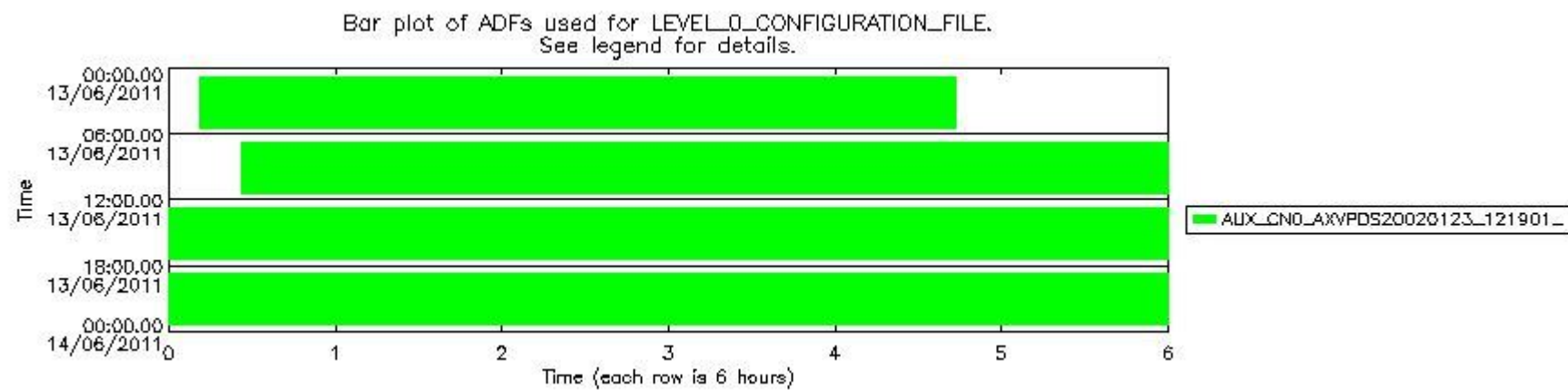
sciamachy_daily_report_level0_KSPT_L0_4504_N_20110613_7.PNG
