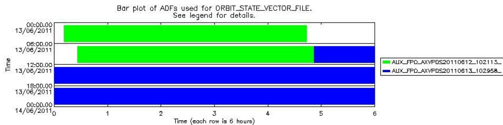
sciamachy_daily_report_level0_KSPT_L0_4504_N_20110613_8.PNG
