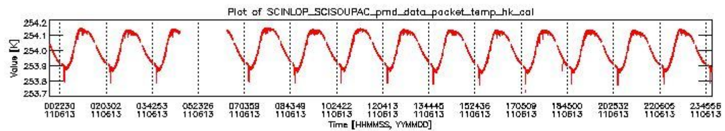
sciamachy_daily_report_level0_KSPT_L0_4504_N_20110613_3.PNG
