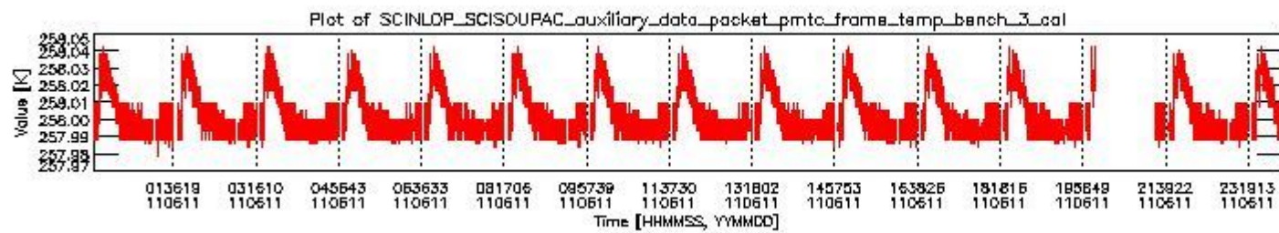
sciamachy_daily_report_level0_KSPT_L0_4504_N_20110611_2.PNG
