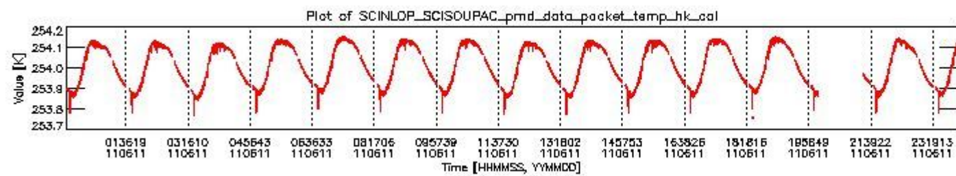
sciamachy_daily_report_level0_KSPT_L0_4504_N_20110611_3.PNG
