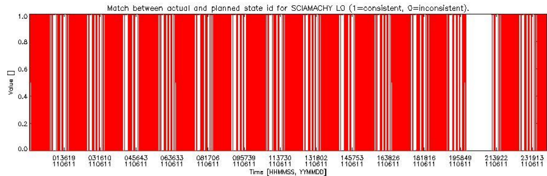
sciamachy_daily_report_level0_KSPT_L0_4504_N_20110611_5.PNG
