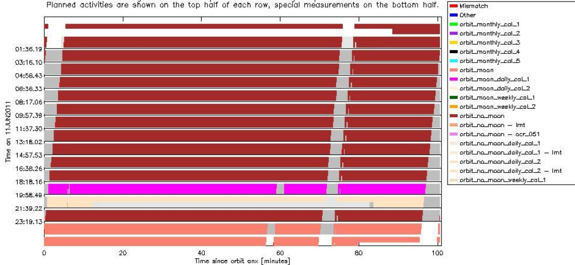
sciamachy_daily_report_level0_KSPT_L0_4504_N_20110611_6.PNG
