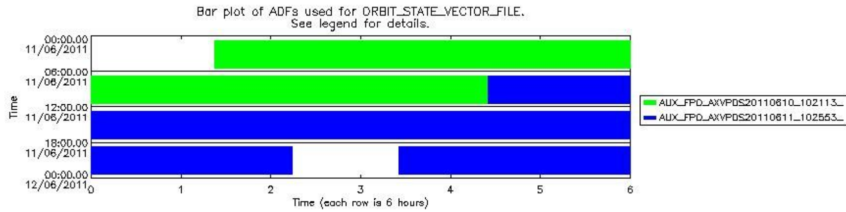
sciamachy_daily_report_level0_KSPT_L0_4504_N_20110611_8.PNG
