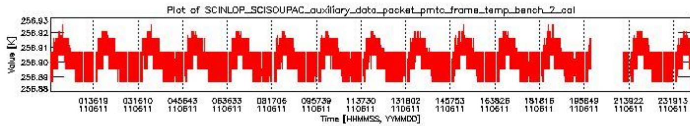
sciamachy_daily_report_level0_KSPT_L0_4504_N_20110611_1.PNG
