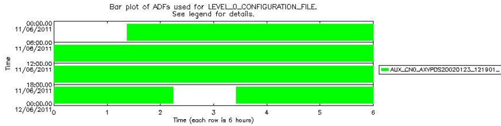
sciamachy_daily_report_level0_KSPT_L0_4504_N_20110611_7.PNG
