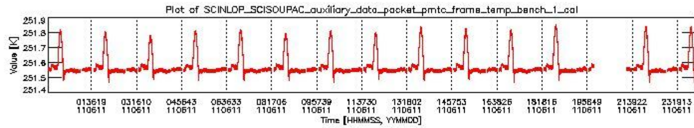
sciamachy_daily_report_level0_KSPT_L0_4504_N_20110611_0.PNG
