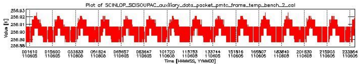
sciamachy_daily_report_level0_KSPT_L0_4504_N_20110605_1.PNG
