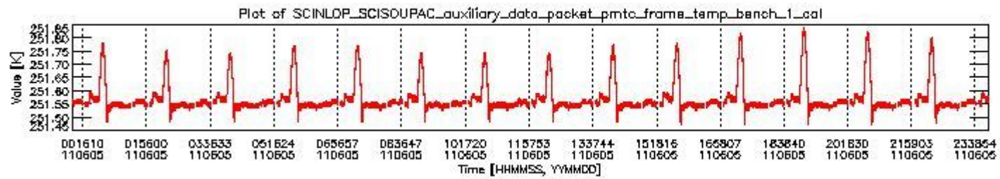
sciamachy_daily_report_level0_KSPT_L0_4504_N_20110605_0.PNG
