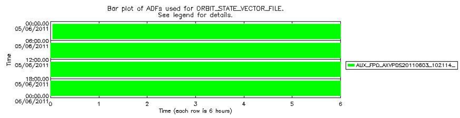
sciamachy_daily_report_level0_KSPT_L0_4504_N_20110605_8.PNG
