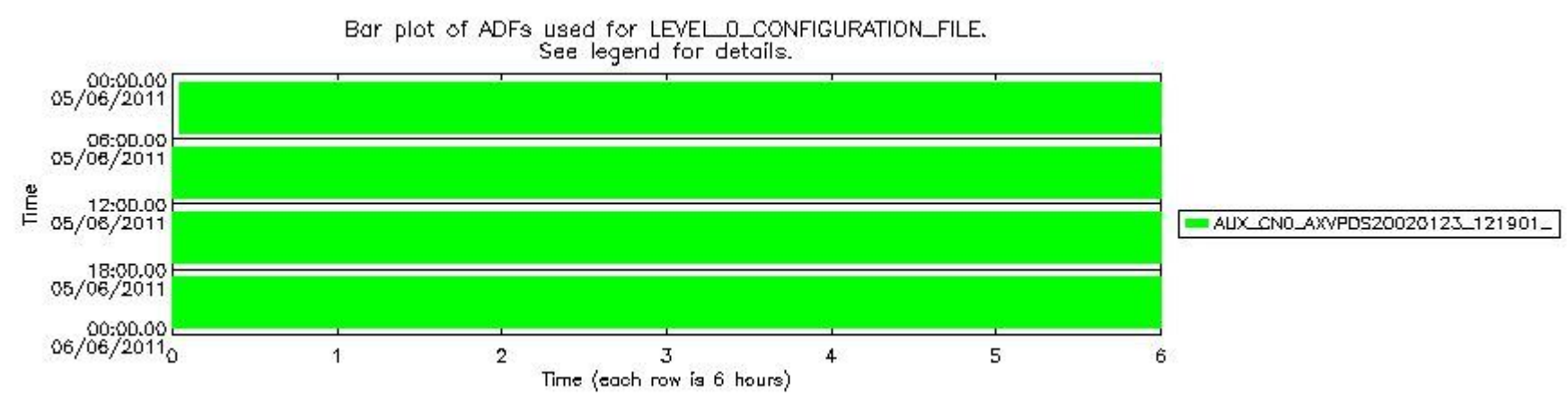
sciamachy_daily_report_level0_KSPT_L0_4504_N_20110605_7.PNG
