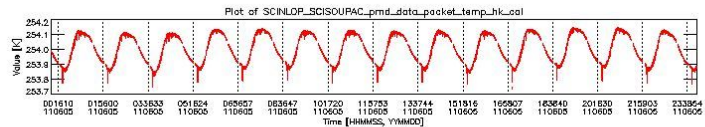
sciamachy_daily_report_level0_KSPT_L0_4504_N_20110605_3.PNG
