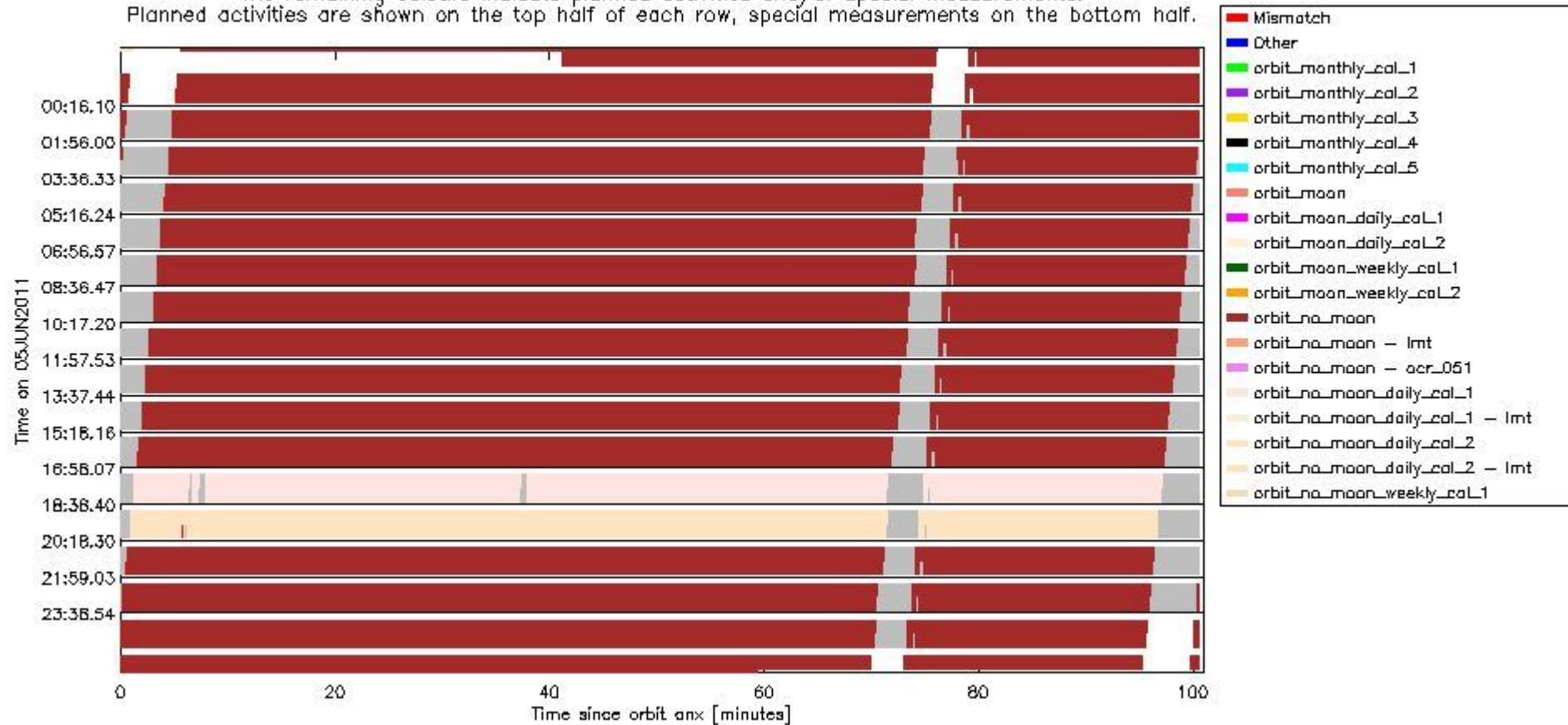
sciamachy_daily_report_level0_KSPT_L0_4504_N_20110605_6.PNG
