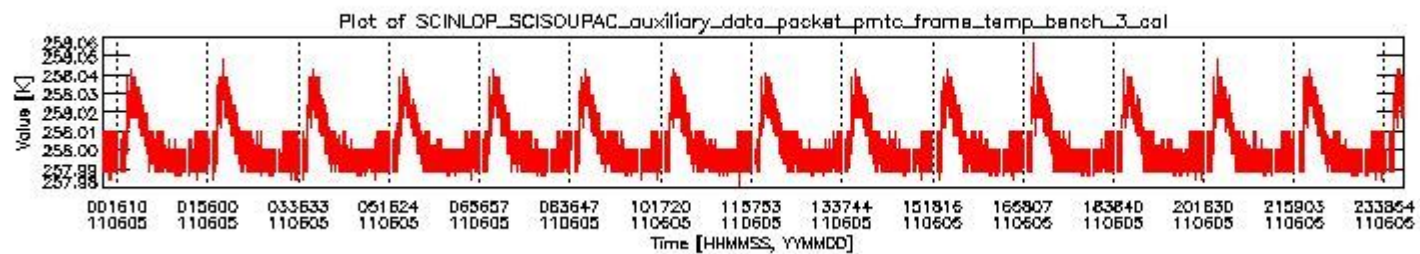
sciamachy_daily_report_level0_KSPT_L0_4504_N_20110605_2.PNG
