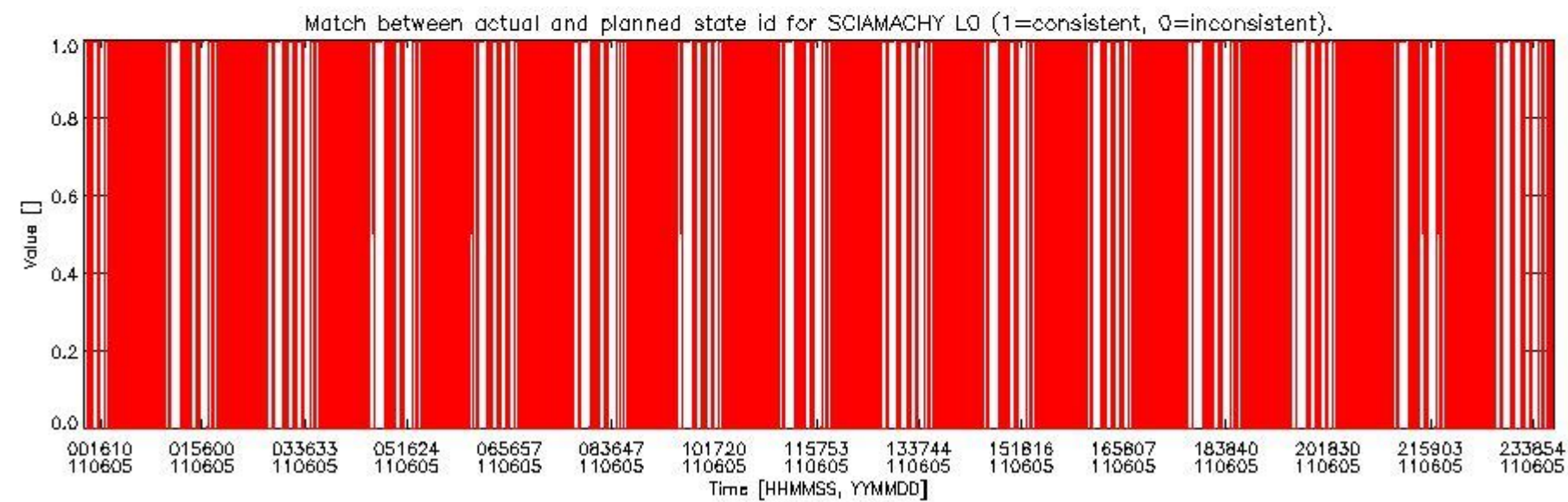
sciamachy_daily_report_level0_KSPT_L0_4504_N_20110605_5.PNG
