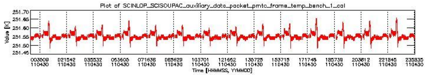
sciamachy_daily_report_level0_KSPT_L0_4504_N_20110430_0.PNG
