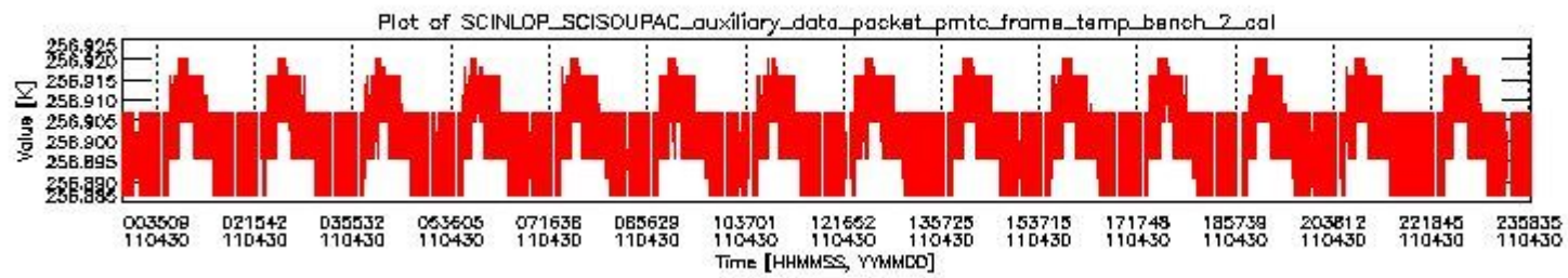
sciamachy_daily_report_level0_KSPT_L0_4504_N_20110430_1.PNG
