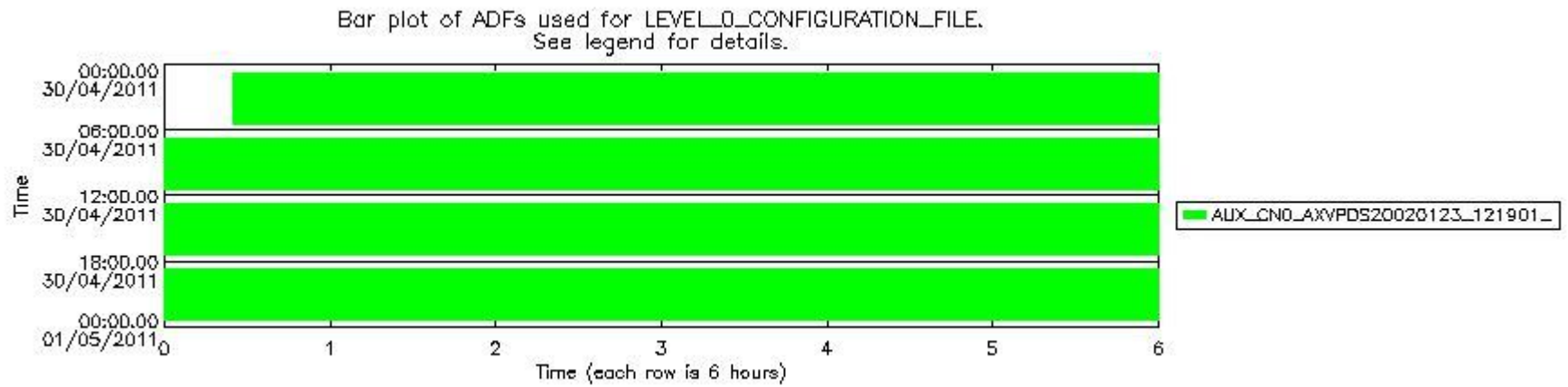
sciamachy_daily_report_level0_KSPT_L0_4504_N_20110430_6.PNG
