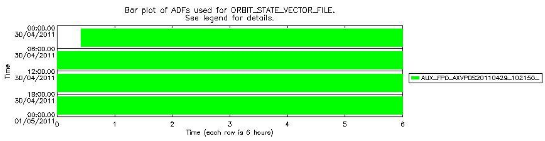
sciamachy_daily_report_level0_KSPT_L0_4504_N_20110430_7.PNG
