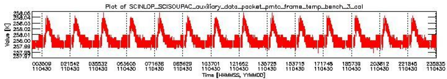
sciamachy_daily_report_level0_KSPT_L0_4504_N_20110430_2.PNG
