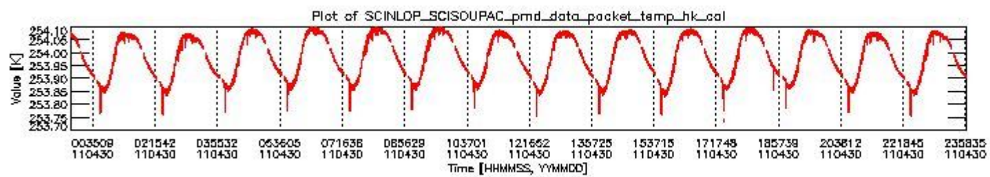
sciamachy_daily_report_level0_KSPT_L0_4504_N_20110430_3.PNG
